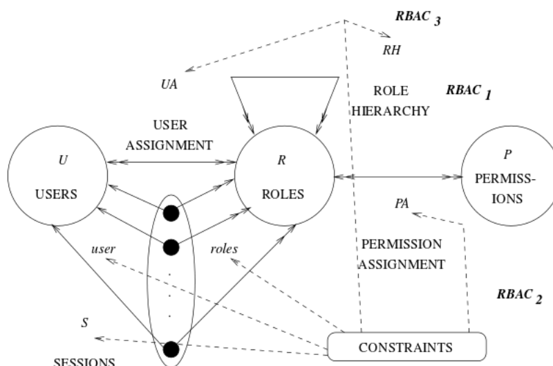
FIGURE 3.8 – Modèles RBAC [157].
