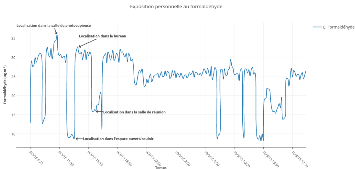
Figure 5.14 : Exposition personnelle au formaldéhyde
