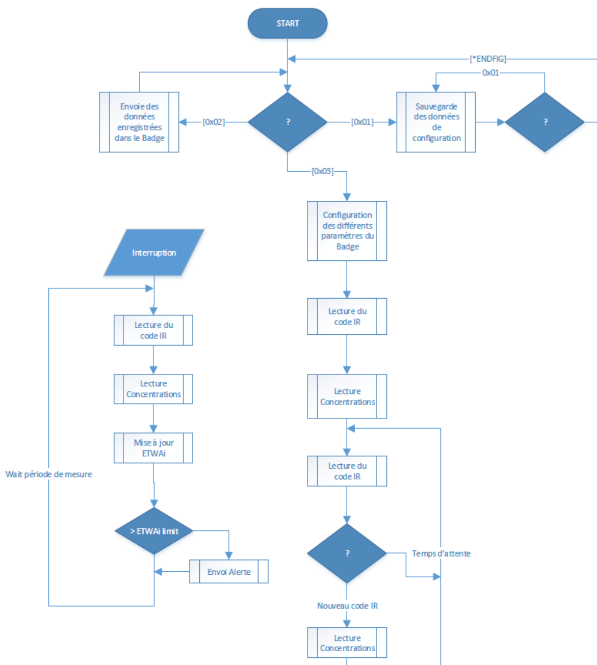
Figure 5.6 : Organigramme de fonctionnement du badge
