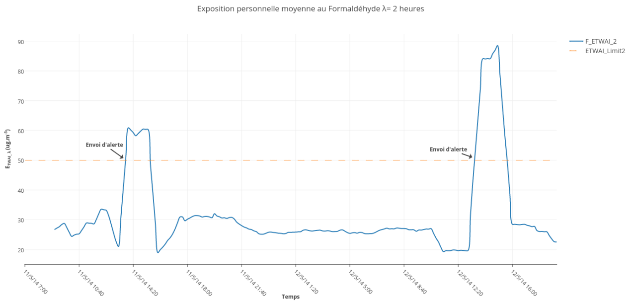
Figure 4.24 : E_{TWAi} au Formaldéhyde pour \lambda = 2 heures
