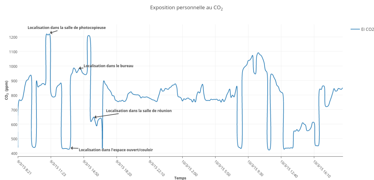
Figure 5.15 : Exposition personnelle au CO 2
