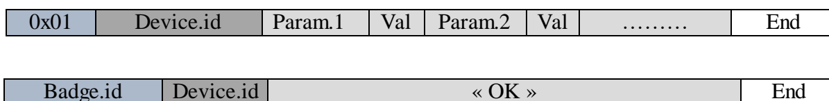
Figure 5.9 : Format de messages "Configuration.req" et "Configuration.resp"
