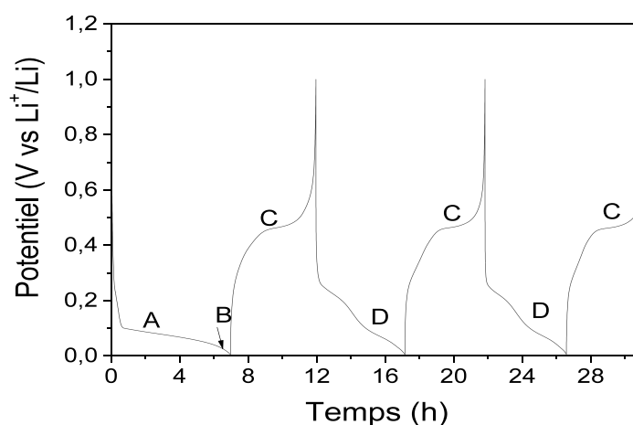
Figure I. 12 Evolution du potentiel lors des 3 premiers cycles d'une électrode de silicium.
