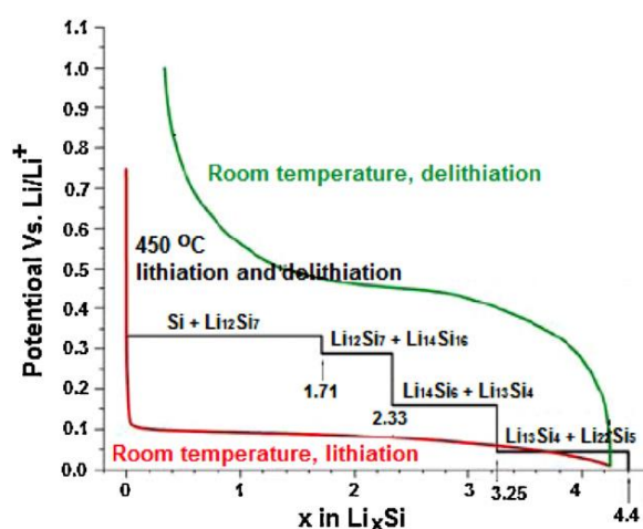
Figure I.11 Evolution du potentiel de l'électrode à base de Si lors du premier cycle de lithiation et delithiation du silicium cristallin à température ambiante (courbes rouge et verte) et à 450°C (courbe noire). [50]
