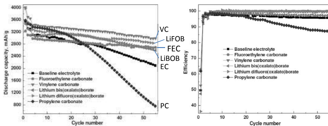
Figure I.20. Tenue au cyclage et efficacité coulombique de films mince de Si avec 1\text{MLiPF}_6 dans PC/EC/DMC ou EC/DMC/DEC avec 3 wt% FEC, 5 wt% VC, 5 wt% LiBOB ou 1 wt% LiFOB.[39]
