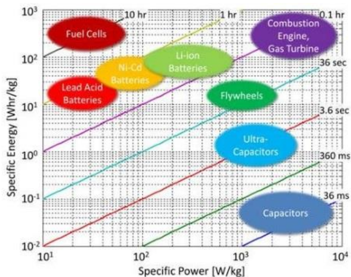
Figure 1.2 Diagramme de Ragone des différentes technologies de stockage électrochimique d'énergie, comparées au volant d'inertie et au moteur thermique. Les lignes diagonales représentent des temps de décharge constants.[4]
