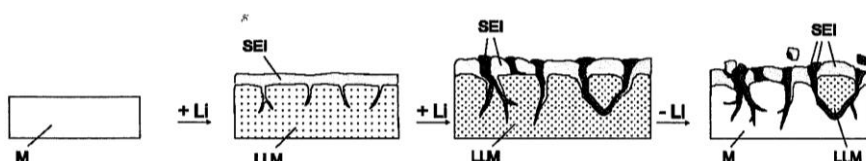
Figure I.17 Dégradation de l'électrode liée à la formation continue de SEI.[94]
