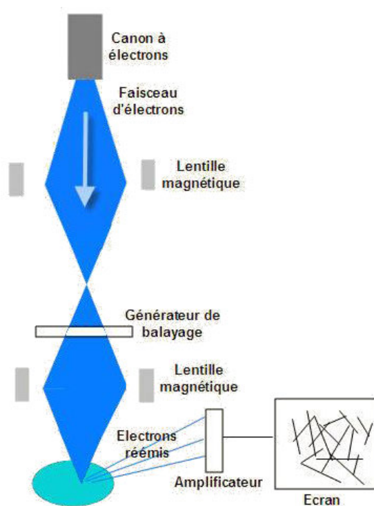
Figure II.11 Schéma d'un microscope électronique à balayage.
