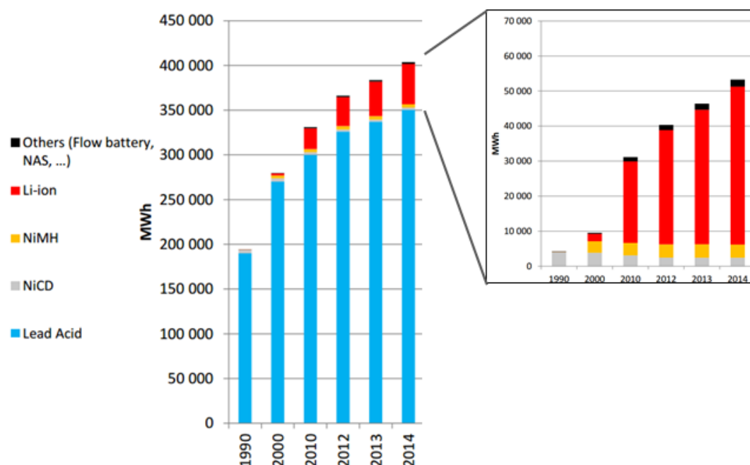
Figure I.4 Evolution en énergie du marché mondial des différentes technologies de batteries de 1990 à 2014.[6]
