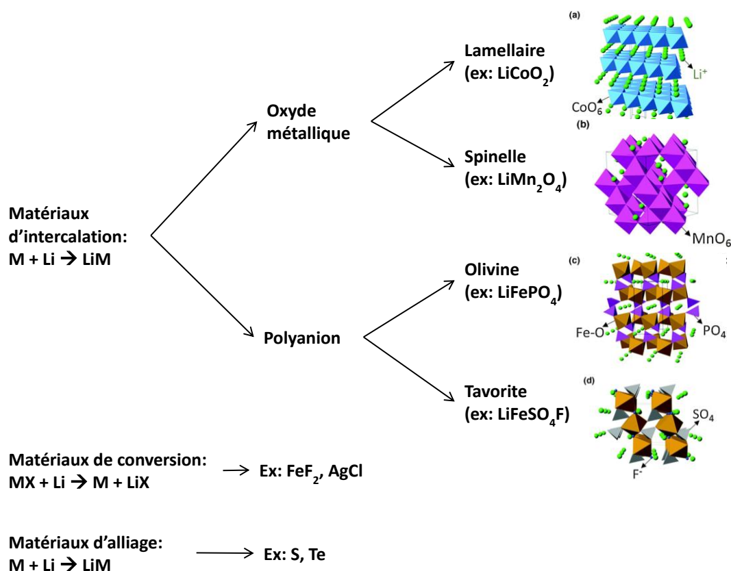
Figure I.7 Diagramme des différentes catégories de matériaux de cathode classés d'après leur mécanisme de lithiation et structure cristallographique [16].
