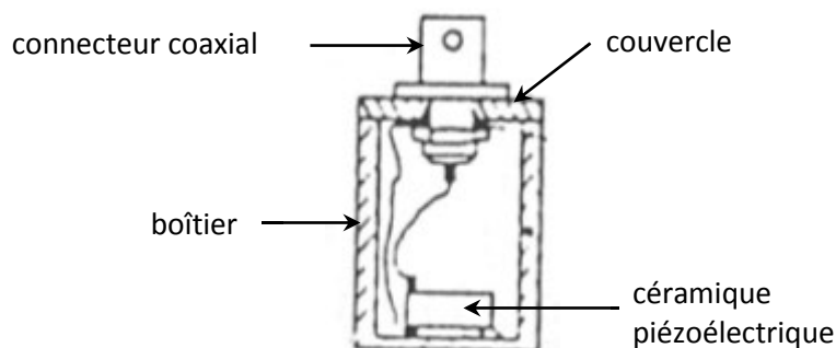
Figure II.3 Schéma d'un capteur piézoélectrique [9].
