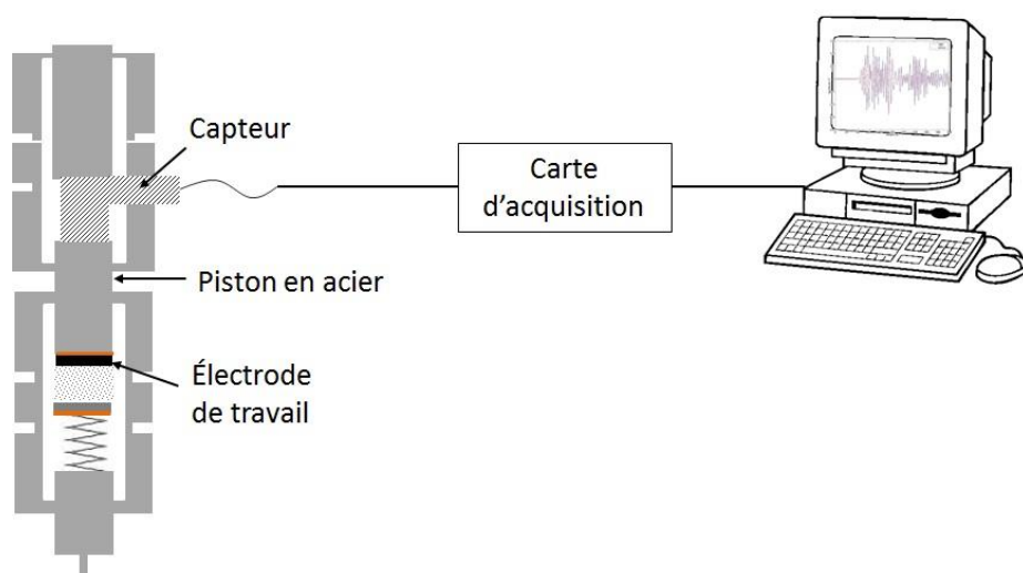
Figure II.7 Schéma du montage de mesure d'émission acoustique.
