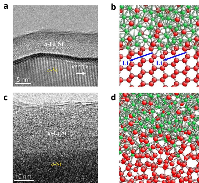
Figure I.13. Mécanisme de lithiation cœur-coquille du silicium cristallin (a et b) et amorphe (c et d). (a et c) Images MET haute résolution de l'interface entre c-Si et a-Li x Si. (b et d) Schémas représentatifs de la structure atomique à l'interface réalisés par simulation de dynamique moléculaire.[54]
