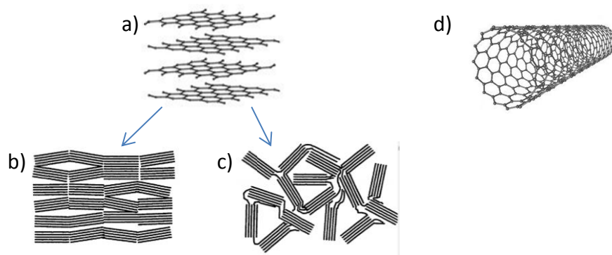
Figure I.8 Structures cristallines du carbone : a) graphite sous forme b) ordonnée et c) désordonnée, et d) nanotube de carbone.
