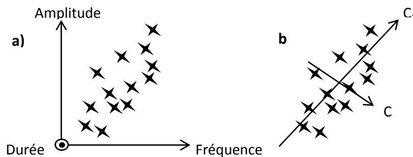
Figure II.5 Dispersion des données a) dans l'espace des paramètres et b) dans celui des composantes principales.
