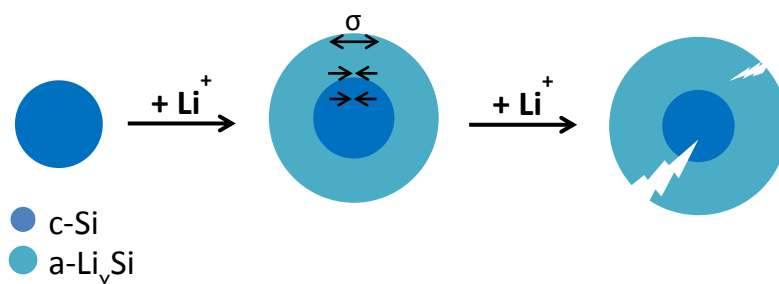
Figure I.14 Répartition des contraintes dans une particule sphérique au cours de la lithiation conduisant à la fracturation.
