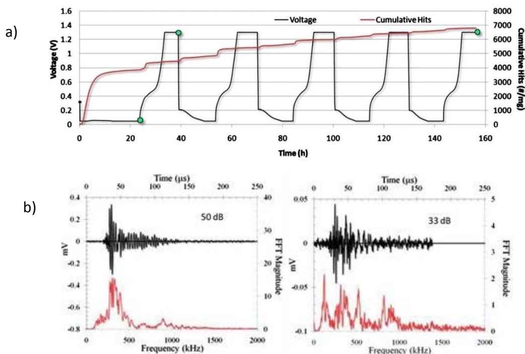
Figure I.21 a) Evolution de l'activité acoustique au cours du cyclage [204] et b) formes d'onde et spectres de puissance de deux signaux associées à la fracture du silicium [205].
