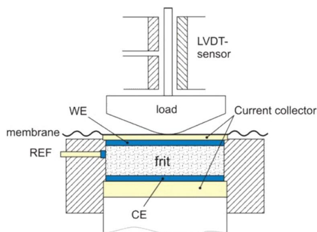
Figure II.8 Schéma de la cellule de dilatométrie électrochimique.
