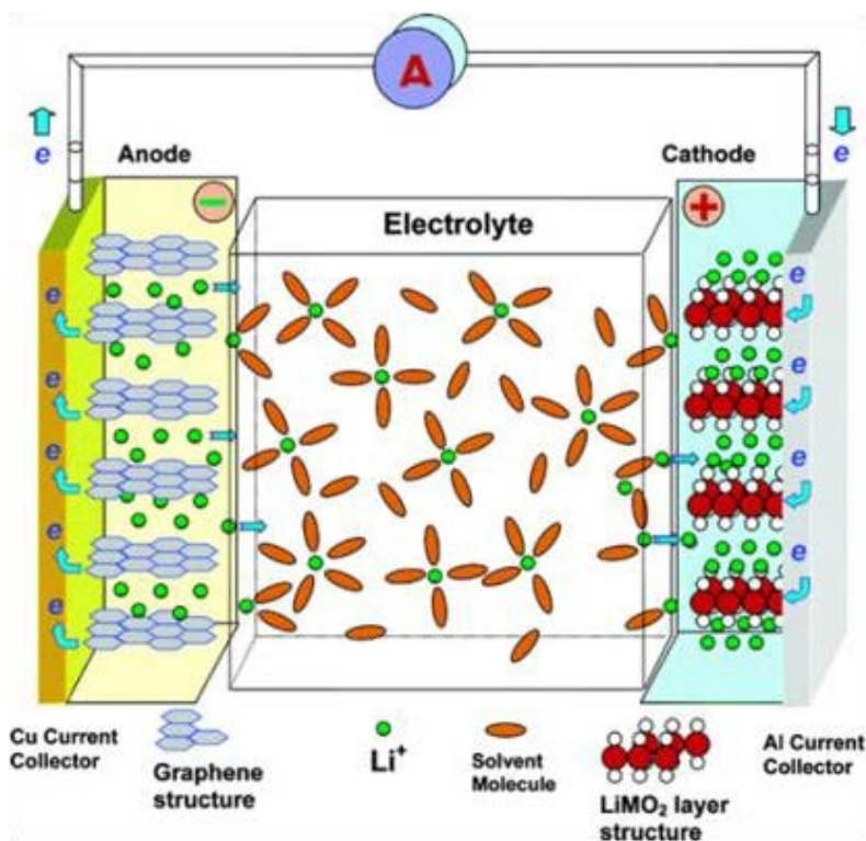
Figure I.5 Schéma du fonctionnement d'une batterie Li-ion lors de la décharge, avec du graphite comme matériau d'électrode négative et LiMO 2 comme matériau d'électrode positive (avec M=Co, Mn,...).
