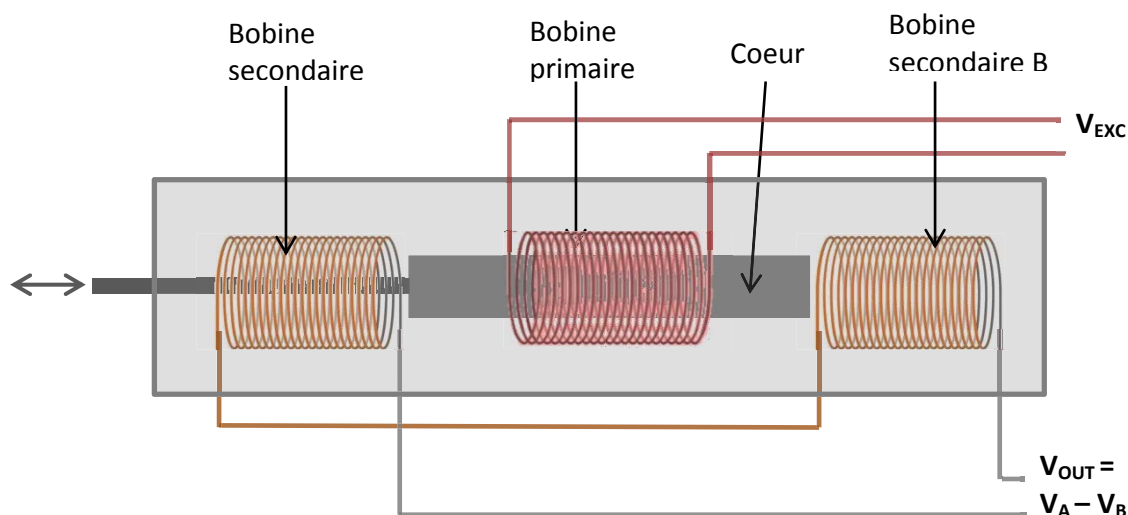
Figure II.8 Schéma de fonctionnement d'un capteur LVDT.
