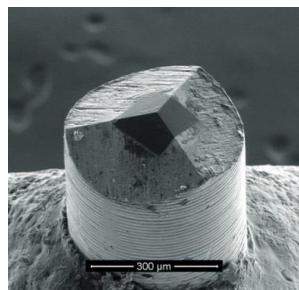
Figure II.9 Micrographe MEB d'une pointe en diamant de type Berkovich.
