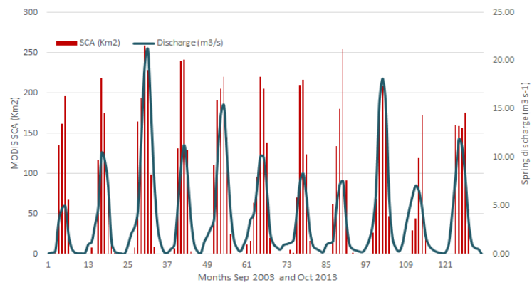
Figure. 1.3 (a) La source Afqa (altitude 1113 m) dans le bassin de la rivière Ibrahim en hiver quand le débit est encore minime. L'image a été prise le 24 Février 2015 (avec l'aimable autorisation de l'auteur); et (b) la corrélation entre MODIS SCA et le débit d'Afqa pour les années 2003 à 2013.
