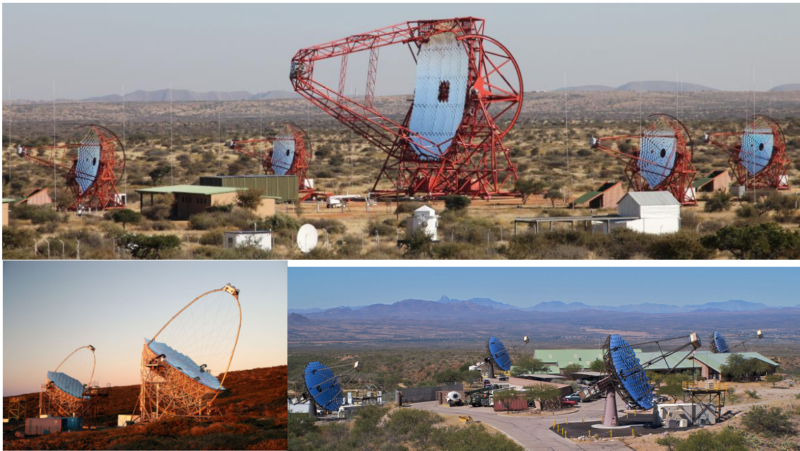
Figure 0.2: En haut: l'expérience H.E.S.S. située dans l'hémisphère sud en Namibie est composée de cinq télescopes Cherenkov. En bas à gauche: l'expérience MAGIC installé à La Palma. En bas à droite: l'expérience VERITAS, composée de quatre télescopes Cherenkov, est située dans l'hémisphère Nord, en Arizona.
