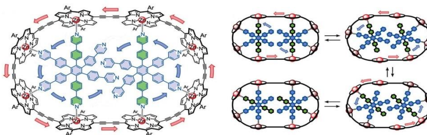
Fig. 15 Supramolecular caterpillar.
