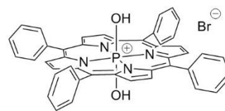
16b, [P(TPP)(OH) 2 ] + Br -
