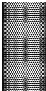
Fig 6.1 – Maillage linéaire d'une éprouvette cylindrique de diamètre 16 cm et de hauteur 32 cm (11217 noeuds et 54983 tétraèdres).
