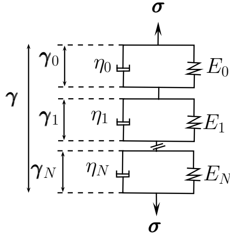
Fig 4.13 – Forme différentielle de la partie non vieillissante du terme viscoélastique \boldsymbol{\varepsilon}^{ve} de la théorie MPS.
