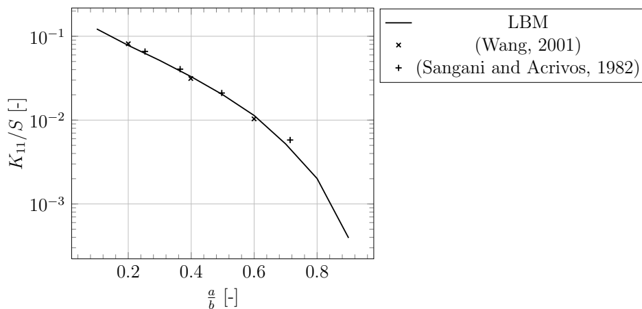
Fig 2.21 – Perméabilité normalisée K_{11}/S d'un écoulement suivant x à travers un réseau de cylindres à section circulaire. Comparaison de la perméabilité calculée par la LBM et les résultats de (Wang, 2001) et de (Sangani and Acrivos, 1982) dans le cas de l'arrangement carré.
