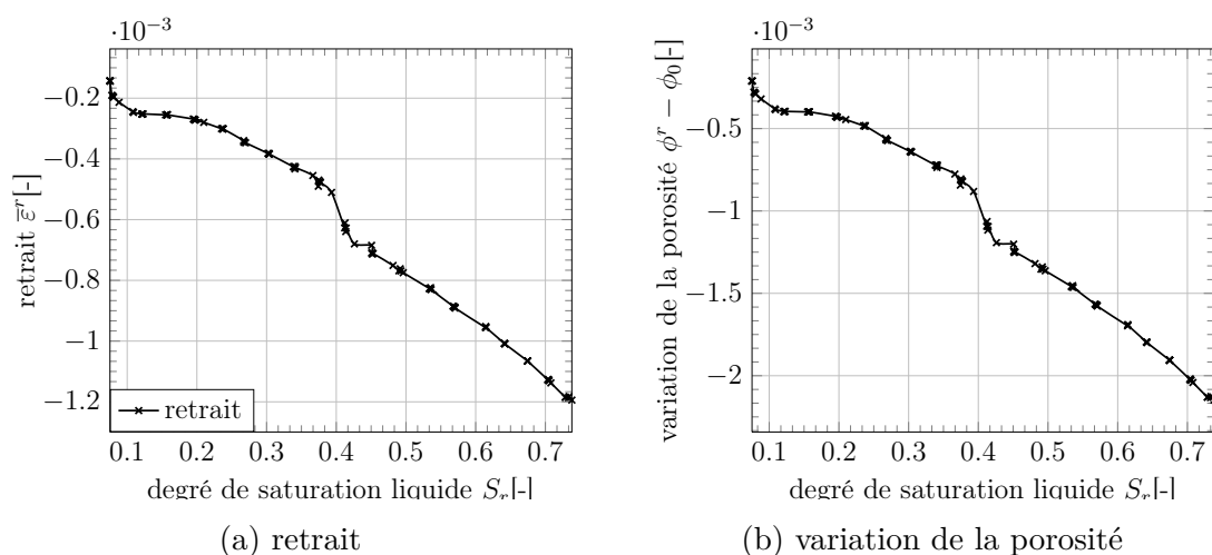
Fig 5.18 – Variation de volume induite par le séchage d'une microstructure cubique centrée.
