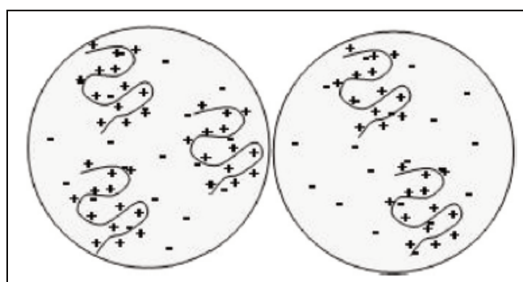
Figure I-0-16. Modèle de flocculation par neutralisation de charge. En surface apparaît des patches électrostatiques positifs et des surfaces négatives où il n'y a pas de polyélectrolytes adsorbés.
