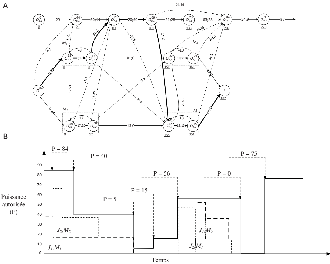
Figure 11 Nouveau graphe après permutation (A) et ordonnancement associé (B)
