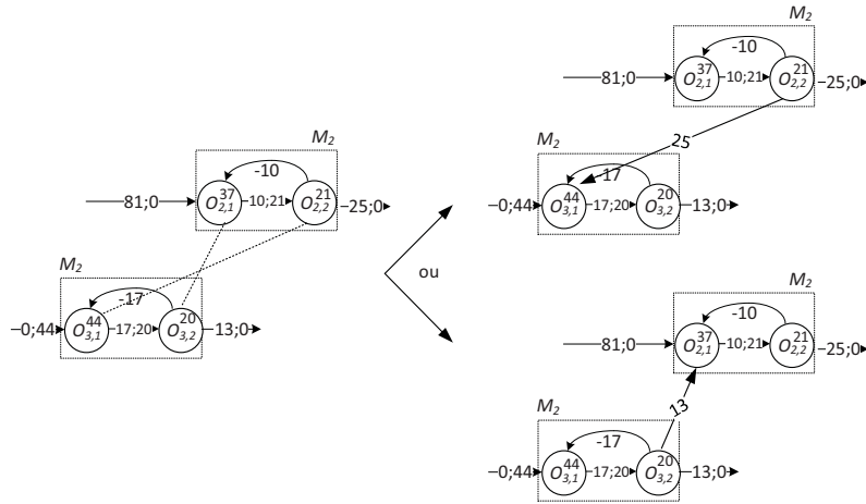
Figure 9 Précédences possibles entre deux sous-opérations (disjonctions)
