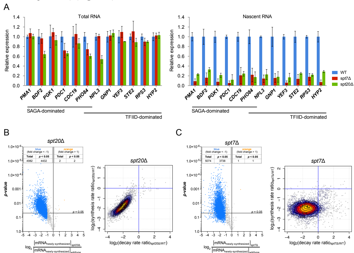
Figure 2 - SAGA est nécessaire pour l'activité de l'ARN polymérase II sur l'ensemble des gènes. (A) Les ARNm totaux et nouvellement synthétisés ont été extraits de souches de levure sauvages (WT), spt7Δ , and spt20Δ et quantifiés par RT-qPCR. (B et C) (Panels de gauche) Volcano plot montrant l'amplitude des modifications des taux d'ARNm nouvellement synthétisés et leur significativité statistique (p-value). Les amplitudes de modification (FC) sont calculées comme le Log 2 du rapport entre le taux d'ARNm de chaque gène après normalisation par le signal S. pombe dans la souche spt20Δ (B) ou la souche spt7Δ (C) et le taux du même ARNm dans la souche sauvage S. cerevisiae . (Panels de droite) Profils cDTA pour les souches spt20Δ (B) et spt7Δ (C). Pour tous les gènes analysés, les modifications de taux de synthèse sont indiquées en fonction des modifications des taux de dégradation. Les taux de modifications sont calculés comme le Log 2 des rapports entre mutant et sauvage.
