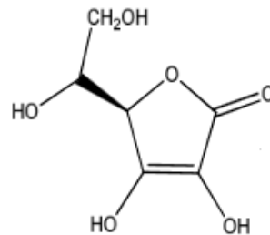
Figure 23. Structure chimique de l'acide L-ascorbique 88 .
