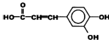
Figure 25. Structure chimique de l'acide caféique 94 .
