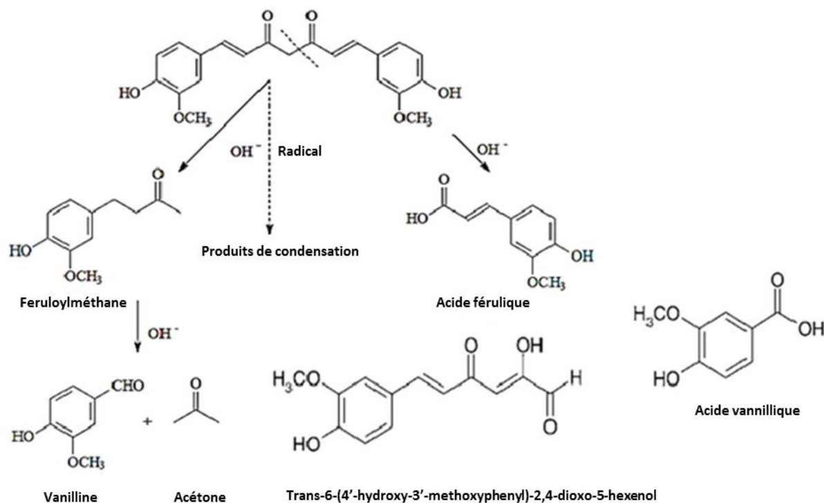
Figure 8. Les différents produits de dégradation et d'autoxydation de la curcumine dans un milieu alcalin 58 .
