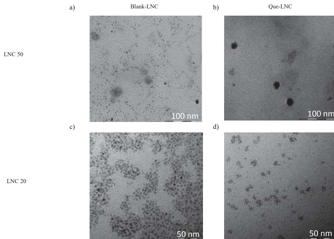
Fig. 2: TEM images for a) blank-LNC 50, b) que-LNC 50, c) blank-LNC 20 and d) que-LNC 20.
