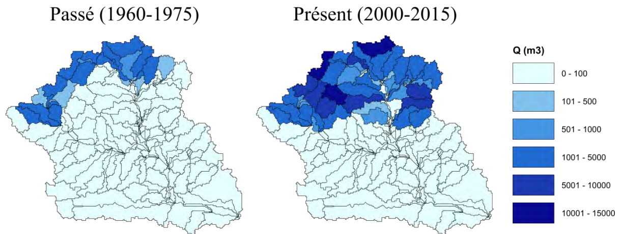
Figure 43: Ruissellement moyen par plan sur la période de mousson (JAS) pour la période passée (1960-1975) et la période présente (2000-2015)
