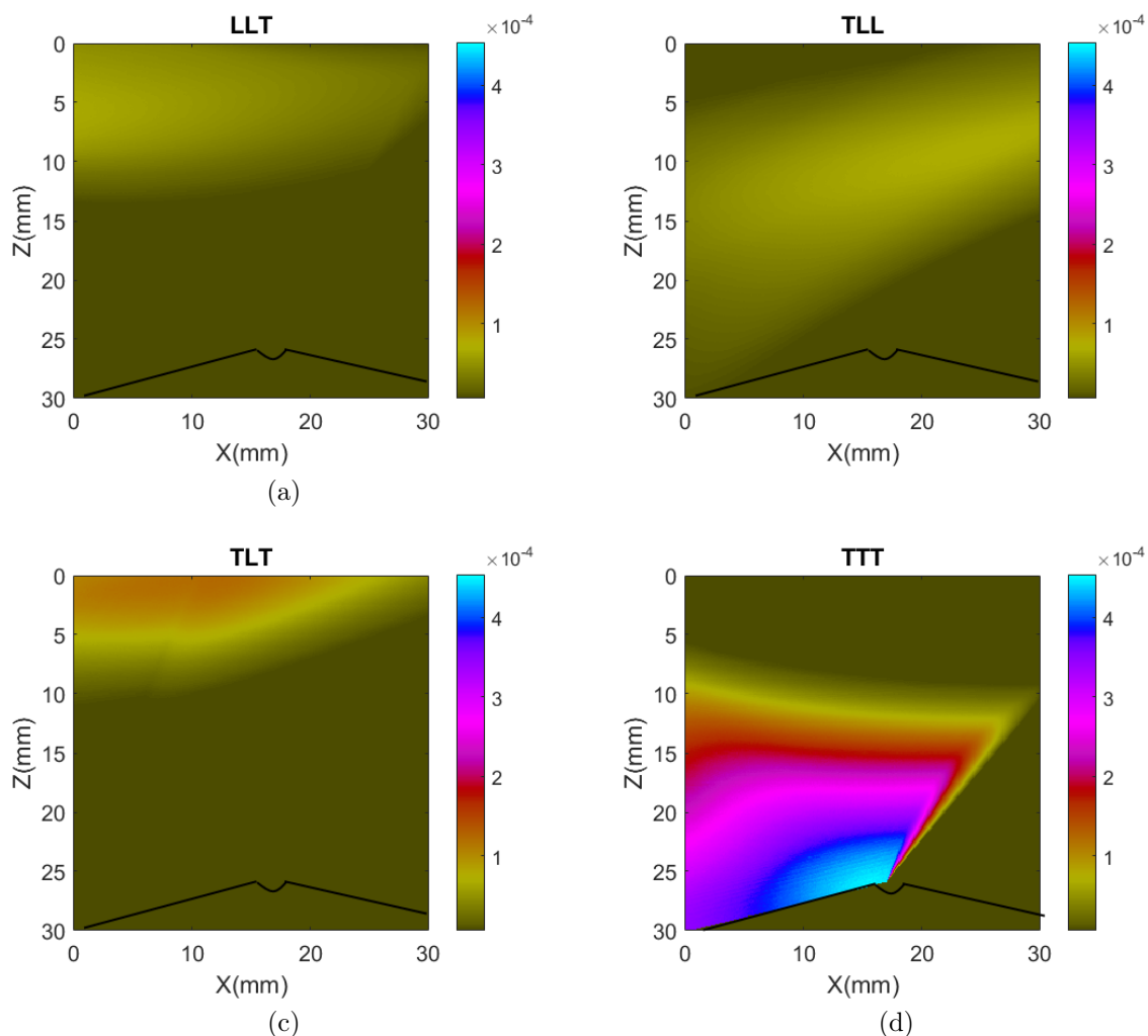
Fig 6.15 – Cartographies SEE des modes LLT, TLL, TLT et TTT
