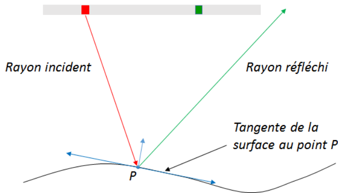
Fig A.5 – Hauteur d'eau suffisante pour une superposition des cônes de divergence mais trajet non spéculaire pour un couple d'éléments
