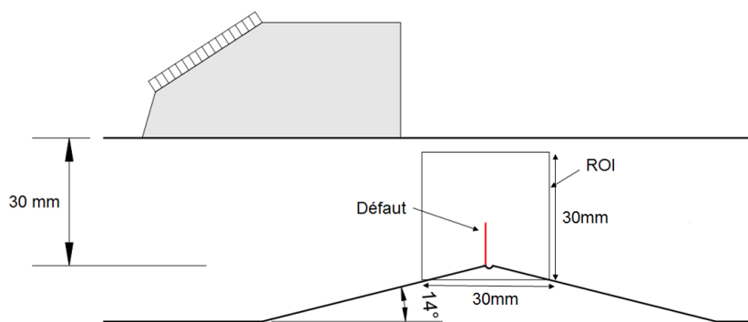
Fig 4.1 – Configuration d’inspection expérimentale
