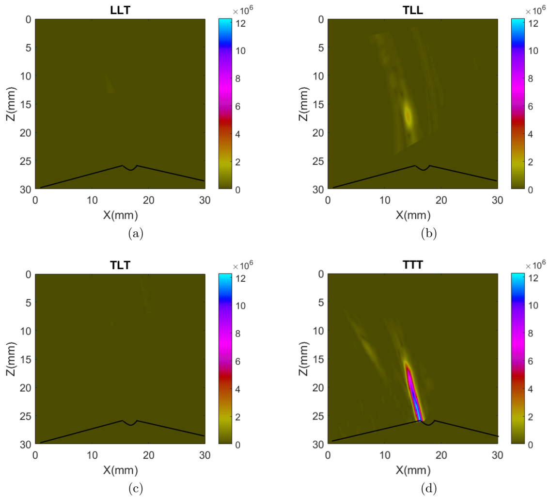
Fig 6.19 – Images TFM expérimentales des modes LLT, TLT et TTT
