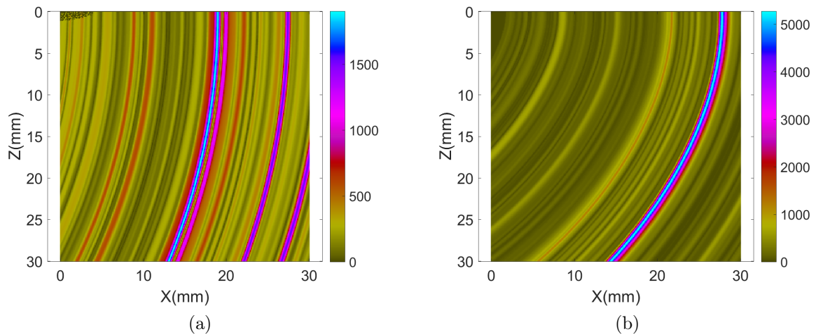
Fig 2.11 – Image TFM réalisée pour le couple d’élément (a)1-1, (b) 64-64
