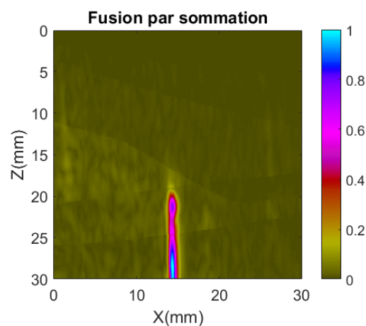
Fig 6.35 – Fusion par sommation des modes sélectionnés
