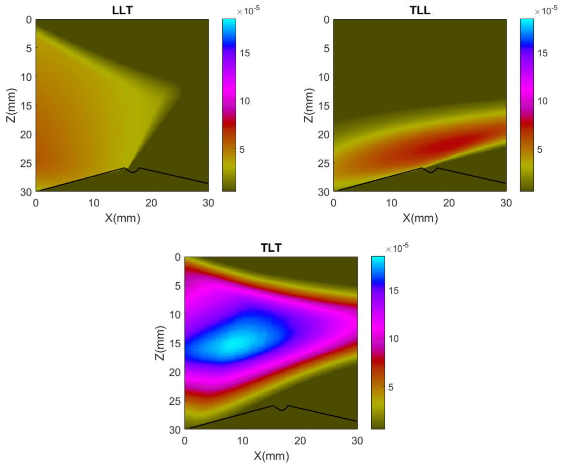
Fig 3.15 – Les trois modes prédits par la sélection des modes basée sur la maximisation du nombre de modes
