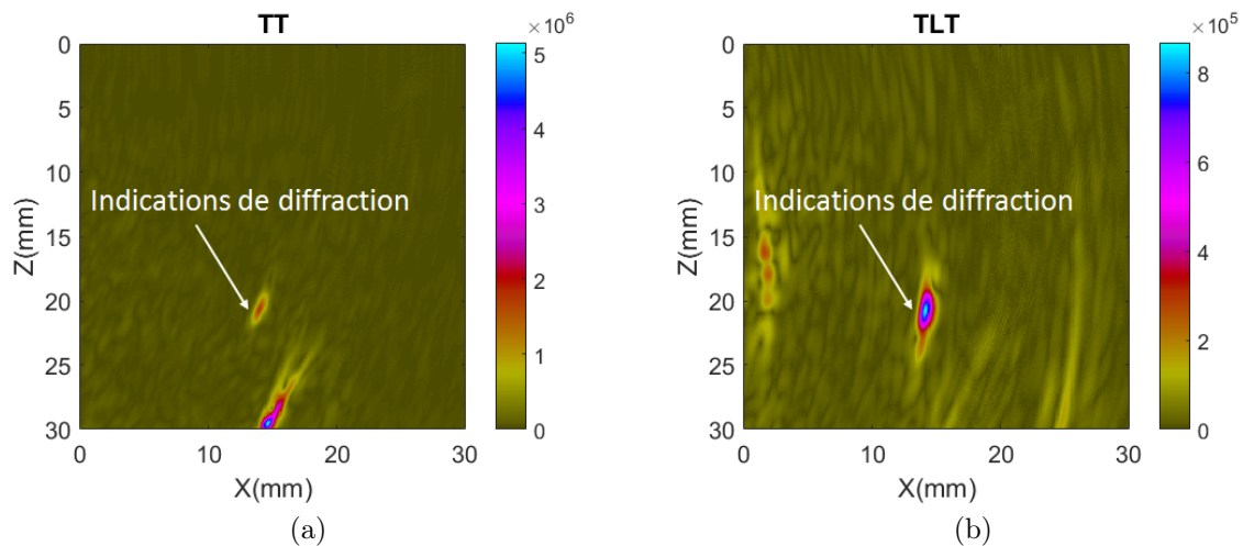
Fig 2.13 – Indication de diffraction reconstruite suivant les modes (a) TT et (b) TLT
