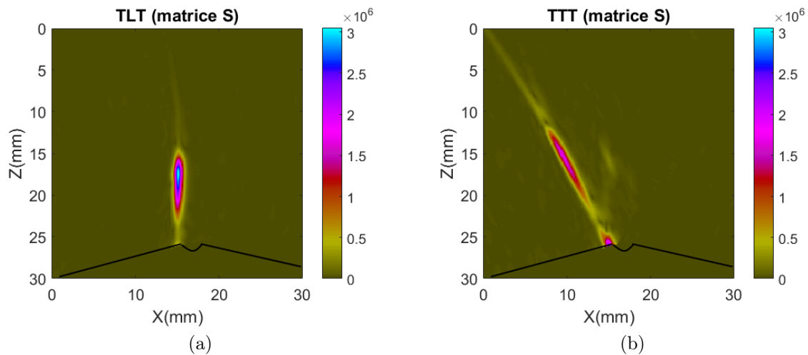
Fig 4.18 – Images TFM des modes TLT et TTT
