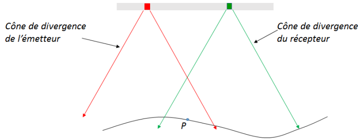
Fig A.4 – Hauteur d'eau suffisante pour une superposition des cônes de divergence pour un couple d'éléments
