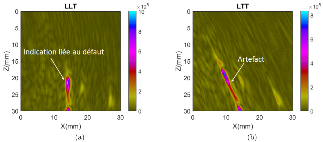
Fig C.1 – Reconstructions TFM suivant les modes (a) LLT et (b) LTT
