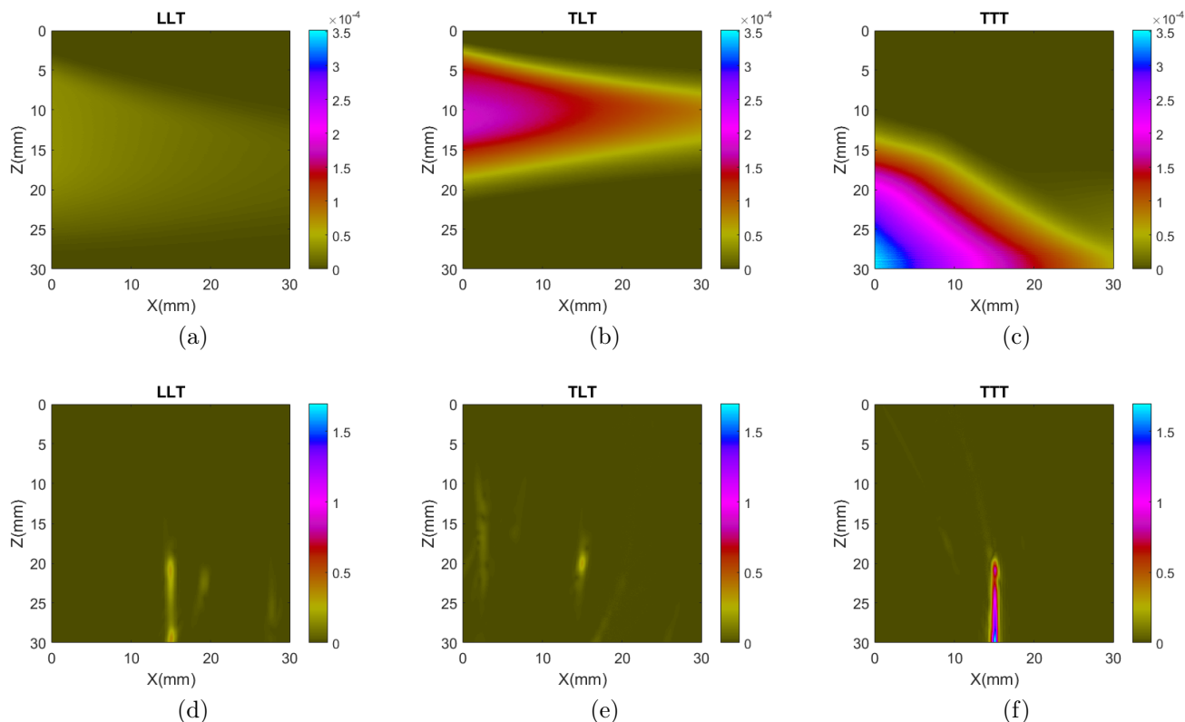
Fig 6.30 – Cartographies SEE des modes (a) LLT, (b) TLT et (c) TTT, Images TFM simulées des modes (d) LLT, (e) TLT et (f) TTT
