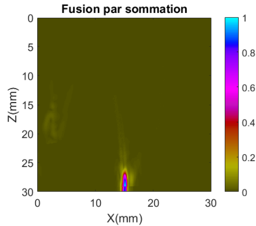
Fig 6.39 – Fusion par sommation des modes sélectionnés
