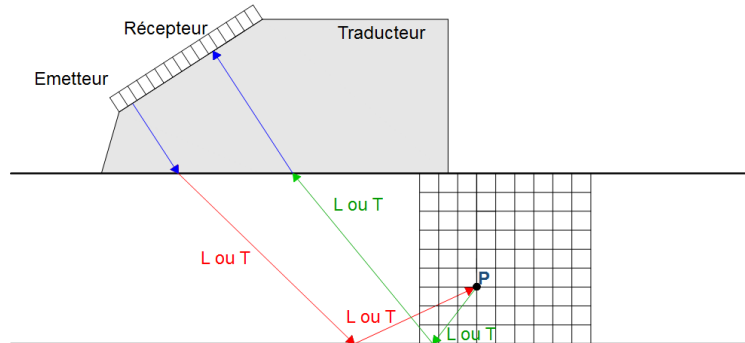
Fig 2.4 – Modes indirects. En rouge, le trajet à l'émission, en vert le trajet à la réception
