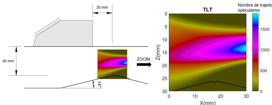
Fig 3.2 – Cartographie du compteur de réflexions pour un défaut plan vertical
