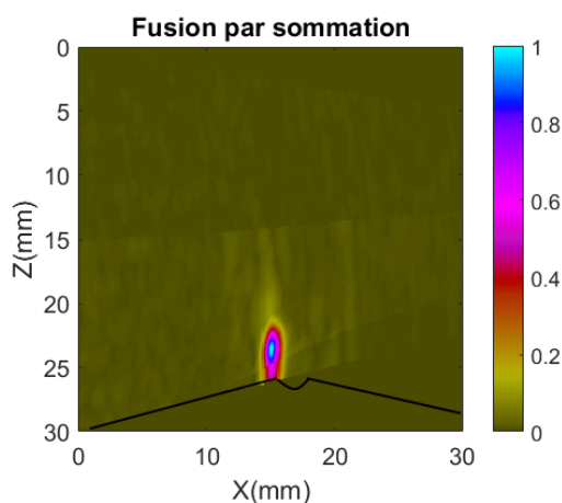
Fig 6.11 – Fusion par sommation des modes sélectionnés
