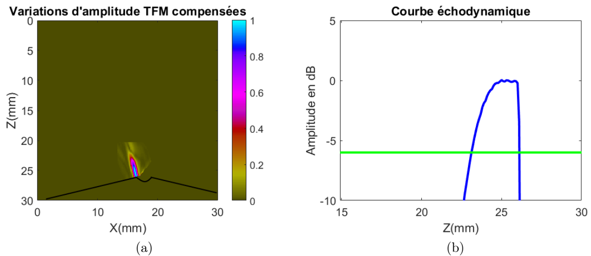
Fig 6.27 – (a) Compensation des variations d'amplitude (b) Courbe échodynamique
