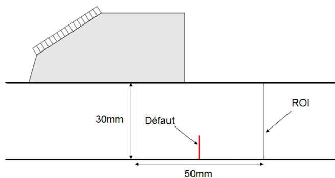
Fig 4.2 – Configuration d’inspection simulée
