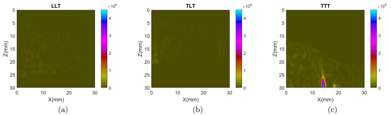
Fig 6.41 – Images TFM expérimentales des modes LLT, TLT et TTT
