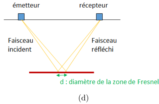
Fig 5.12 – Zone de Fresnel pour un couple d’éléments
