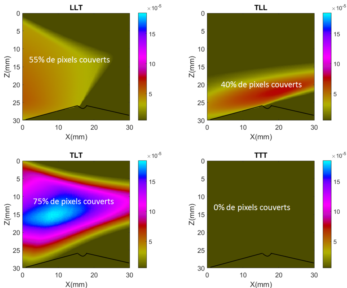
Fig 3.12 – Proportion de pixels couverts par modes pour un défaut vertical
