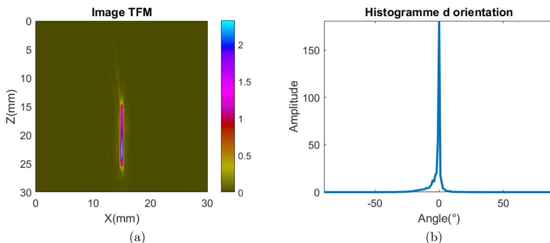
Fig 5.1 – (a) Image TFM reconstruite suivant le mode TTT et (b) histogramme d'orientation associée à l'image
