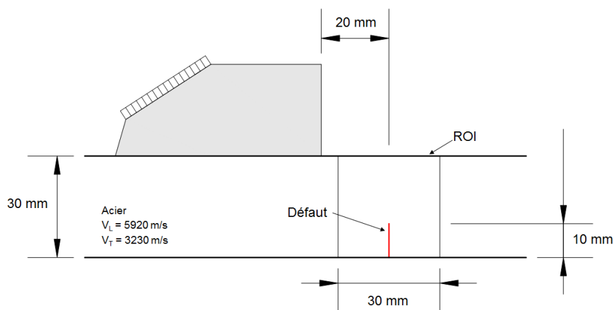
Fig 6.28 – Configuration d'inspection : pièce plane, défaut vertical de 10mm de hauteur
