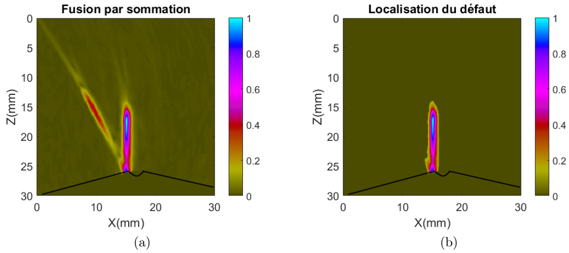
Fig 4.22 – (a) Image issue de la fusion par sommation des modes TLL, TLT et TTT (b) Image obtenue après l'application de l'algorithme de croissance de région
