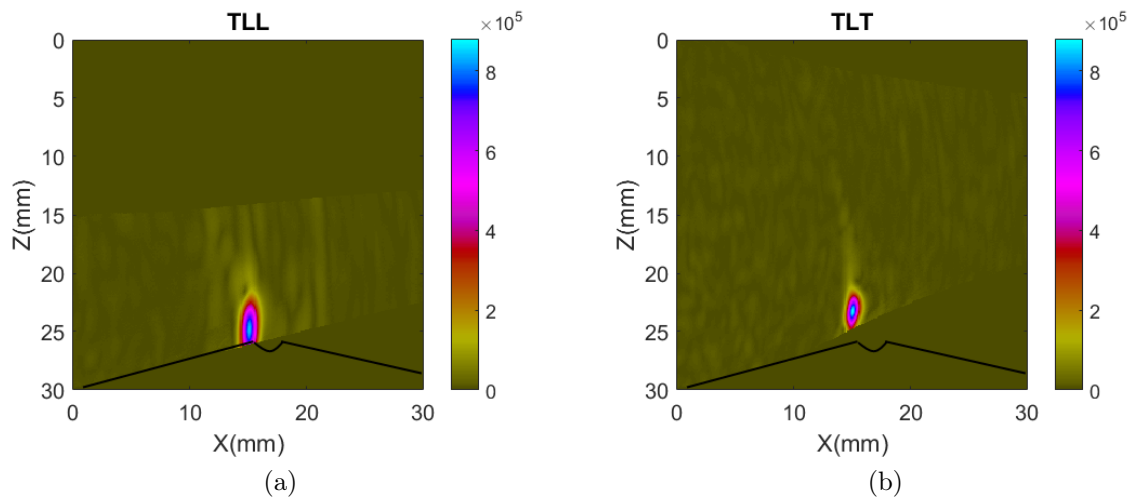
Fig 6.10 – Images TFM expérimentales des modes TLL et TLT
