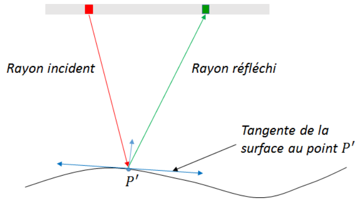
Fig A.6 – Hauteur d'eau suffisante pour une superposition des cônes de divergence et trajet spéculaire pour un couple d'éléments
