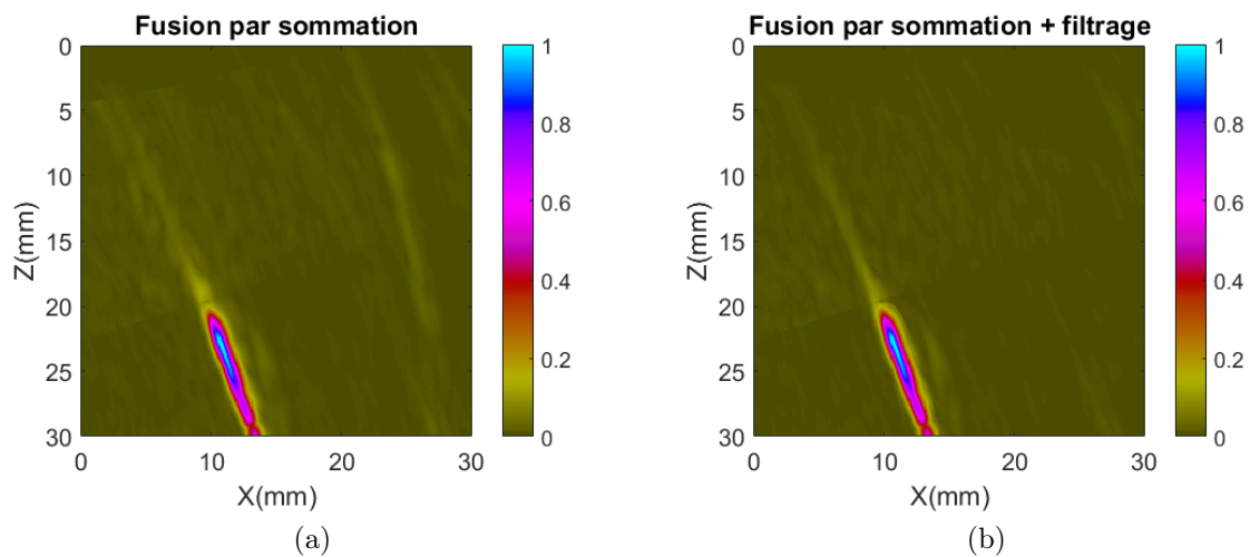
Fig 6.50 – (a) Fusion par sommation des modes sélectionnés (b) Image filtrée de ses artefacts
