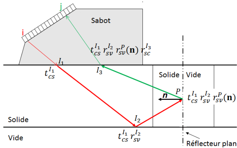
Fig 3.4 – Variation de l'amplitude d'une onde plane entre un couple émetteur et récepteur
