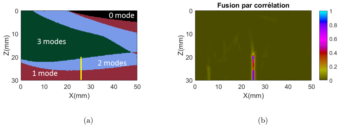
Fig 4.12 – (a) Cartographie de la distribution du nombre de modes fusionnés par pixel, (b) Fusion par corrélation des modes LLT, TLT et TTT
