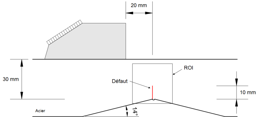
Fig 2.19 – Configuration d'inspection
