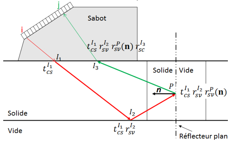
Fig 3.4 – Variation de l'amplitude d'une onde plane entre un couple émetteur et récepteur
