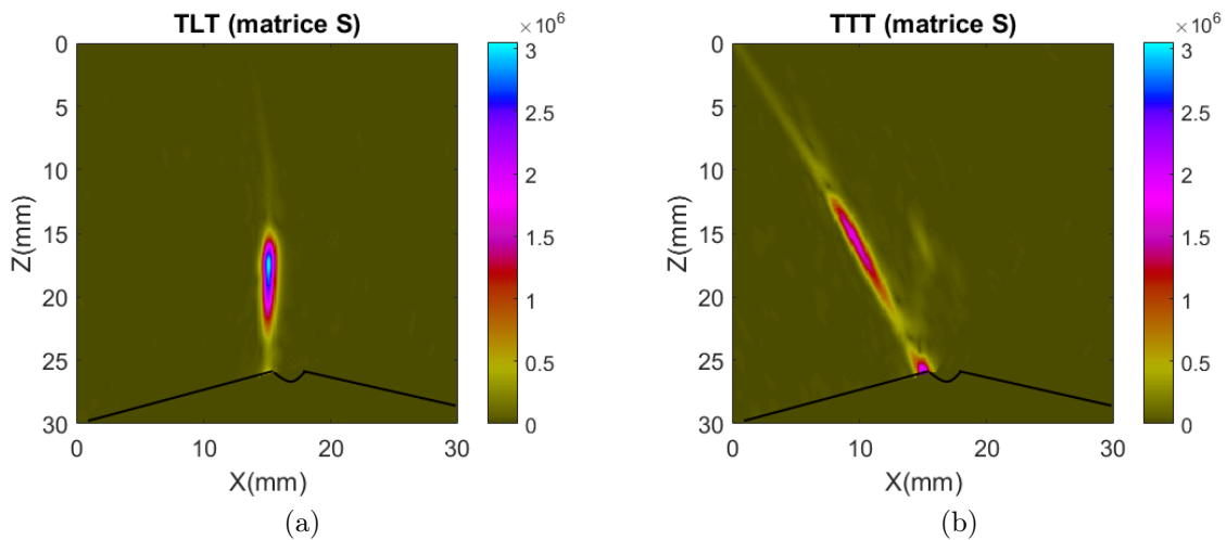
Fig 4.18 – Images TFM des modes TLT et TTT
