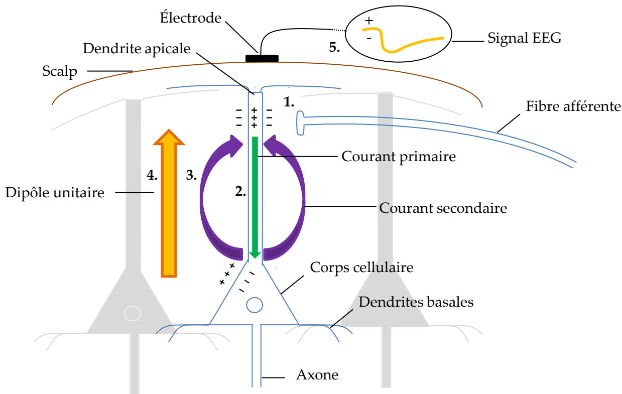
Figure 7 - Principe de l'EEG.
