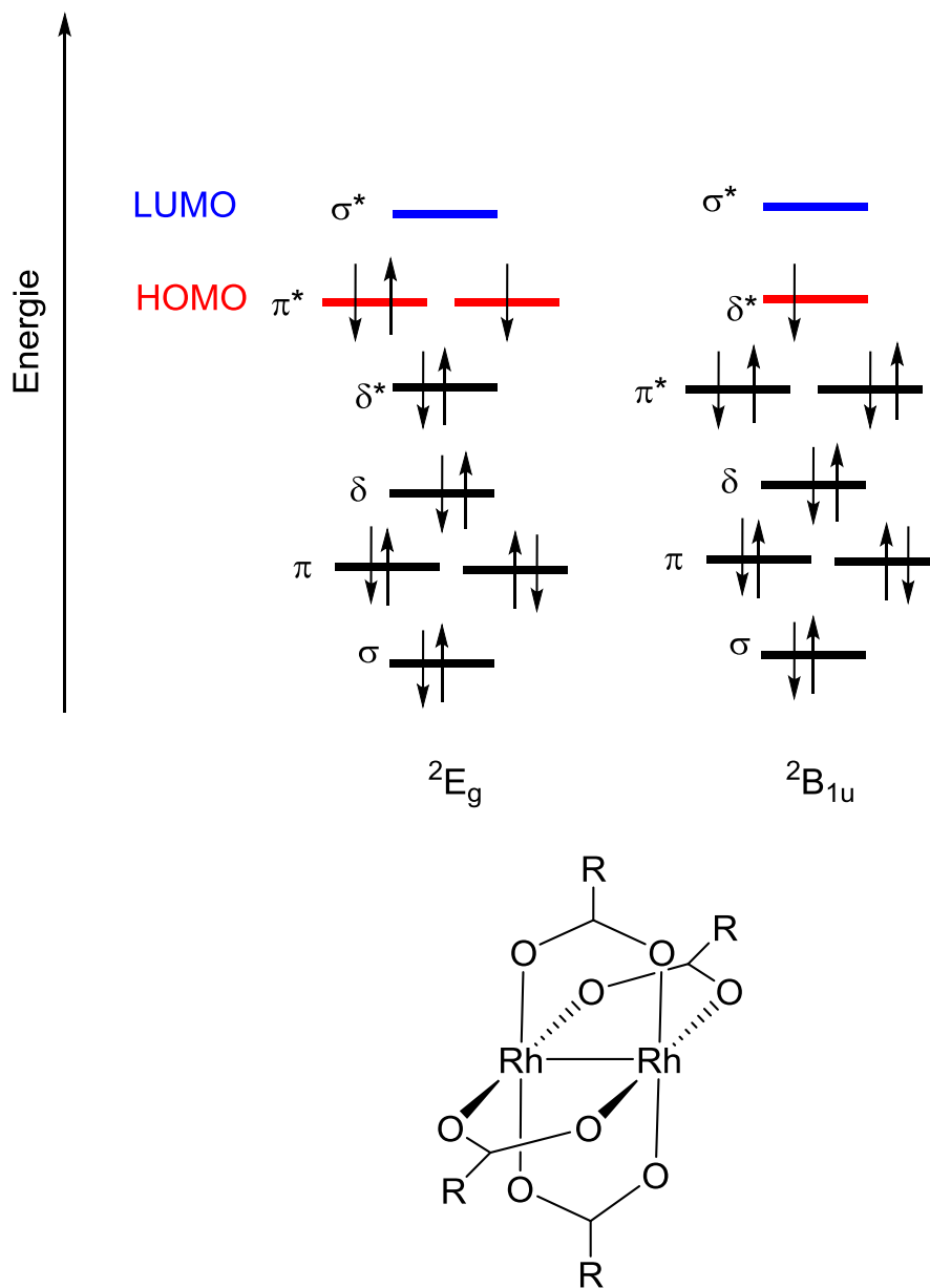
Figure 190 : Diagrammes orbitaux qualitatifs d'un dimère Rh^{II}-Rh^{II} .
