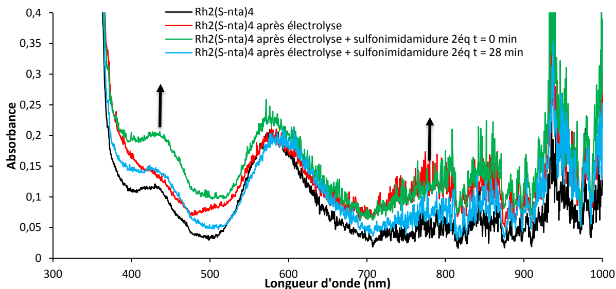
Figure 18 : Evolution du spectre d'absorption UV-visible d'une solution de \text{Rh}_2(\text{S-nta})_4 (0,62 mM) dans TCE/MeOH (3 : 1) + \text{TBAPF}_6 0,1 M à -20\text{ }^{\circ}\text{C} (noire), après électrolyse (rouge), après ajout de sulfonimidamide (vert puis violet).
