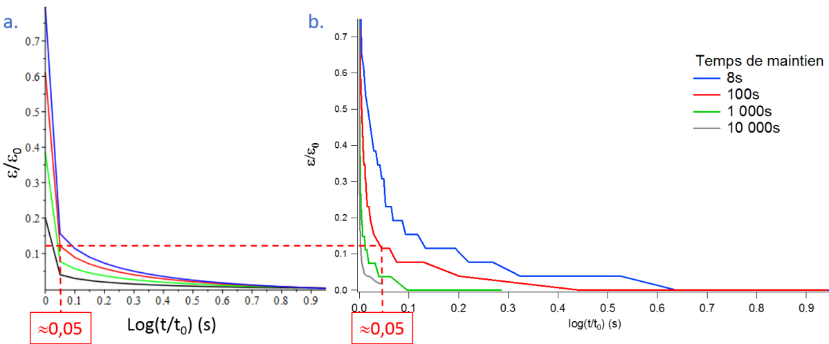
Figure 76 : Recouvrance relative à la déformation initiale pour m=0,1 , r=200 et \tau=10^{23} s (a.) pour différents temps de maintien en compression : 10^{-6} s (noir), 10^{-2} s (vert), 10^2 s (rouge) et 10^6 s (bleu) pour le modèle (b.) et pour des temps de maintien de 8 s (noir), 10^2 s (rouge), 10^3 s (vert) et 10^4 s (gris) pour les données expérimentales. Les abscisses représentent le logarithme du rapport entre le temps d'observation t et le temps de maintien t_0 .
