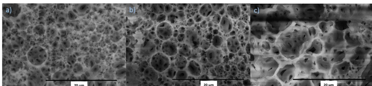
Figure 42 : Images MEB de mousses de MAC 4 (a), MAC 12 (b) et MAC 18 (c) pour 15 mol% de tensioactif, 20 mol% réticulant et 80 vol% de phase dispersée.
