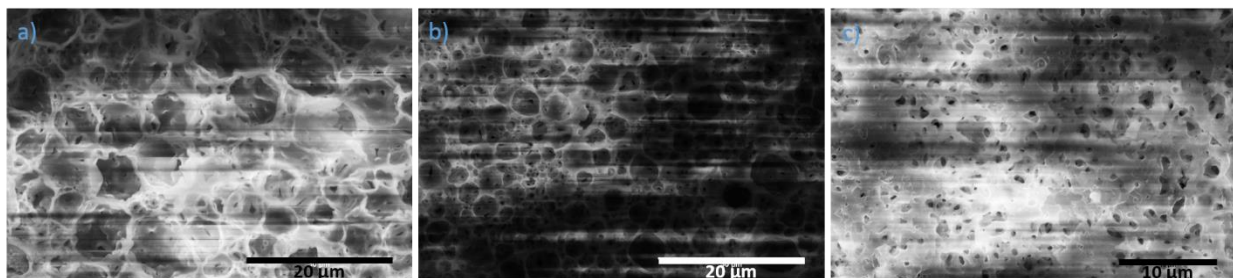
Figure 37 : Images MEB des polyHIPEs à base de MAC 12 avec 15 mol% de tensioactif, 10 mol% de réticulant et a) 75 vol%, b) 80 vol% et c) 85 vol% de phase dispersée.
