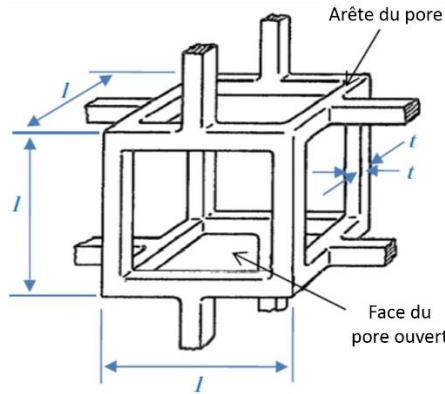
Figure 51 : Image du schéma d'un pore ouvert pour le modèle de Gibson et d'Ashby. Les faces sont ouvertes et la matrice est constituée uniquement d'arêtes à section cubique de longueur l et d'épaisseur t . 12
