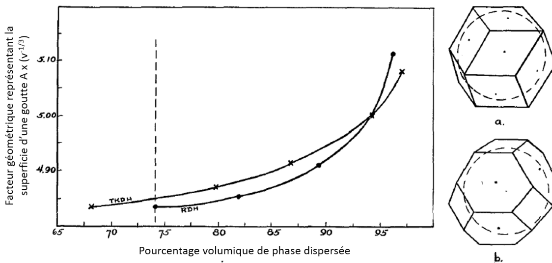
Figure 13 : Evolution de la surface d'une goutte en fonction du volume de phase interne (vol%). Schéma d'une géométrie dodécaèdre rhombique (a) et tétrakaïdécaédrique (b) 70 .
