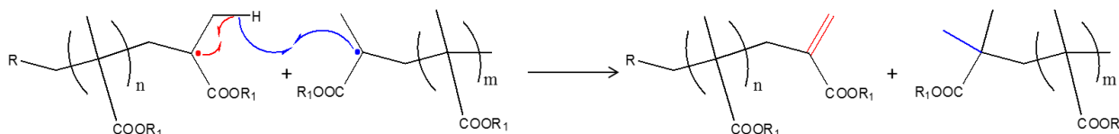
Figure 83 : Réaction de terminaison par dismutation de deux chaînes en croissance.
