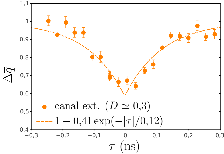
Figure 4.8: Mesures obtenues au voisinage de \tau \simeq 0 pour une excitation carré, boîte pincée.
