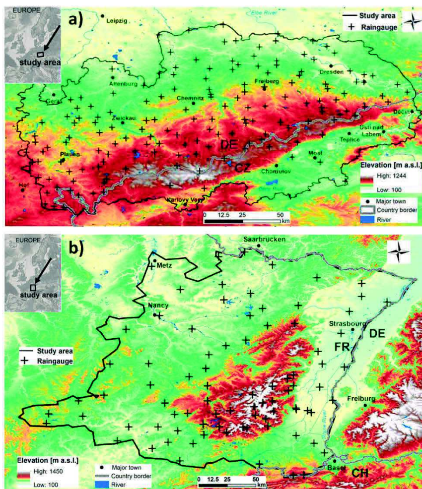
Figure 1 Zone d'étude et la distribution spatiale des pluviomètres dans (a) Monts Métallifères et (b) les Vosges. L'altitude est représentée en couleurs avec les sites élevés en blanc et les bas en vert.
