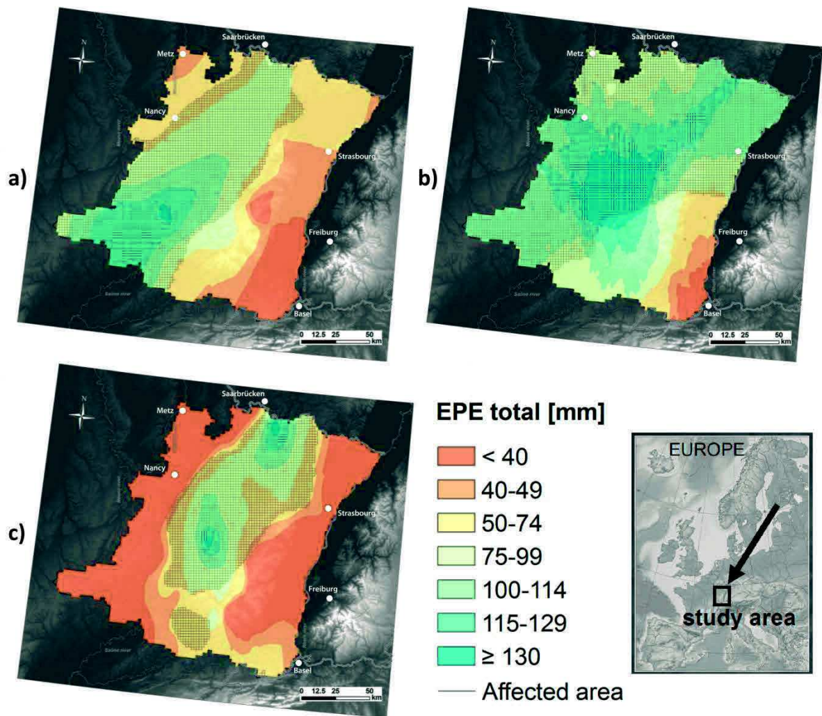
Figure 2 Totaux de précipitation représentés en grille en VG pour (a—c) les 3 EPEs les plus fortes (EPEs 1—3 dans la Table 1). La grille grise montre la zone touchée par les EPEs estimée via WEI. Les grilles sont d’une résolution 2x2 km.
