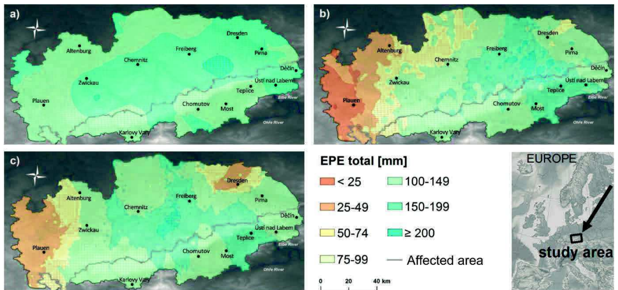
Figure 3 Totaux de précipitation représentés en grille en OM pour (a–c) les 3 EPEs les plus forts (EPEs 1–3 dans la Table 2). La grille grise montre la zone touchée par les EPEs estimée via WEI. Les grilles sont d’une résolution 2x2 km.
