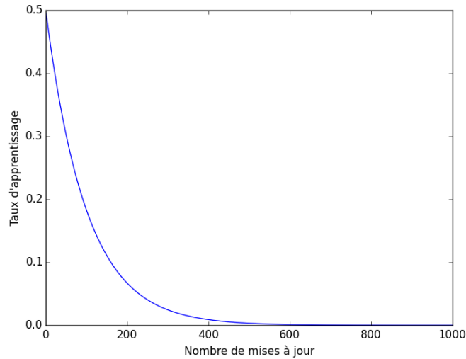
FIGURE 3.14 – Evolution du taux d'apprentissage lors de l'apprentissage de 10 000 symboles (soit 1000 mises à jour du taux d'apprentissage) issues de séquences RG avec le RNN-LSTM décrit section 3.3.2.
