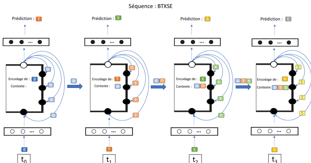
FIGURE 2.15 – Représentation schématique des étapes de la propagation avant dans un RNN-LSTM pour toute une séquence. Chaque symbole de la séquence est représenté par une couleur. Les symboles dotés d’une couleur plus claire représentent la version encodée des symboles présentés en entrée au réseau.
