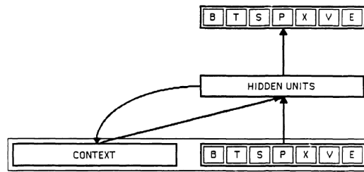
FIGURE 2.8 – Réseau de neurones récurrent simple de Elman décrit par Servan-Schreiber et al. [1988]
