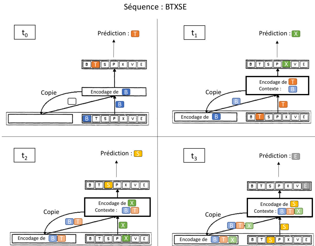
FIGURE 2.11 – Etapes de la propagation avant dans un SRN pour toute une séquence. Chaque symbole de la séquence est représenté par une couleur. Les symboles dotés d’une couleur plus claire représentent la version encodée des symboles présentés en entrée au réseau.
