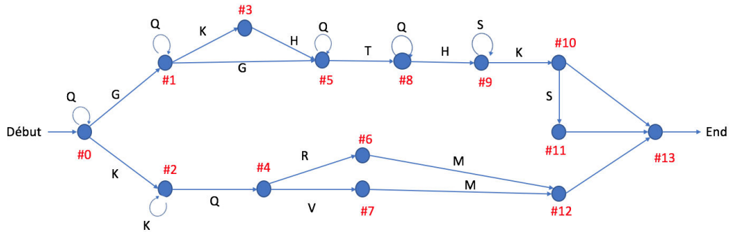
FIGURE 3.23 – Grammaire électrique issue de l'étude de 3 schémas électriques d'un même client
