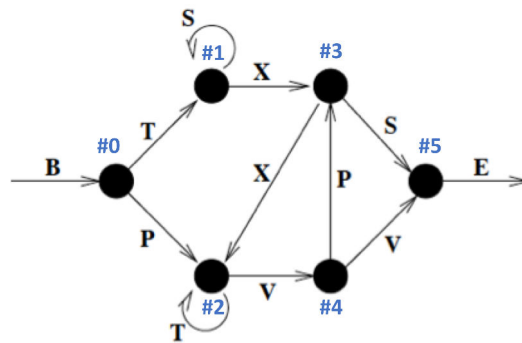
FIGURE 3.3 – Grammaire de Reber avec nœuds numérotés. Image extraite de Servan-Schreiber et al. [1988]
