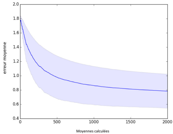
FIGURE 3.12 – Evolution de la moyenne de l’erreur lors de l’apprentissage du RNN-LSTM de 200 000 séquences issues de la grammaire de Reber Embarquée
