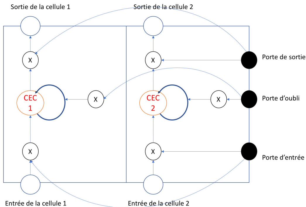
FIGURE 2.13 – Présentation d’une unité LSTM dotée d’un bloc composé de 2 cellules
