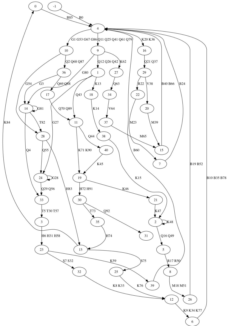
FIGURE 3.26 – Un graphe-automate avec étiquettes longues obtenu avec un algorithme k-means pour le clustering, où k=41 et issu d'un RNN-LSTM ayant appris des séquences EL. Extraction réalisée sur les 79 premiers pas de temps.
