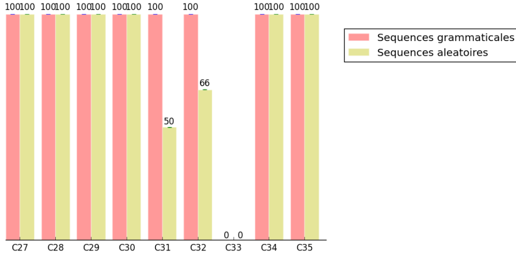
FIGURE 3.8 – Evolution des performances de Elman pour les configurations C27 à C35. Moyennes obtenues sur 10 simulations.
