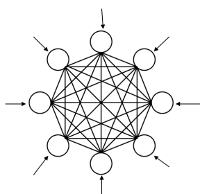
FIGURE 2.6 – Le modèle de Hopfield. Image extraite de Durand [1995]
