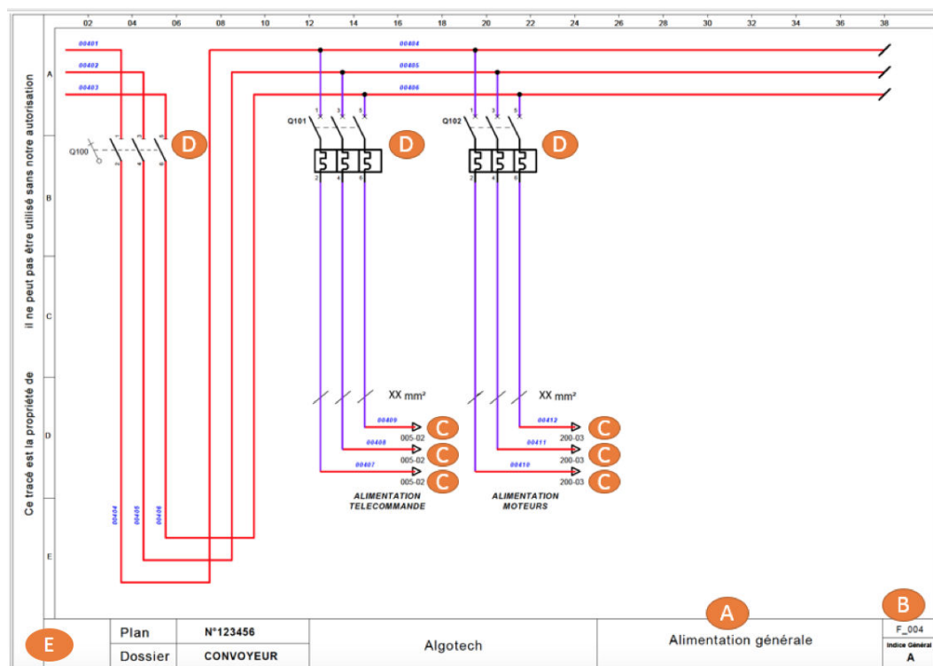
FIGURE 1.1 – Organisation et contenu du folio F_004 : A - Le titre du folio, B - Le numéro de folio, C - Les renvois folios, D - Les composants électriques, E - Le cartouche
