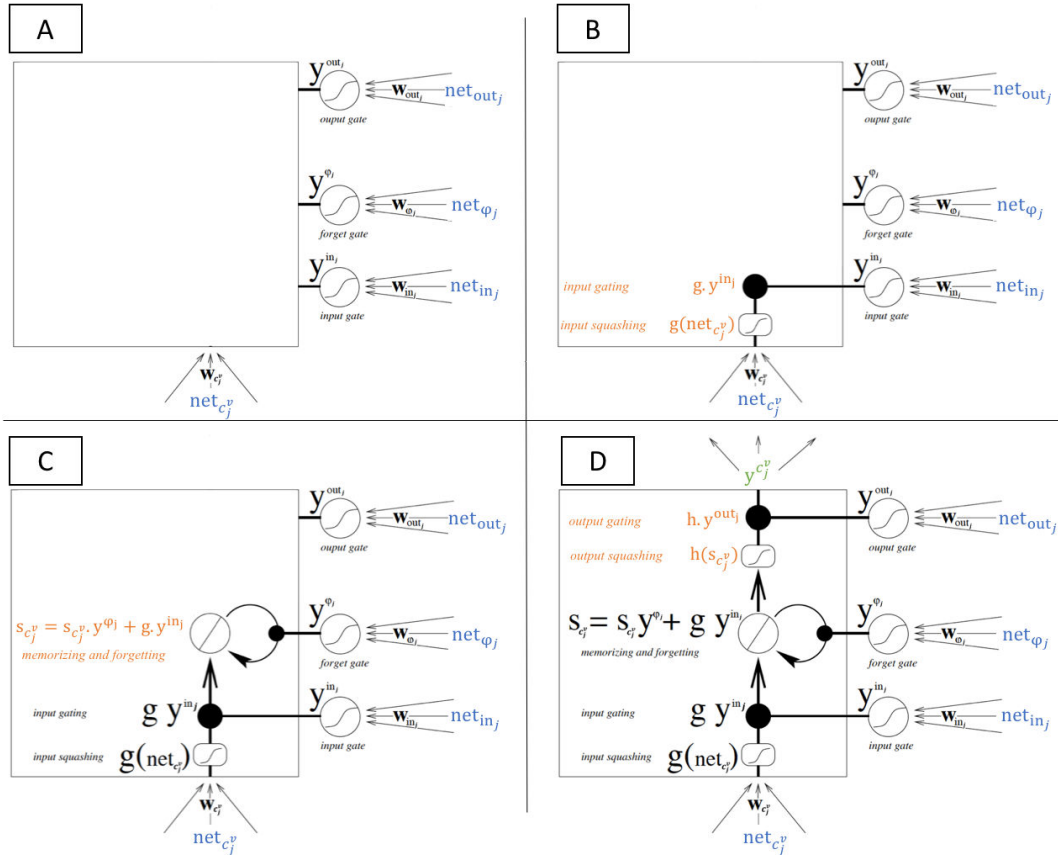
FIGURE 2.16 – Etapes de la propagation avant dans une unité LSTM dotée d'un bloc d'une cellule. Les informations entrantes dans une unité sont en bleu, celle sortante en vert. Les calculs au sein d'une cellule sont en orange.
