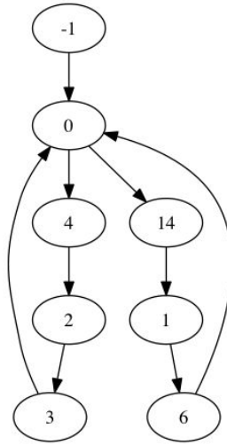
FIGURE 3.17 – Un graphe-automate sans étiquette obtenu avec un algorithme k-means pour le clustering, où k=15 , et issu d'un RNN-LSTM ayant appris des séquences RG. Extraction réalisée sur les 50 premiers pas de temps.
