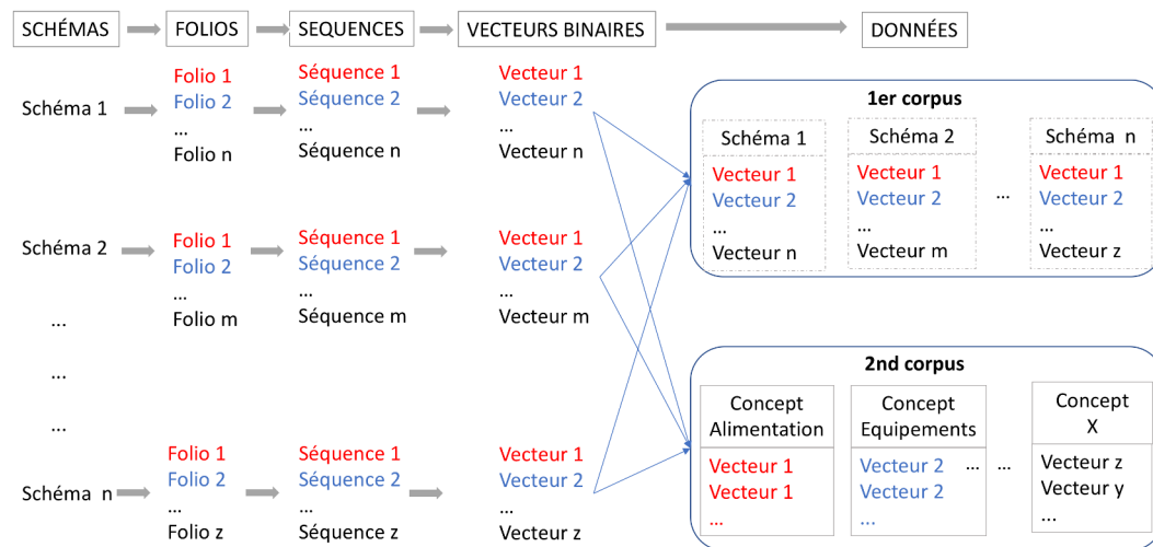
FIGURE 1.8 – Présentation des étapes de constitution des corpus. Les éléments qui partagent une même couleur appartiennent au même concept métier. Dans le 1er corpus, les pointillés indiquent les schémas d'origines dont sont issus les vecteurs.
