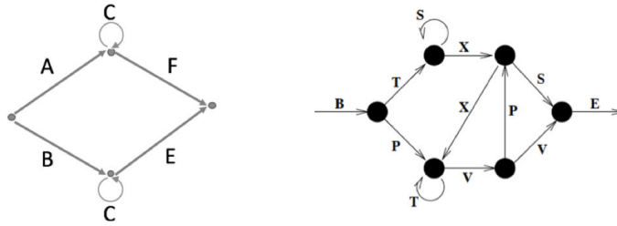
FIGURE 3.2 – Grammaire manuelle à gauche et Grammaire de Reber à droite (Image extraite de Servan-Schreiber et al. [1988] )
