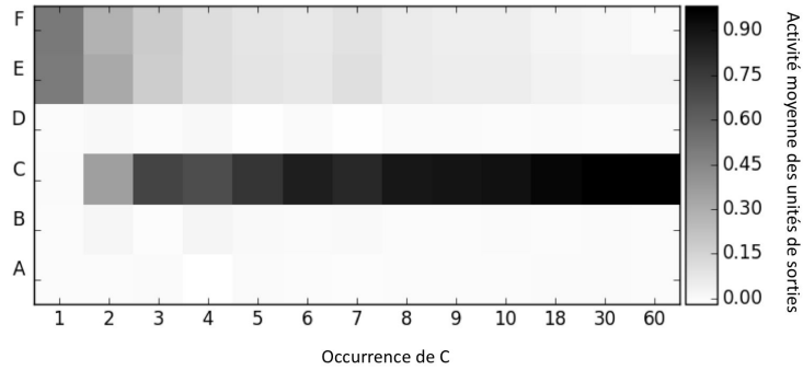
FIGURE 3.9 – Activité moyenne des unités de la couche de sortie pour un SRN de 3 unités cachées. Apprentissage réalisé avec : taux d'apprentissage=0.01 et momentum=0.01.
