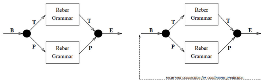
FIGURE 3.4 – Grammaire de Reber embarquée à gauche et Grammaire de Reber embarquée et continue à droite. Images extraites de Servan-Schreiber et al. [1988]
