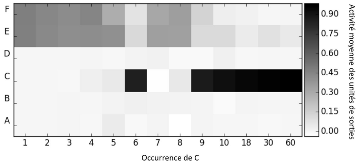
FIGURE 3.10 – Activité moyenne des unités de la couche de sortie pour un SRN de 15 unités cachées. Apprentissage réalisé avec : taux d'apprentissage=0.01 et momentum=0.01.
