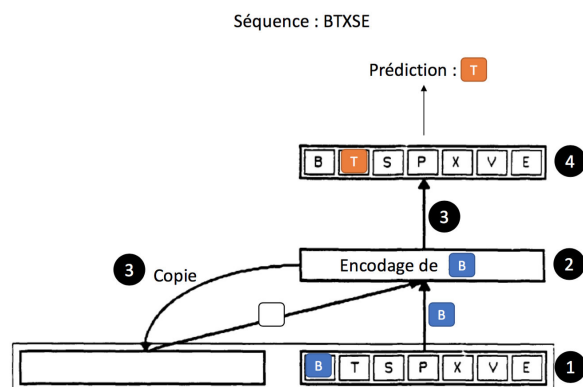
FIGURE 2.10 – Etapes de la propagation avant à un instant t dans un SRN
