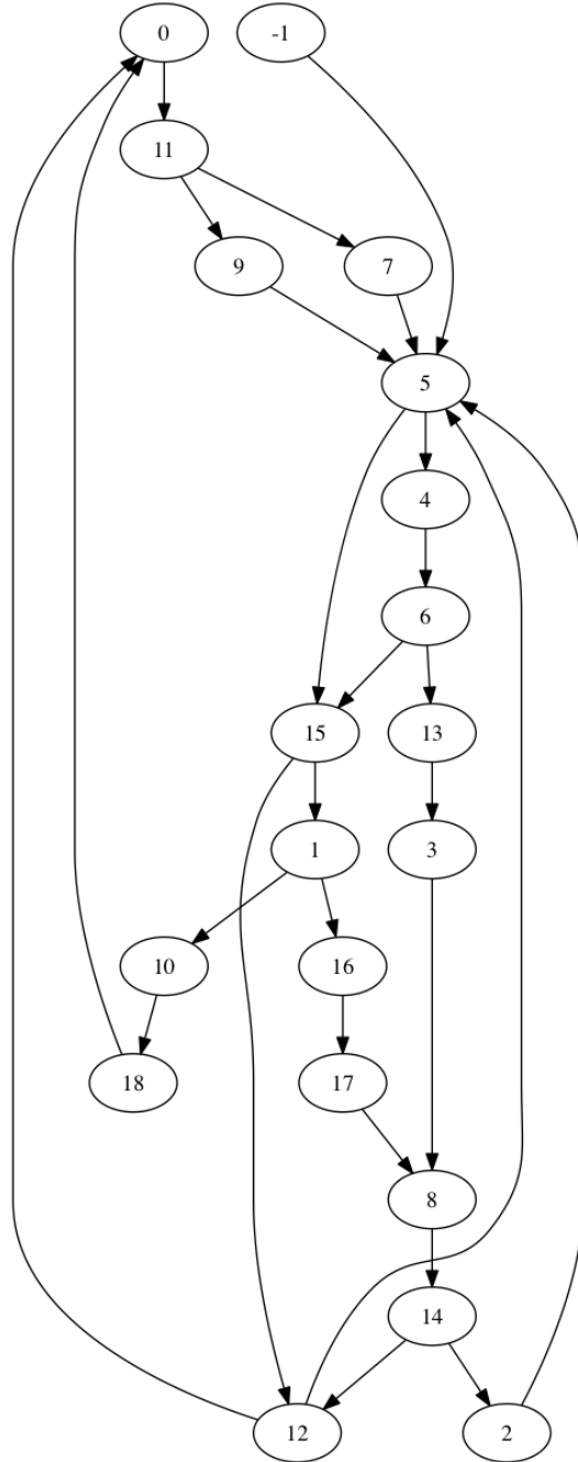
FIGURE 3.20 – Un graphe-automate sans étiquette obtenu avec un algorithme k-means pour le clustering, où k=19 et issu d'un RNN-LSTM ayant appris des séquences ERG. Extraction réalisée sur les 80 premiers pas de temps.
