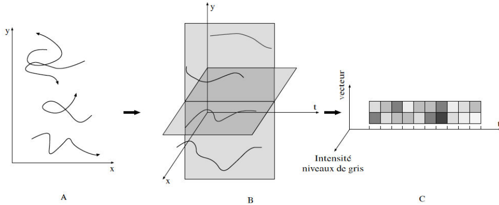
FIGURE 2.3 – Classification de séquences pour les modèles à représentation externe du temps.
