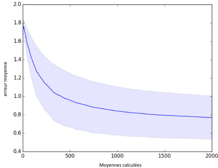
FIGURE 3.11 – Evolution de la moyenne de l'erreur lors de l'apprentissage du RNN-LSTM de 200 000 séquences issues de la grammaire de Reber
