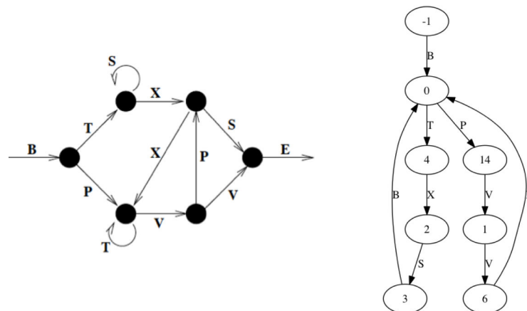
FIGURE 3.29 – Grammaire de Reber à droite et Graphe-automate extrait à gauche (pour 50 premiers pas de temps).
