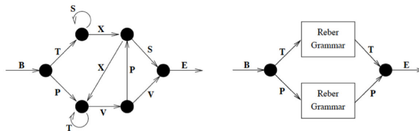
FIGURE 3.16 – La grammaire de Reber à gauche et la grammaire de Reber embarquée à droite
