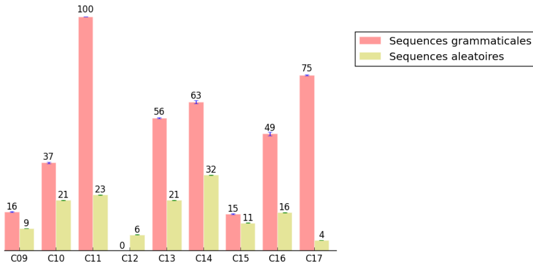
FIGURE 3.6 – Evolution des performances d’un SRN de 3 unités cachées pour les configurations C9 à C17. Moyennes obtenues sur 10 simulations.
