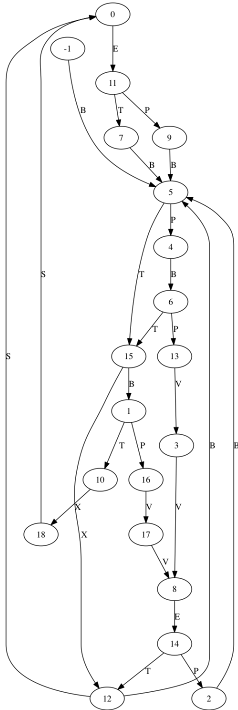
FIGURE 3.22 – Un graphe-automate final non-compressé obtenu avec un algorithme k-means pour le clustering, où k=19 et issu d'un RNN-LSTM ayant appris des séquences ERG. Extraction réalisée sur les 80 premiers pas de temps.
