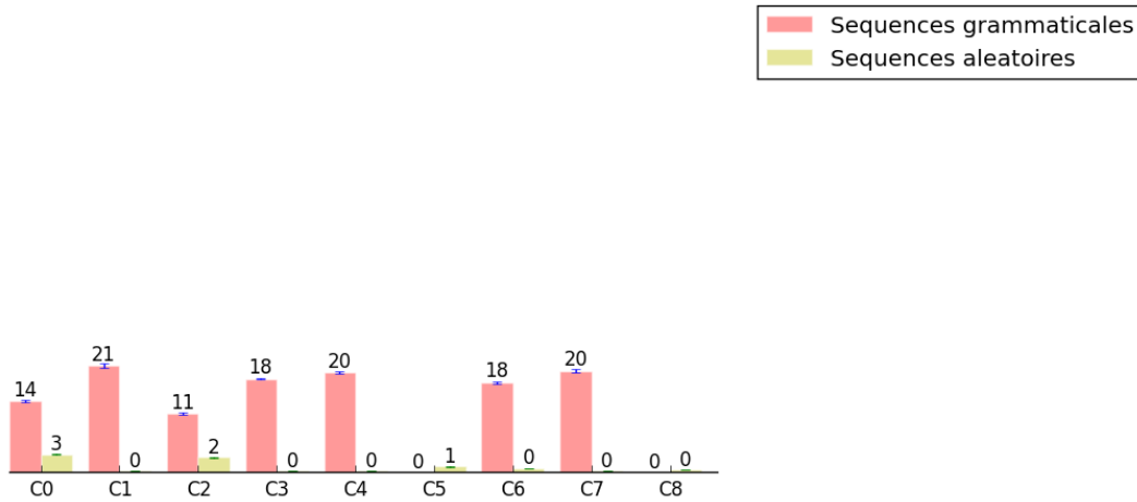
FIGURE 3.5 – Evolution des performances d’un SRN de 3 unités cachées pour les configurations C0 à C8. Moyennes obtenues sur 10 simulations.
