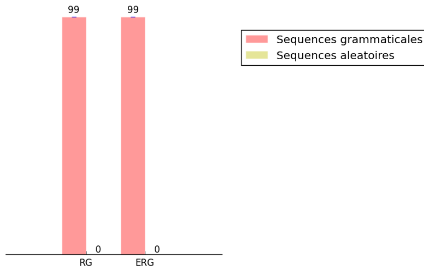
FIGURE 3.13 – Performances moyennes sur 10 simulations pour RNN-LSTM appliquées à la grammaire de Reber (RG) et la grammaire de Reber embarquée (ERG).
