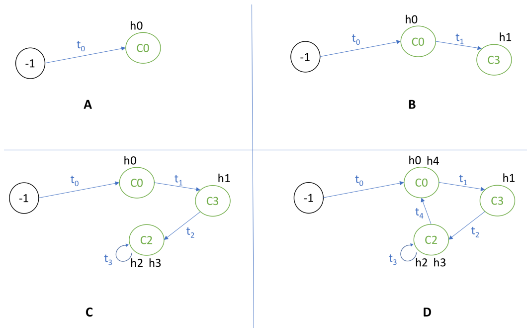
FIGURE 3.15 – Exemple de génération d’automate avec une liste-patterns [h0, h1, h2, h3, h4] et une liste-cluster [0\ 3\ 2\ 2\ 0] .
