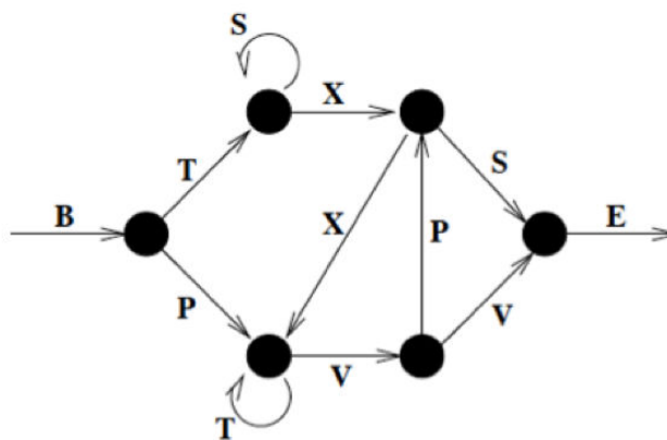
FIGURE 2 – Exemple de grammaire artificielle : B désigne "Begin" et E désigne "End". Image inspirée de Reber [1967], extraite Servan-Schreiber et al. [1988]
