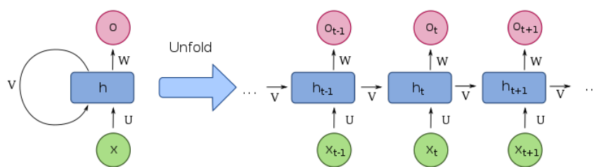
FIGURE 2.9 – Représentation d’un RNN déplié. Image issue de Deloche [2017]
