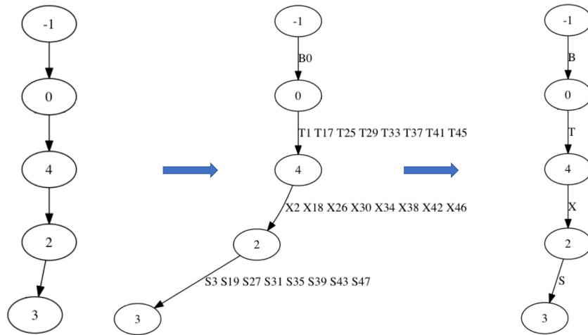
FIGURE 3.28 – Règles extraites à partir d’un RNN-LSTM ayant appris des séquences RG. Exemples issus, de gauche à droite, du graphe-automate sans étiquettes (figure 3.17), du graphe-automate doté d’étiquettes longues (figure 3.18) et du graphe-automate avec une étiquette simple (figure 3.19)
