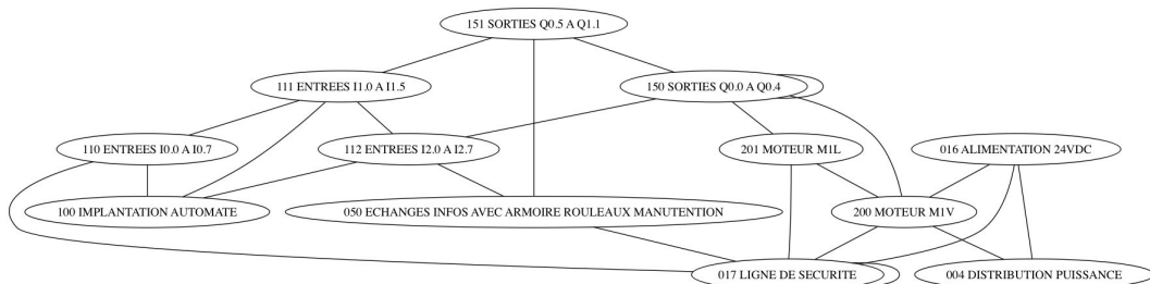
FIGURE 1.4 – Graphe original du schéma électrique A de 43 pages : seuls les folios comportant des renvois folios et donc des portions de circuits électriques sont représentées.
