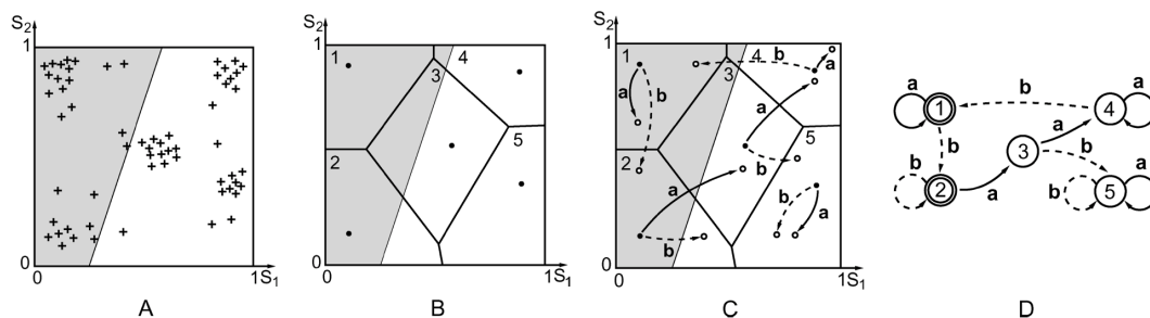
FIGURE 2.18 – Exemple d'extraction de règles à travers une recherche en largeur dans un espace d'états groupés par k-means. A - Les états du RNN sont échantillonnés pendant l'entraînement. B - Ces états sont regroupés en un nombre prédéfini de clusters. C - Une recherche en largeur est effectuée (voir la figure 2.17). D - L'automate est construit. Images extraites de Jacobsson [2005]
