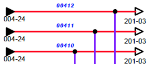
FIGURE 1.3 – Agrandissement des renvois folios du folio 200
