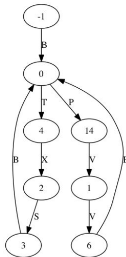
FIGURE 3.19 – Un graphe-automate final obtenu avec un algorithme k-means pour le clustering, où k=15 et issu d'un RNN-LSTM ayant appris des séquences RG. Extraction réalisée sur les 50 premiers pas de temps.
