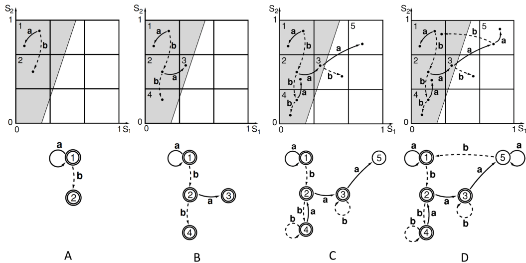
FIGURE 2.17 – Itérations d'un algorithme d'extraction d'automate avec un paramètre de quantification q = 3 utilisé sur un RNN avec deux neurones, entraîné sur un langage binaire. L'espace d'état est divisé en une région d'acceptation et une de rejet (respectivement en gris et en blanc). L'algorithme développe le graphe jusqu'à ce que tous les nœuds aient deux arcs sortants. A et B représentent les deux premières itérations, C et D représentent les 2 dernières. Exemples de Giles et al. [1991] extrait de Jacobsson [2005]
