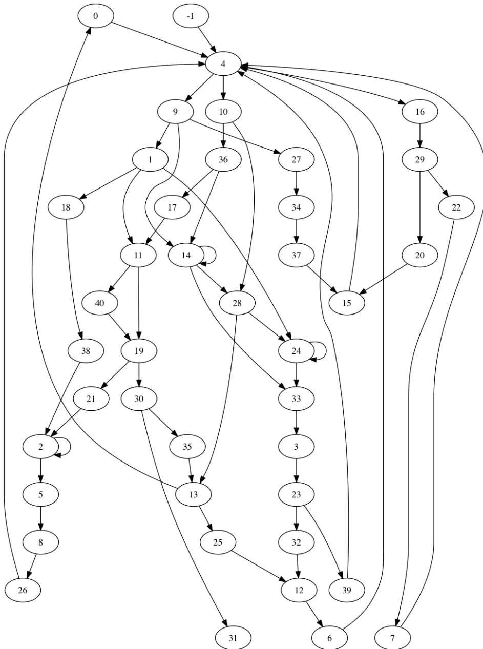
FIGURE 3.25 – Un graphe-automate sans étiquette obtenu avec un algorithme k-means pour le clustering, où k=41 et issu d'un RNN-LSTM ayant appris des séquences EL. Extraction réalisée sur les 79 premiers pas de temps.
