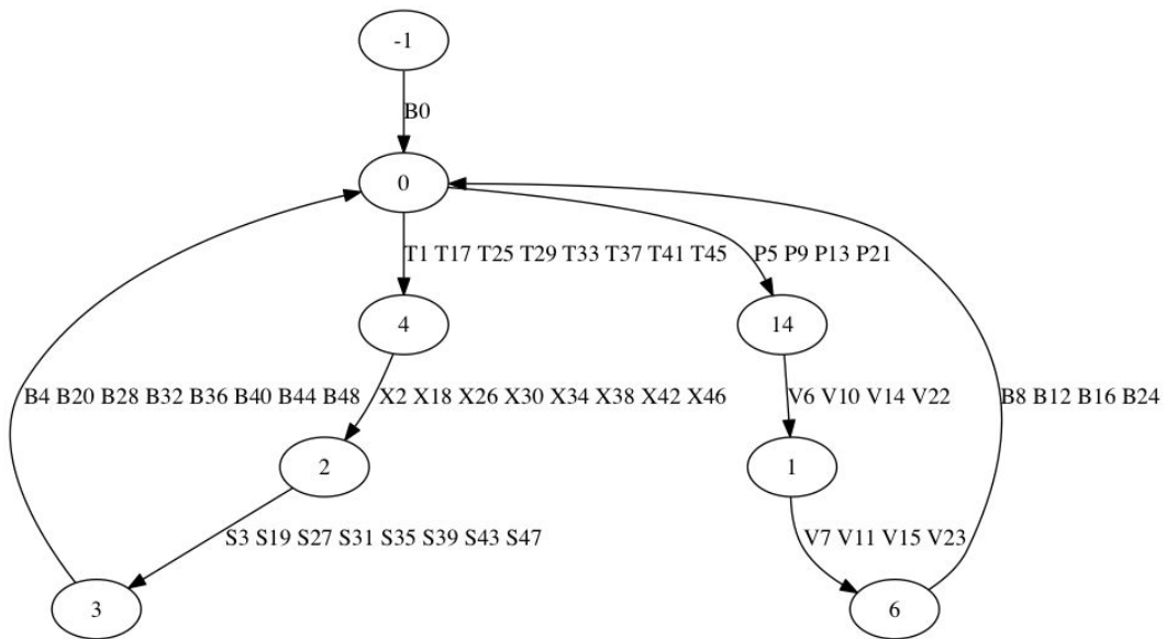
FIGURE 3.18 – Un graphe-automate avec étiquettes longues obtenu avec un algorithme k-means pour le clustering, où k=15 et issu d'un RNN-LSTM ayant appris des séquences RG. Extraction réalisée sur les 50 premiers pas de temps.
