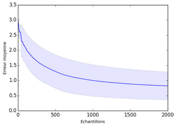
FIGURE 3.24 – Evolution de la moyenne de l'erreur lors de l'apprentissage du RNN-LSTM de 200 000 séquences issues de la grammaire électrique.
