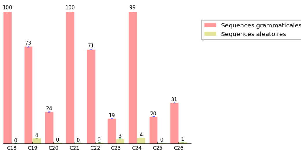
FIGURE 3.7 – Evolution des performances d'un SRN de 15 unités cachées pour les configurations C18 à C26. Moyennes obtenues sur 10 simulations.
