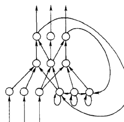
FIGURE 2.7 – Le modèle de Jordan. Image extraite de Servan-Schreiber et al. [1991]
