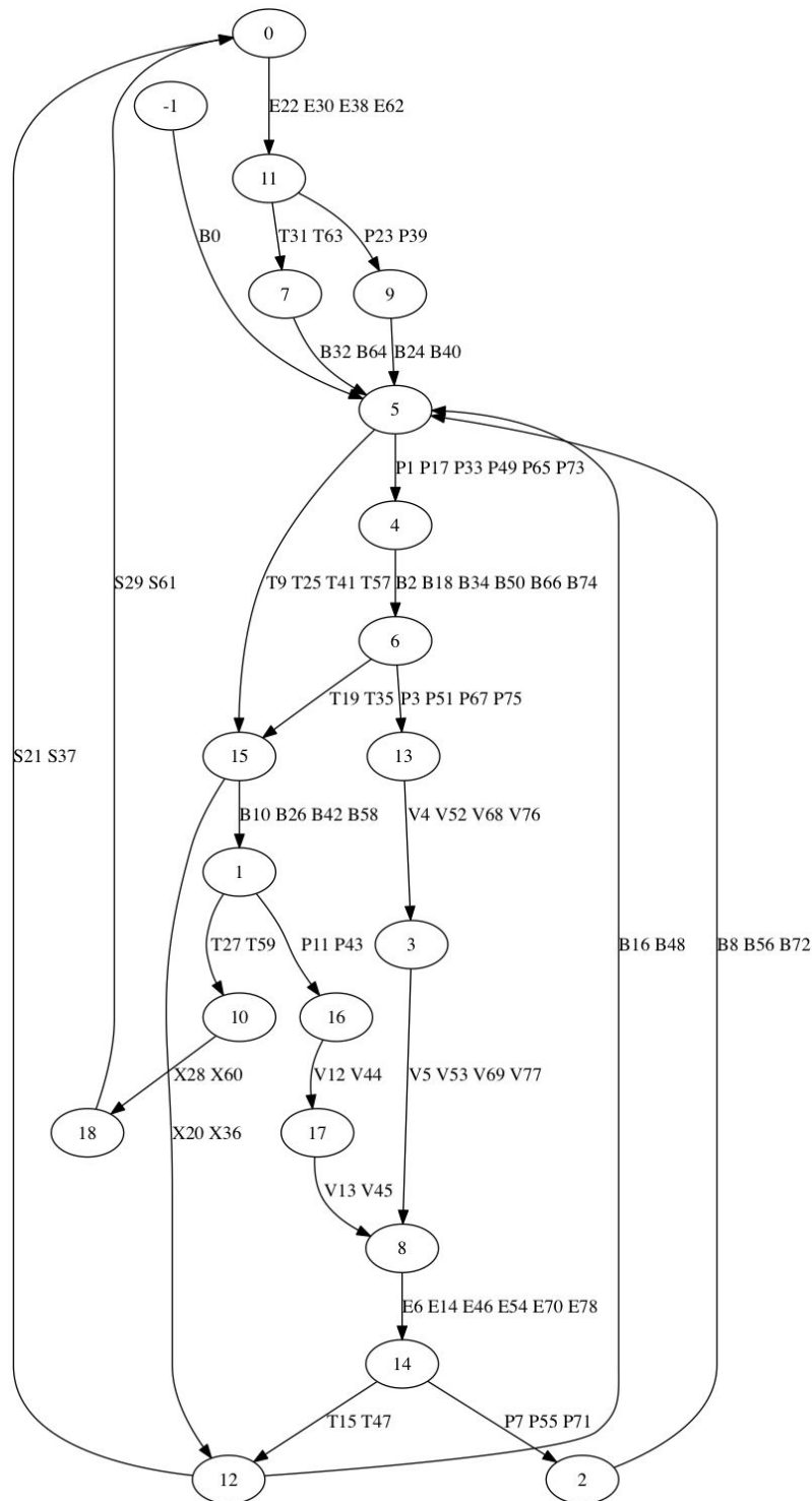
FIGURE 3.21 – Un graphe-automate avec étiquettes longues obtenu avec un algorithme k-means pour le clustering, où k=19 et issu d'un RNN-LSTM ayant appris des séquences ERG. Extraction réalisée sur les 80 premiers pas de temps.
