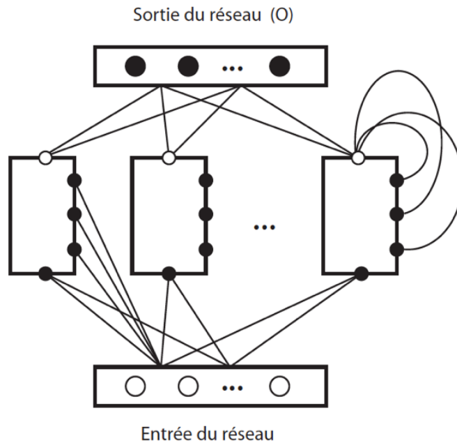
FIGURE 2.12 – Présentation d'un réseau doté d'unités LSTM au niveau de la couche cachée. Image issue de Lapalme [2006]
