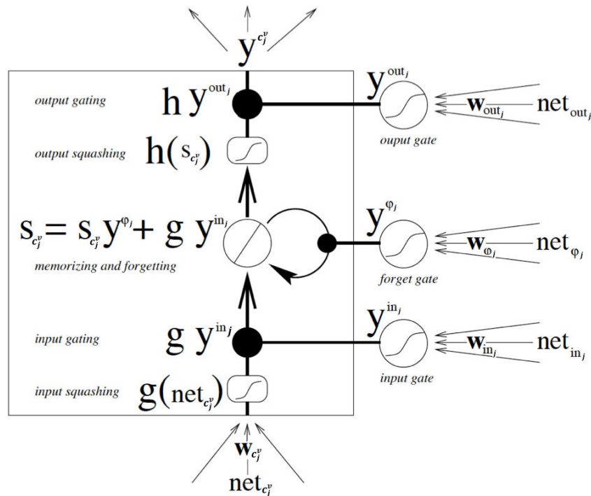
FIGURE 2.14 – Présentation d'une unité LSTM doté d'un bloc, lui même doté d'une cellule. Image issue de Gers et al. [1999]
