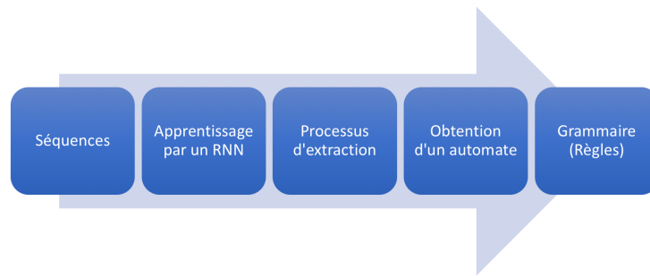
FIGURE 2.1 – Présentation schématique du processus d'extraction des règles à partir d'un RNN
