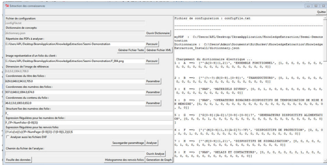
FIGURE 1.13 – Interface d'accueil du prototype d'extraction des connaissances réalisé
