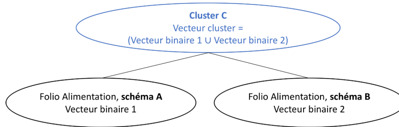
FIGURE 1.10 – Portion d’un arbre de cluster résultant du clustering hiérarchique : les vecteurs binaires des clusters-nœuds, résultent de l’union des vecteurs binaires des clusters-fils.
