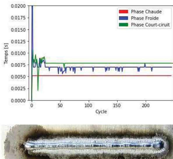
Figure 4.65 Réduction du défaut en début de cordon détectable sur le signal de durée des phases, grâce à l'augmentation de l'intensité I_{\text{boost}}
