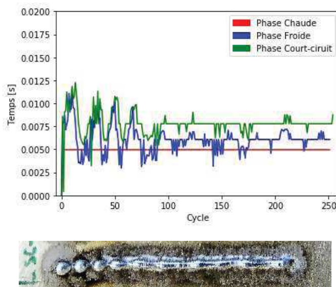
Figure 4.66 Forme du signal de l'évolution des durées des phases révélant le défaut de « humping »
