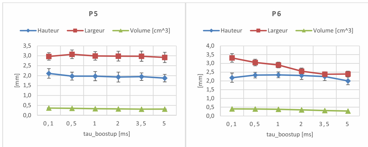
Figure A2.12: Caractéristiques géométriques en fonction du paramètre \tau_{\text{boostup}}
