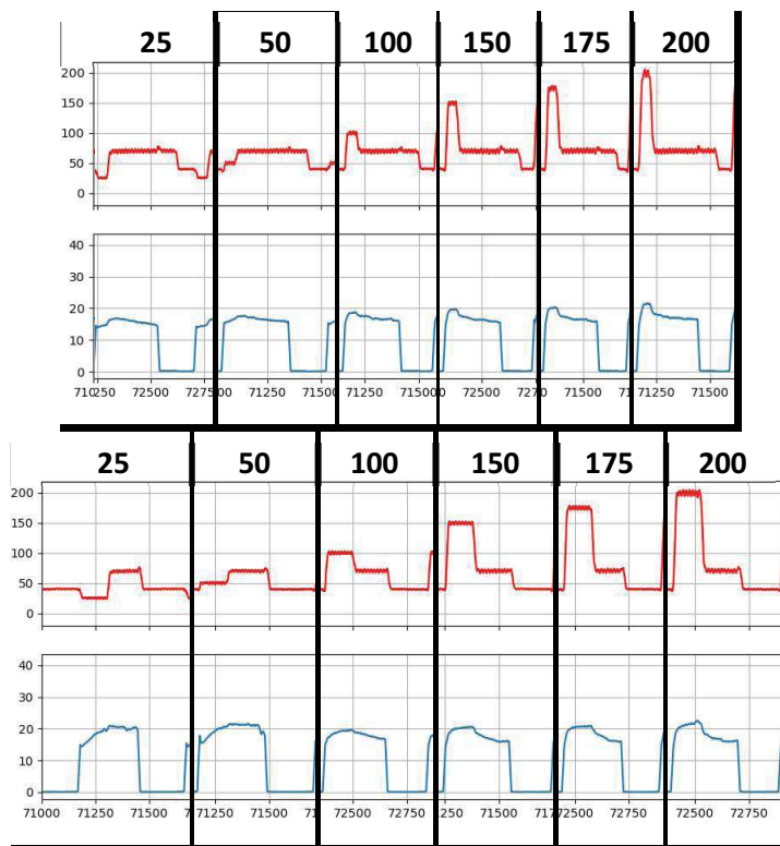
Figure A2.14: Modifications du cycle CMT avec différentes valeurs de I_{\text{boost}} a) P5 b) P6
