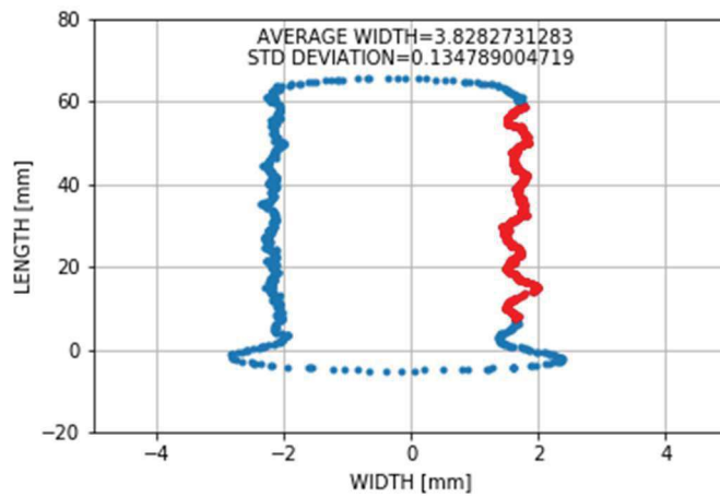
Figure 2.26 : Représentation du contour du cordon dans une coupe longitudinale parallèle au plan du substrat, et séparation des points du contour en deux catégories pour la mesure de largeur
