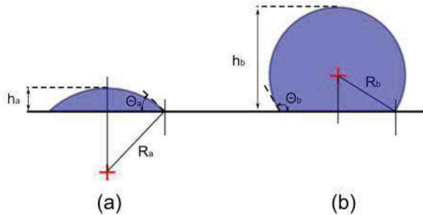
Figure 4.6 Géométries simplifiées de macro-goutte, (a) pour un angle de mouillage inférieur à 90^\circ , et (b) pour un angle de mouillage supérieur à 90^\circ
