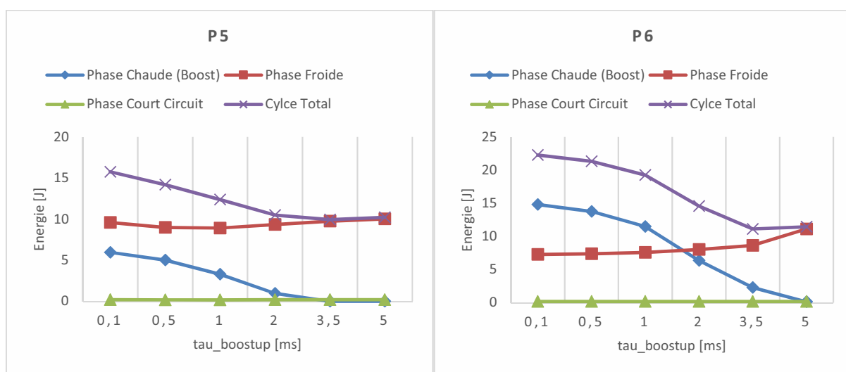
Figure A2.10: Energie apporté par phase dans les cycles CMT
