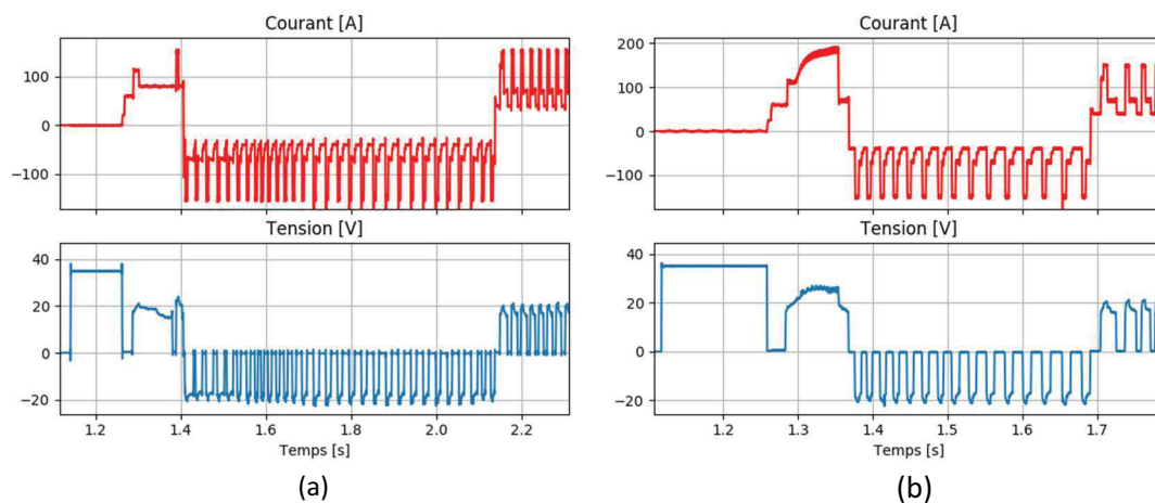
Figure 4.21 Forme d'onde du courant et de la tension durant la phase de démarrage de cordon avec le mode « advanced », (a) sans Hotstart, (b) avec Hotstart
