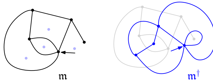
Figure I.2 – Une carte \mathbf{m} et son dual \mathbf{m}^\dagger . Les flèches indiquent les coins racines.
