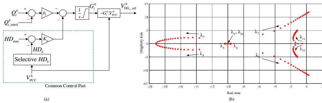
FIGURE 5 : Schéma du contrôleur harmonique droop.
