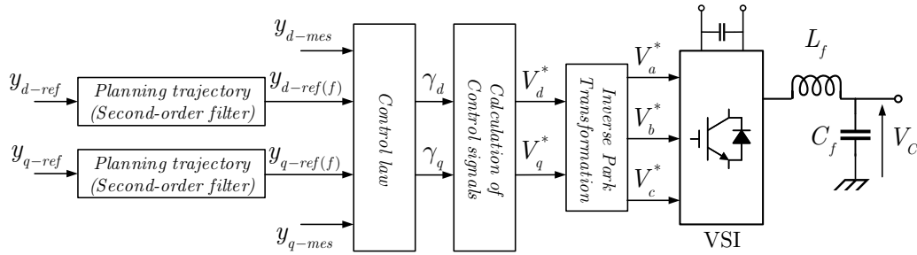
FIGURE 2 : Schéma fonctionnel de la commande basée sur la platitude.
