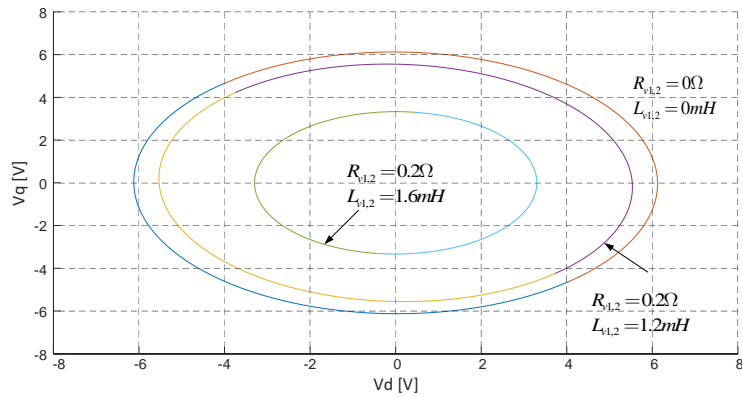
FIGURE 12 : Effet de l'inductance virtuelle L_v sur le bassin estimé de la stabilité asymptotique.
