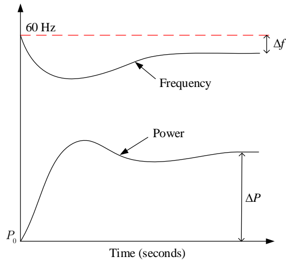
FIGURE 1 : Réponse transitoire d'un générateur synchrone.
