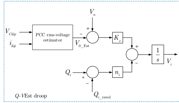
FIGURE 3 : Schéma du contrôleur Q - VEst .
