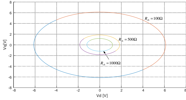
FIGURE 11 : Bassin d'attraction estimé pour le système sous l'effet de la charge résistive.
