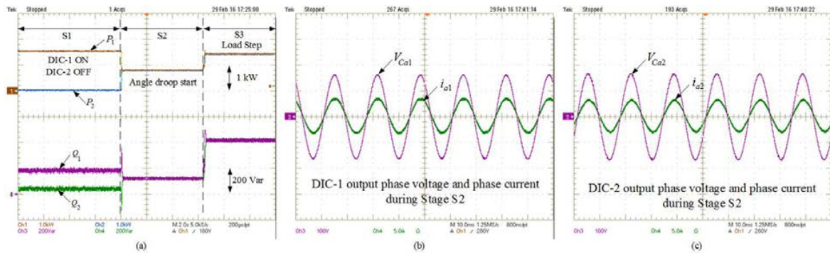
FIGURE 10 : Résultats expérimentaux : (a) Puissances active et réactive entre deux DG ; (b-c) Tension et courant pour chaque DIC-1 et DIC-2.
