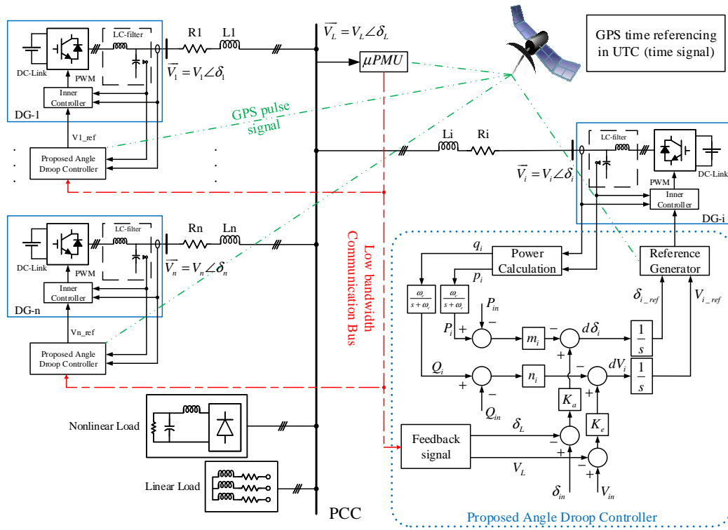
FIGURE 8 : Micro-réseaux avec schéma ensemble Angle s'affaisser contrôle proposé.
