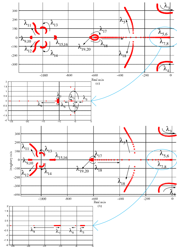
FIGURE 9 : Lieu des pôles pour différentes valeurs des coefficients du contrôleur "angle droop" proposé.
