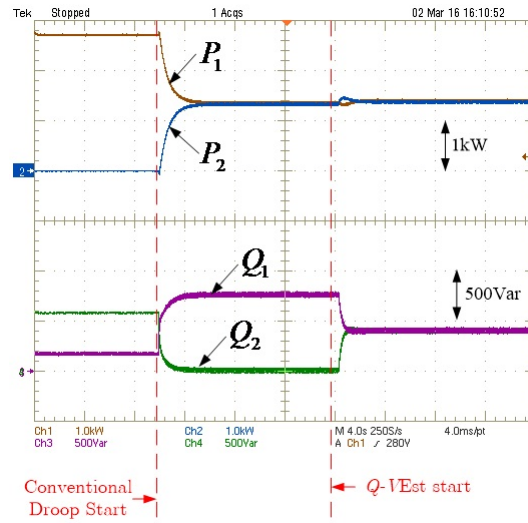
FIGURE 4 : Résultats expérimentaux : Répartition des puissances active et réactive entre deux DGs avant et après l'activation de l'algorithme proposé.
