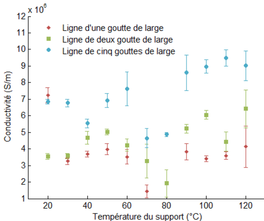
Figure V.12 : Conductivité des lignes imprimées en fonction de la température du support
