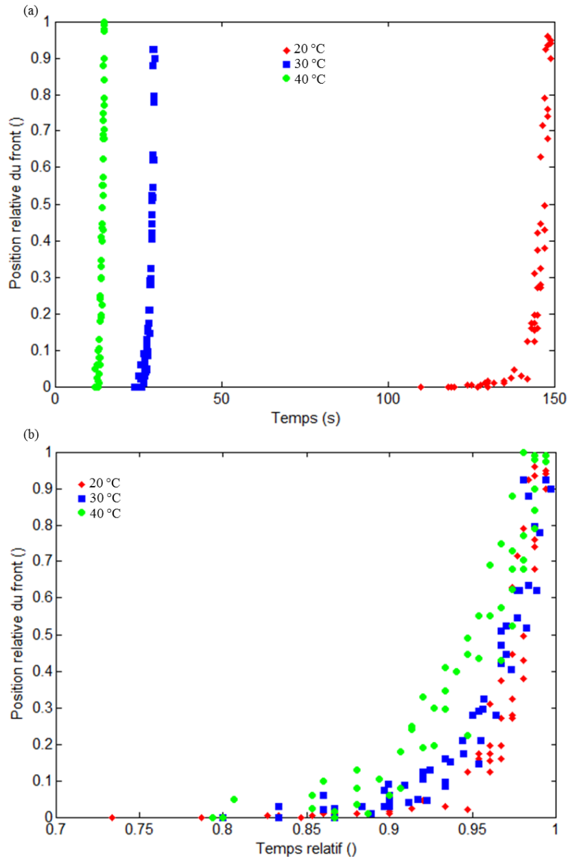
Figure IV.13 : Position relative du front en fonction (a) du temps et (b) du temps relatif ( t_{relatif} = t/t_{séchage} )
