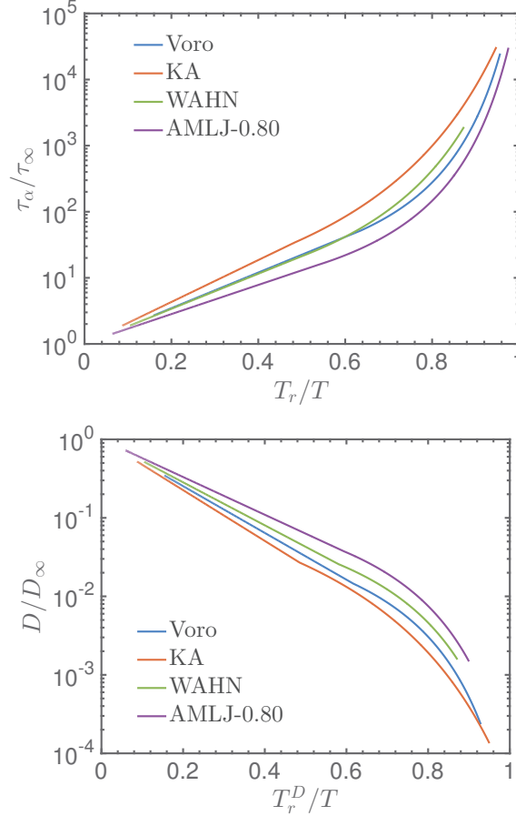
FIGURE 7: Comparaison de l'évolution de \tau_\alpha / \tau_\infty (haut) et de D / D_\infty (bas) en fonction de la température adimensionnée T_r / T . \tau_\infty et D_\infty sont des constantes extraites du fit Arrhénien à haute température. T_r et T_r^D sont des températures de référence arbitrairement choisies comme les températures pour lesquelles \tau_\alpha = 4 \cdot 10^4 et D(T_r^D) = 10^5 .
