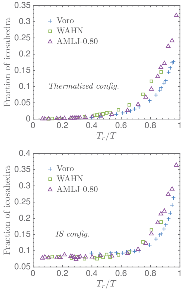
FIGURE 15: Evolution de la fraction d'icosaèdres en fonction de T_r/T pour le liquide de Voronoï bidisperse et deux liquides LJ. Les fractions ont été calculées pour des configurations thermalisées (haut) et également pour des configurations correspondant à des IS (bas).
