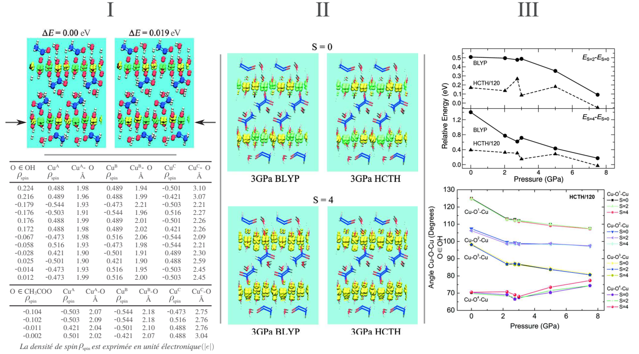
FIGURE 3 – I) Partie supérieure : structure optimisée de l’hydroxyde acétate de cuivre \text{Cu}_2(\text{OH})_3(\text{CH}_3\text{COO})\cdot\text{H}_2\text{O} ( \text{CuOHAc} ) dans la configuration antiferromagnétique (spin total S = 0 ) pour les deux distributions de densité de spin les plus stables du système. Les atomes Cu sont marron, C en bleu, O en rouge, H en blanc et les surfaces solides correspondent à des isosurfaces de densité de spin ( \alpha en vert et \beta en jaune) à une valeur de \pm 0.03 \text{ e}/\text{\AA}^3 (adapté à partir de la Figure 1 de la référence [36]). Partie inférieure : Valeurs de densité de spin ( \rho_{spin} ) localisées sur les deux types d’atomes d’oxygène (voir texte) en correspondance avec la densité de spin et les distances des trois atomes de cuivre voisins (adapté du TABLEAU 4 de la référence [36]). II) distribution de la densité de spin pour le système \text{CuOHAc} sous l’effet d’une pression de 3 GPa, calculée avec les fonctions d’échange-corrélation BLYP (gauche) et HCTH (droite) et pour deux états de spin total du système, S = 0 (en haut) et S = 4 (en bas). Résultats adaptés des figures 2 et 3 de la référence [37]. III) Partie supérieure : énergies totales relatives, par rapport à la configuration S = 0 (AF), des états de spin S = 2 et S = 4 du système \text{CuOHAc} en fonction de la pression appliquée et pour les deux fonctionnelles d’échanges-corrélations considérées. Partie inférieure : angles \text{Cu}\hat{\text{O}}\text{Cu} en fonction de la pression, pour chaque oxygène (appartenant à \text{CH}_3\text{CO}_2^- ) reliant les sites de cuivre dans la structure \text{CuOHAc} . Les courbes de \text{CuO}^i\text{Cu} ( i = 1-4 ) sont déplacées de manière rigide le long de l’axe des ordonnées (la figure originale et les valeurs numériques sont repris des tableaux 2, 3 et 4 et de la figure 4 de la référence [7])
