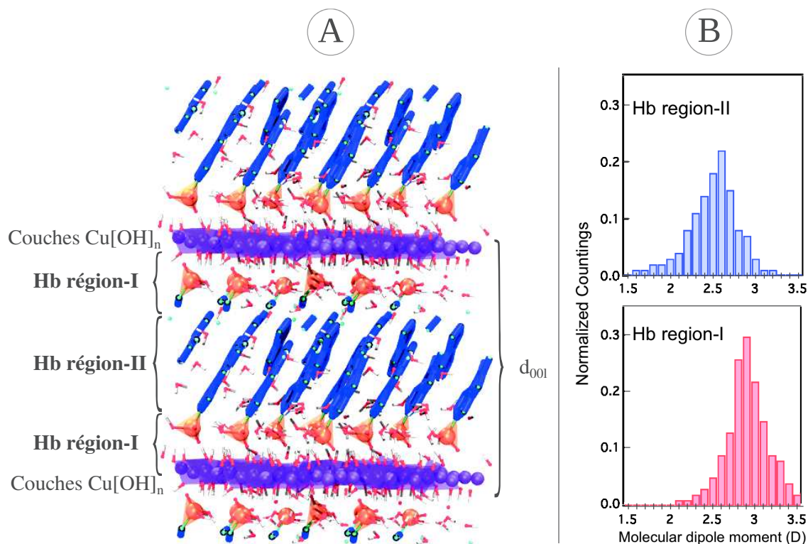
FIGURE 12 – A) Configuration typique de l'hydroxyde fluorène monophosphonique de cuivre obtenue via des simulations FPMD (la supercellule considérée est répliquée 2 \times 2 \times 2 le long de x, y et z pour plus de clarté). La distance interlamellaire ( d_{00l} ), les couches d'hydroxyde de cuivre ( \text{Cu}[\text{OH}]_n ) ainsi que les régions correspondantes aux type I et II de liaisons hydrogènes (H) sont également indiquées (voir texte). Couleurs : Cu en pourpre ; P en orange et \text{PO}_3 en polyèdres oranges ; C et squelette des groupes fluorène en bleu ; O en rouge ; H en blanc. B) Distributions normalisées du module des moments dipolaires moléculaires des molécules d'eau pour le même matériau CuOHFP1. Dans la partie interfaciale de l'espace interlamellaire, région I, correspond la distribution en bas de la figure (en rouge) et à la partie centrale de la structure, région II, correspond la distribution en haut de la figure (en bleu)
