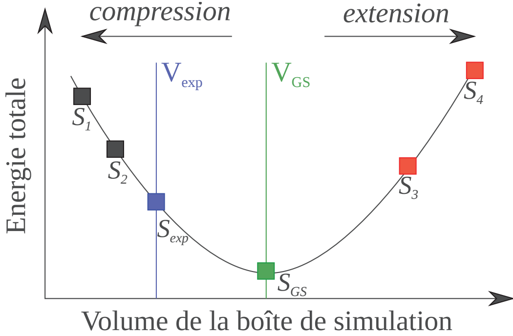
FIGURE 5 – Représentation schématique de la procédure d'évaluation de la pression appliquée sur les systèmes simulés pour la recherche de l'état fondamental structural ( P = 0 GPa). Le système expérimental est noté S_{exp} et est le système initial, puis après compression, les systèmes S_1 et S_2 sont obtenus ou après extension, les systèmes S_3 et S_4 sont obtenus. Dans la recherche de la structure d'équilibre optimisée du matériau ( S_{GS} à pression nulle), on évalue la dérivée de la courbe d'énergie totale en fonction du volume de la boîte de simulation et on obtient une estimation de la pression appliquée sur le système ( voir texte )
