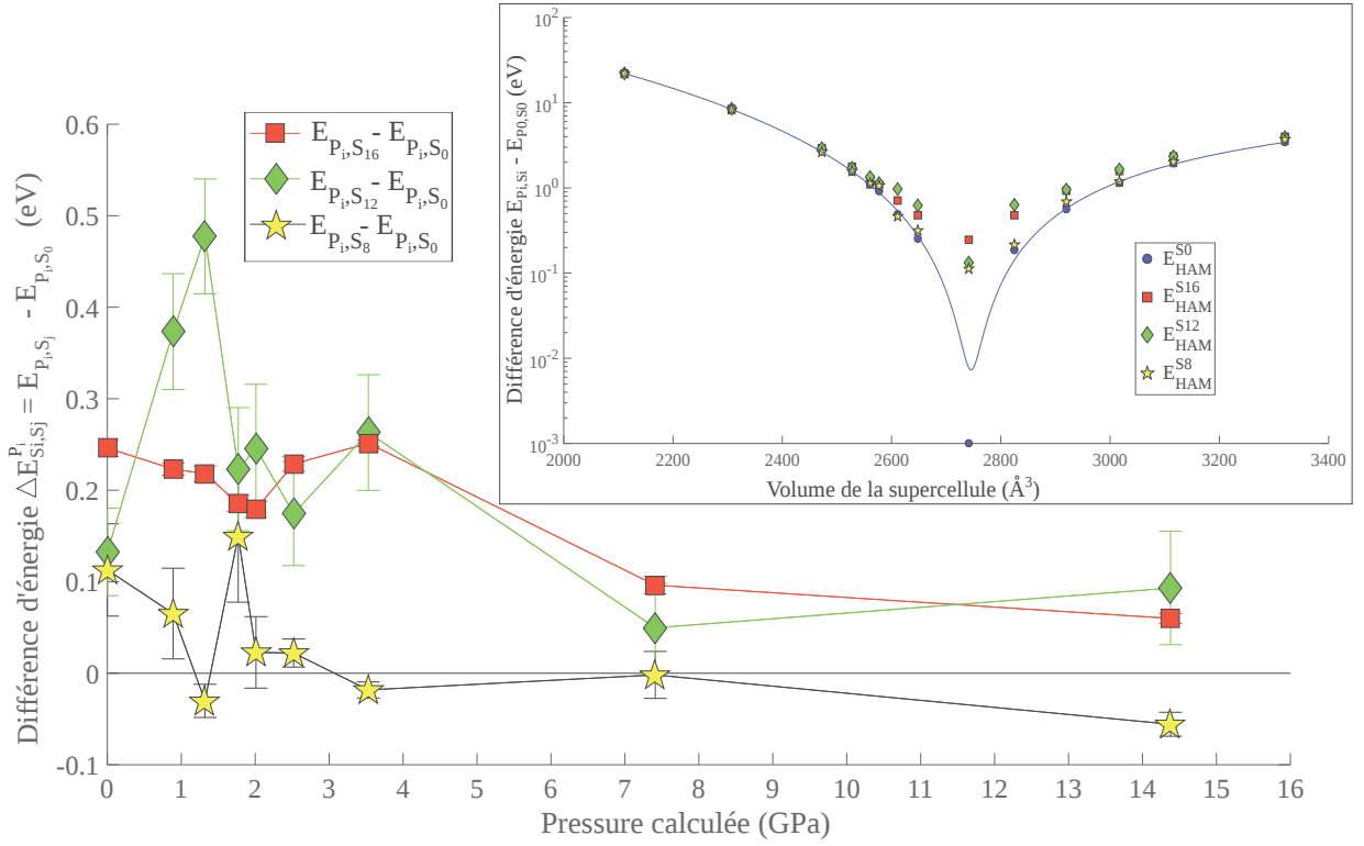
FIGURE 6 – Graphique principal : Stabilité relative (énergies totales) des deux états magnétiques intermédiaires ( S = 8 et S = 12 ) et les systèmes entièrement ferromagnétiques ( S = 16 ) par rapport à l'état fondamental anti-ferromagnétique (ligne en pointillés pour le cas S = 0 ). Encadré : équation d'état des structures considérées E_{\text{tot}}(V_{\text{SuperCell}})
