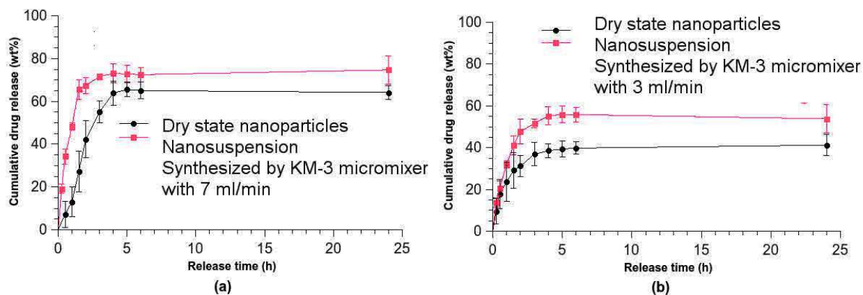
Figure 4. Profil de libération du principe actif modèle pour des nanoparticules séchées par pulvérisation puis redispersées et des nanoparticules non séchées et toutes deux produites avec deux débits d'eau différents: 7 ml/min (a) et 3 ml/min (b).
