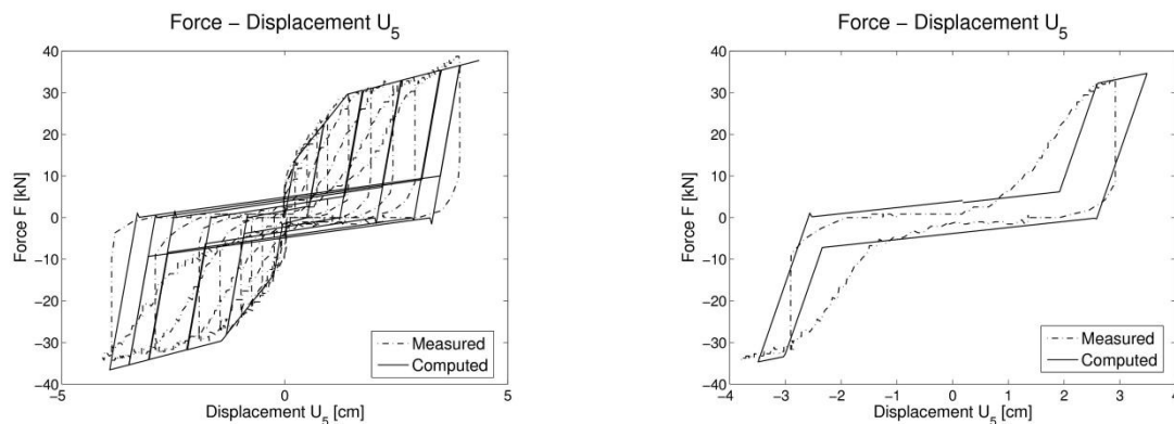
c) Hysteresis
