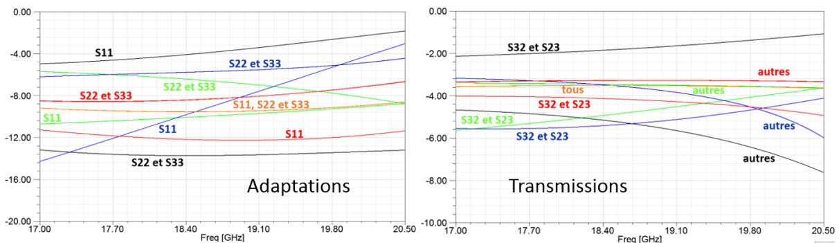
Figure 60 : Courbes des paramètres S en dB en simulation HFSS® pour les adaptations (à gauche) et les transmissions (à droite) des différents designs de té plan H : design 1 en noir, design 2 en rouge, design 3 en orange, design 4 en bleu et design 5 en vert
