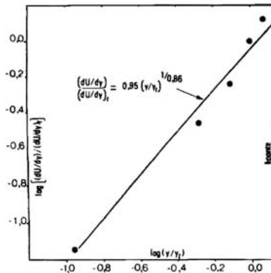
Figure X-5:Diagramme log-log montrant la bonne corrélation linéaire des valeurs du gradient de vitesse relatif et permettant de caractériser le comportement pseudoplastique du magma A lors de l'écoulement.
