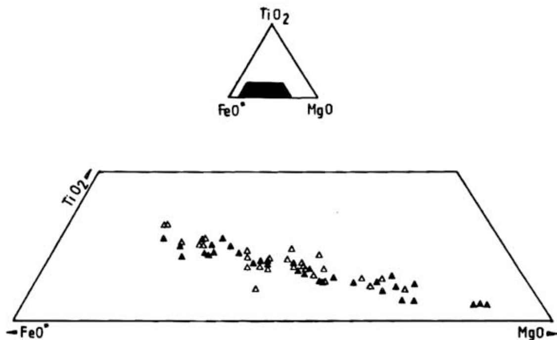
Figure XI.8: Diagramme triangulaire TiO_2, FeO, MgO . Noter la similitude d'évolution entre roches volcaniques basiques du Viséen inférieur (symboles ouverts) et faciès plutoniques septentrionaux du massif des Ballons (symboles fermés).
