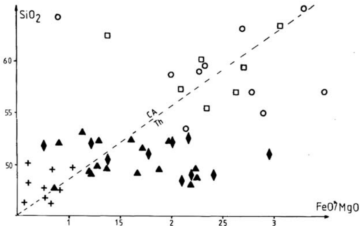
Figure VI-2: Diagramme SiO_2 , FeO/MgO . La limite séparant les domaines des champs calcoalcalins (CA) et tholéitiques (Th) a été reportée (Miyashiro, 1974). Mêmes symboles que figure VI-1.
