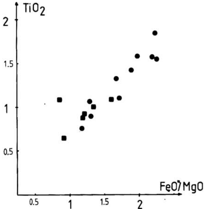
Figure IV-10: Diagramme TiO_2 , FeO^*/MgO . Noter la similitude avec la figure IV-9 et la bonne corrélation TiO_2-FeO . Explications dans le texte. Carrés : dolérites; cercles: diorites et microdiorites.
