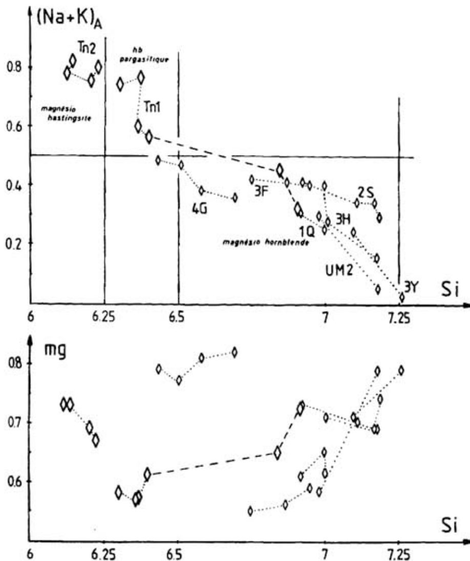
Figure IV-7: Diagramme (Na+K)_A, Si illustrant la variété de composition des amphiboles de dolérites (grands losanges) et microdiorites et diorites (Petits losanges). Les pointillés relient les compositions provenant d'un même échantillon.
