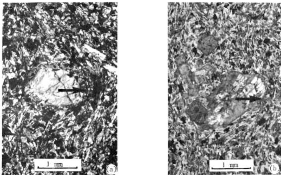
Figure X-8: Microphotographies illustrant les phénomènes de migration transversale de phénocristaux dans le faciès B, à 4cm de l'intraéponge A-B. L'écoulement se fait vers le haut, le coeur du filon est sur la droite des photos.
