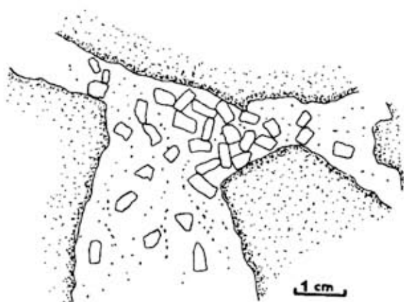
Figure VIII-10: Illustration du phénomène de Filter-press (Propach, 1973) Les phénocristaux de placioclases restent bloqués entre les enclaves; seul le liquide résiduel quartzofeldspathique peut s'injecter en filonnets.
