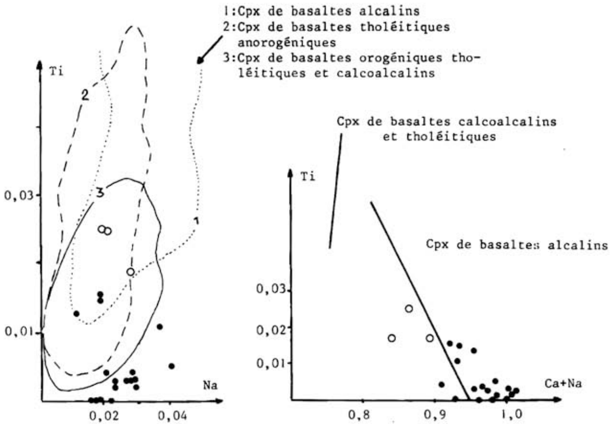
Figure XII.5: Projections des compositions des clinopyroxènes dans les diagrammes Ti, Na et Ti, Na+Ca proposés par Leterrier et Maury (1982).
