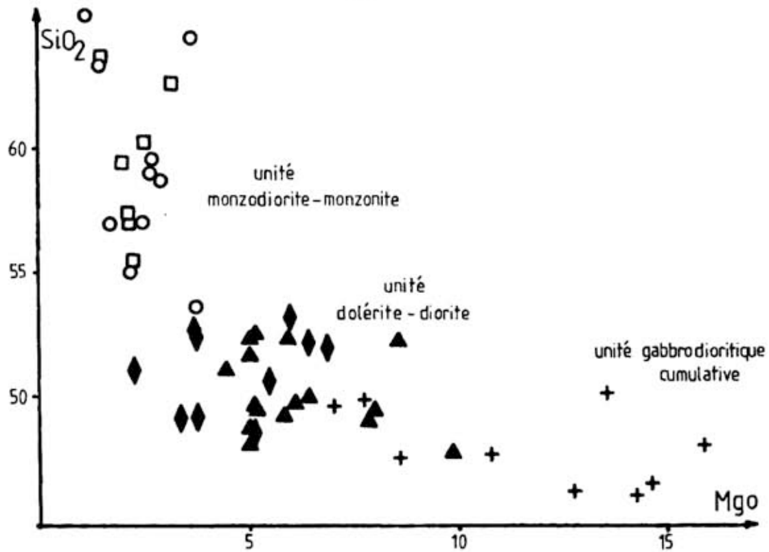
Figure VI-1: Diagramme SiO 2 ,MgO.Symboles ouverts:unité monzodiorite-monzonite;symboles fermés:unité dolérite-diorite;plus:unité cumulative.Les cercles et les losanges correspondent aux analyses C.R.P.G. répertoriées en annexe (explications dans le texte).
