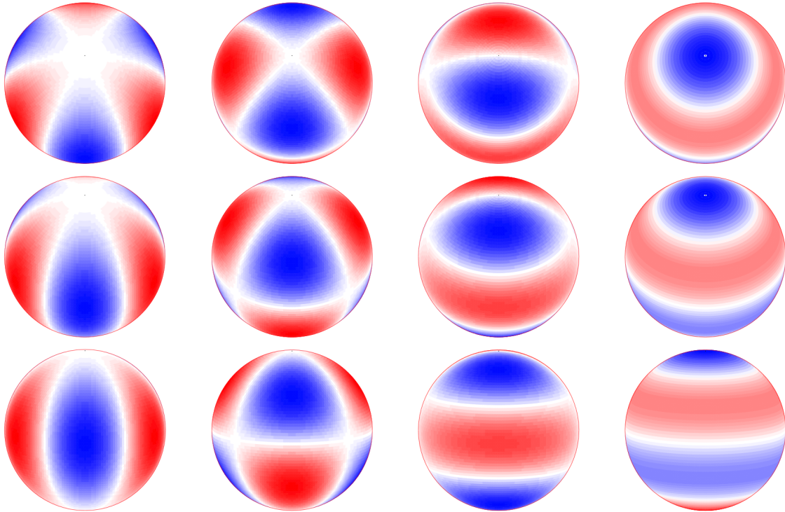
FIGURE 1.2 – Exemples d’harmoniques sphériques intervenant dans la description des oscillations stellaires. Celles-ci sont représentées pour différents angles de vue suivant l’inclinaison de l’axe polaire par rapport à la ligne de visée. Nous avons, du haut vers le bas, des inclinaisons respectives de 30^\circ , 60^\circ et 90^\circ . La valeur du degré est fixée à l = 3 tandis que les valeurs de l’ordre azimutal sont respectivement de m = 0, 1, 2 et 3 de la droite vers la gauche. Le système de couleurs indique les régions de l’étoile se rapprochant ou s’éloignant de son centre suivant le signe, respectivement négatif ou positif, de l’harmonique sphérique. Cette dernière s’annule au niveau des lignes nodales marquant la séparation entre les différentes régions. Figure tirée des notes de cours de C. Aerts.
