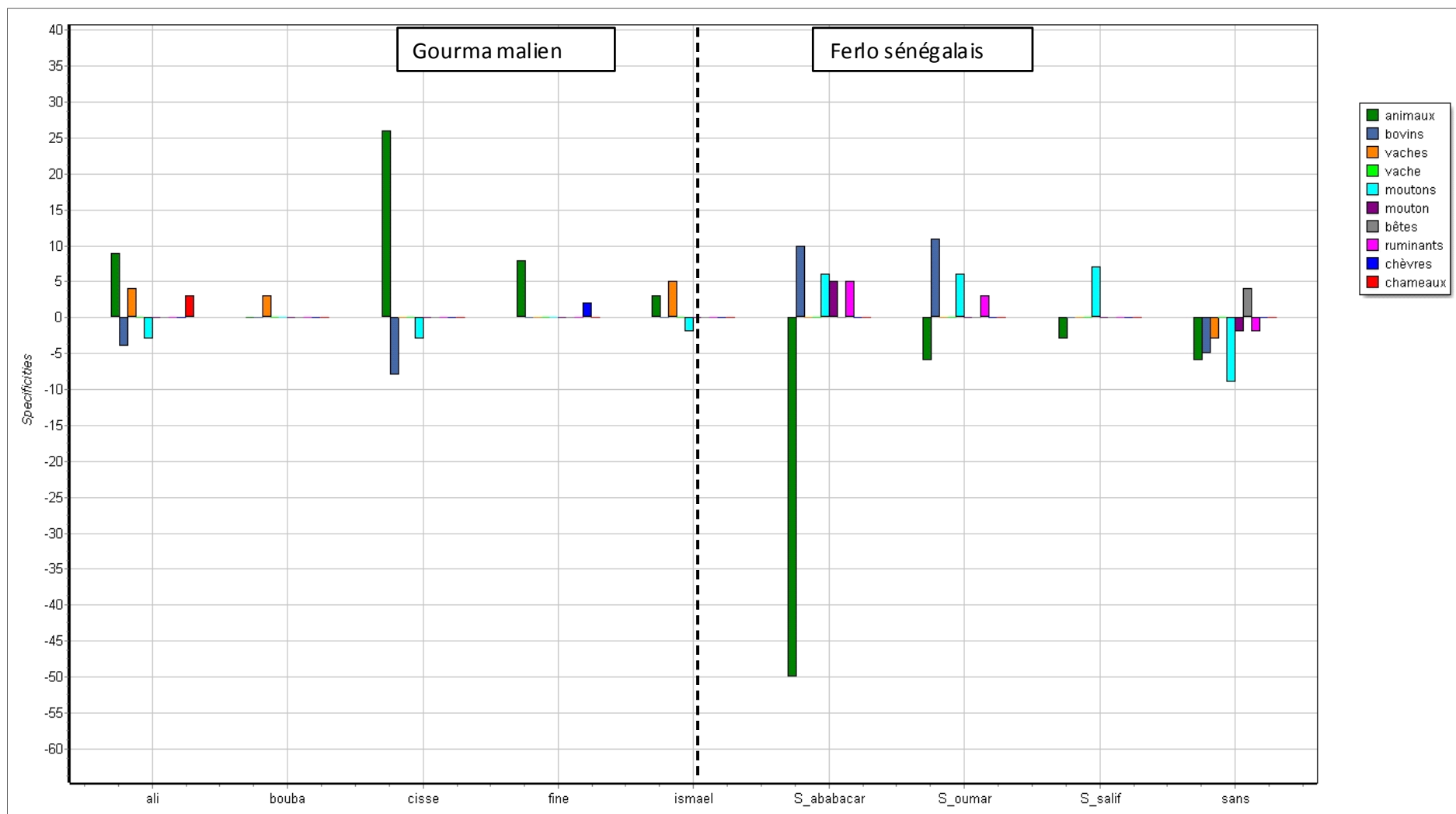
Figure n°10. 14: Spécificités lexicales de la forme « Animaux » par traducteur
