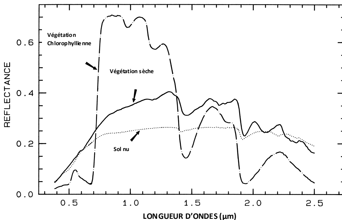
Figure n°4. 1: Signatures spectrales de la végétation et du sol nu (d'après : http://speclab.cr.usgs.gov/ )
