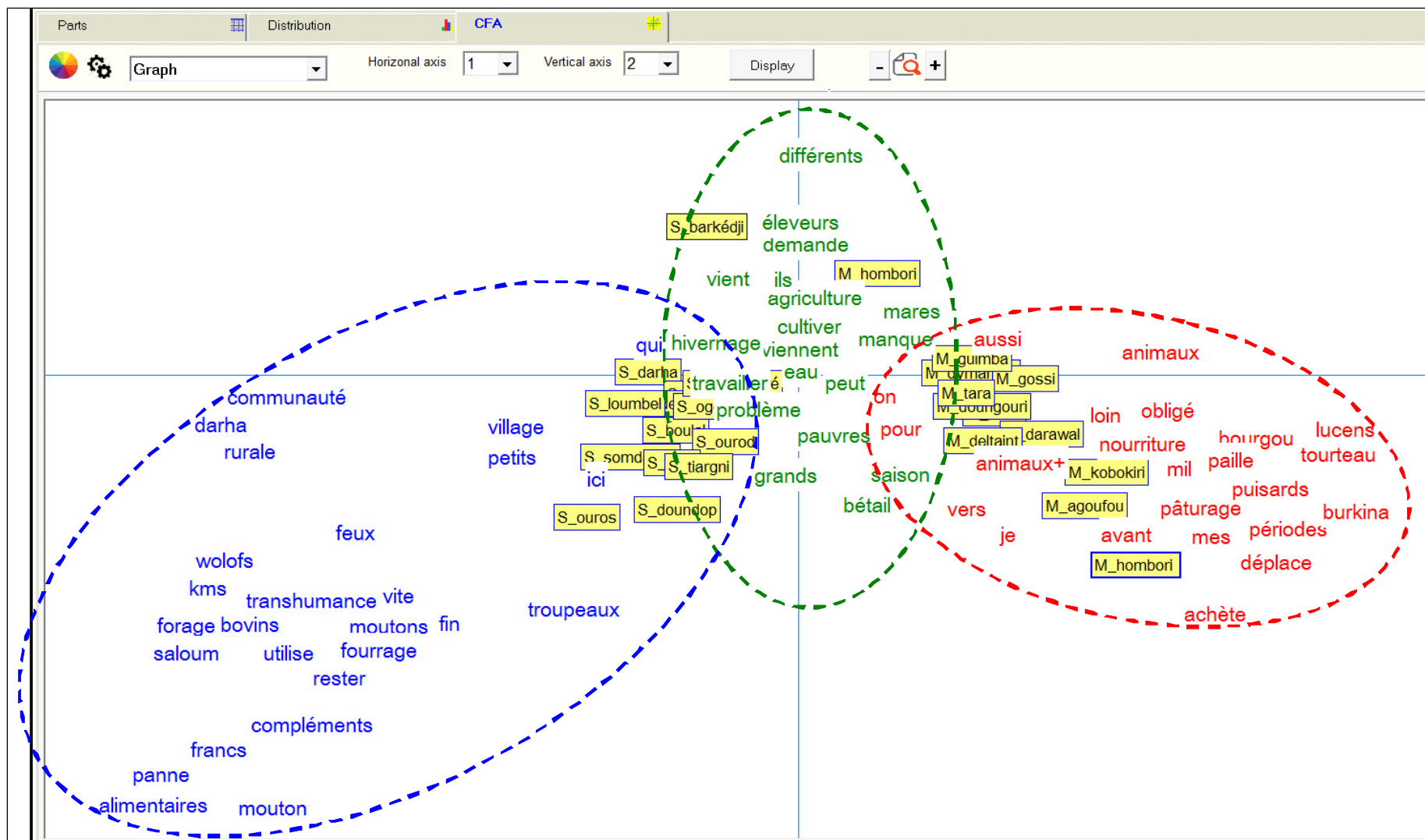
Figure n°10. 21: AFC sur les discours du Ferlo et du Gourma par localité
