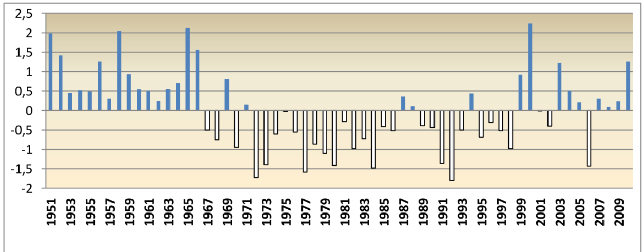
Figure n°6. 25: Évolution de l'indice standardisé des précipitations entre 1951 et 2010 à Matam (Ferlo) (Fall, 2014)
