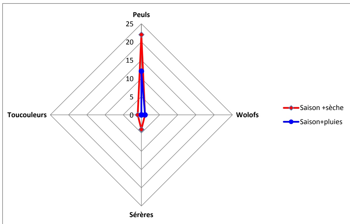
Figure n°10. 8: Perception de la vulnérabilité d'origine climatique en fonction des groupes ethniques : structure du champ lexical autour des saisons
