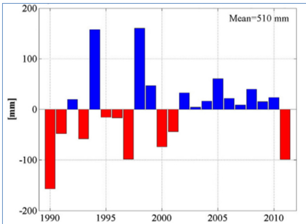
Figure n°6. 28: Évolution des précipitations entre 1990 et 2010 dans le degré carré de Niamey, (Source : Dardel, 2014)
