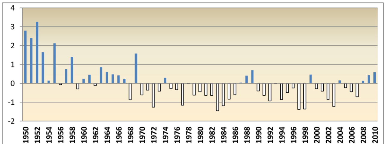
Figure n°6. 26: Évolution de l'indice standardisé des précipitations entre 1950 et 2010 à Louga (Ferlo) (Fall, 2014)
