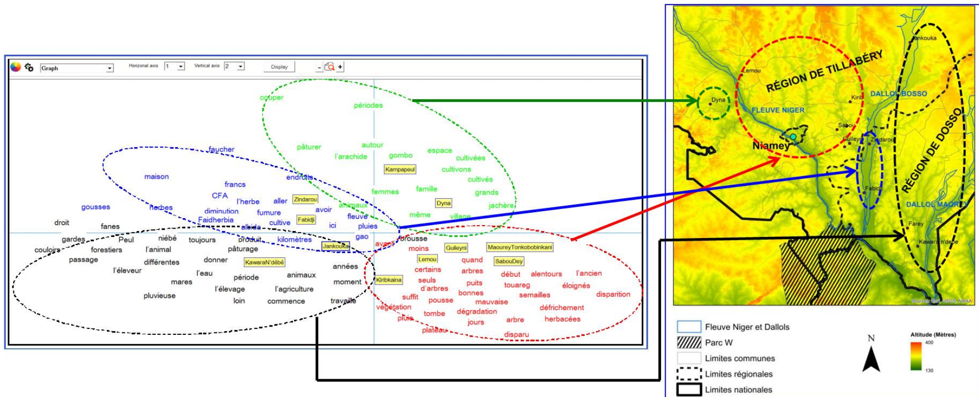
Figure n°9. 3: AFC du discours par localité (Fakara)
