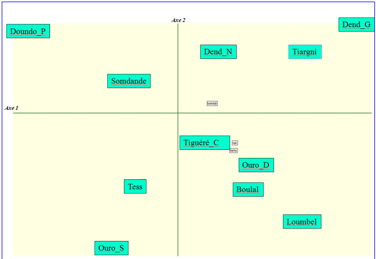
Figure n°8. 8: Analyse factorielle des correspondances sur la partition en « Localités » à partir d'entretiens réalisés dans le Ferlo
