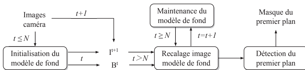
Fig. 2.3.: Processus de la soustraction de fond pour une caméra PTZ. N est le nombre d'images utilisées pour initialiser le modèle de fond B^t . I^t est l'image au temps t .
