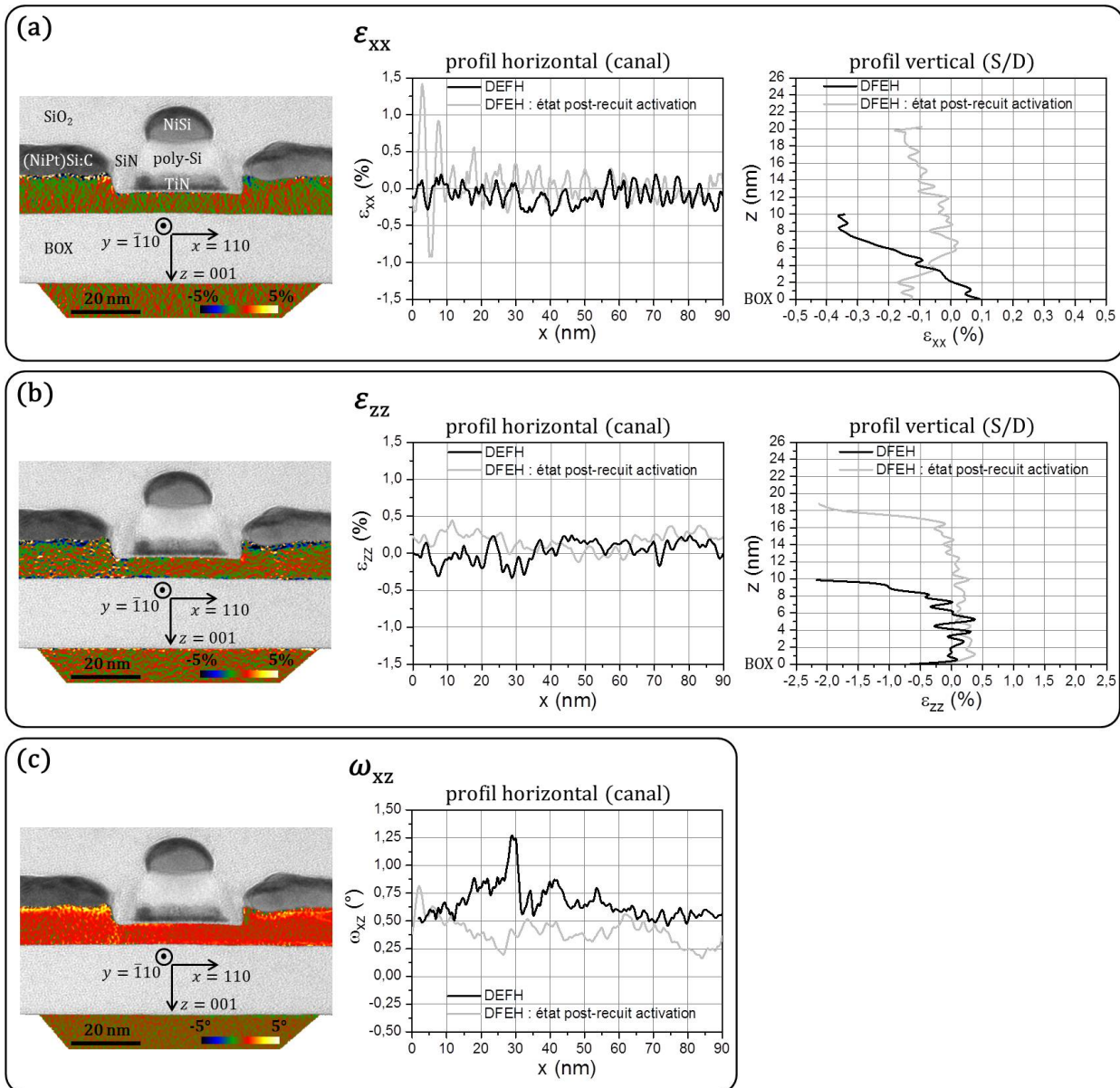
FIGURE 4.13 – Cartographies DFEH de (a) \epsilon_{xx} , (b) \epsilon_{zz} et (c) \omega_{xz} de l'échantillon n-MOS "post-siliciuration", montées avec une image en champ clair pour repérage. Les profils sont extraits dans le canal le long du film mince Si et à travers l'épaisseur des S/D Si:C. Les profils de l'échantillon "post-recuit diffusion" sont superposés pour visualiser l'évolution des déformations.
