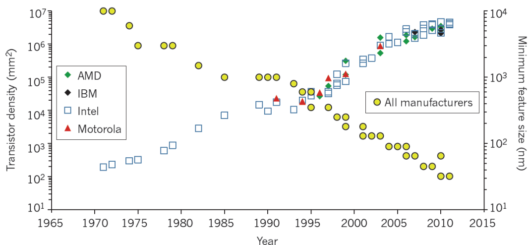
FIGURE 1.3 – Graphique représentant l'évolution de la longueur de grille et de la densité de MOSFETs sur un circuit intégré en fonction des années, illustrant la loi de Moore [Fera11].
