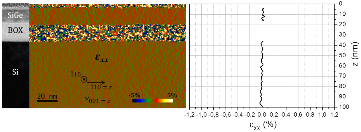
FIGURE 2.5 – Cartographie des déformations \epsilon_{xx} obtenue par DFEH dans la structure SGOI, après la RTO, avec l’image champ clair (BF pour Bright Field) sur la gauche pour repérage. Sur la droite est tracé le profil de déformation vertical, intégré sur une largeur de 25 nm.
