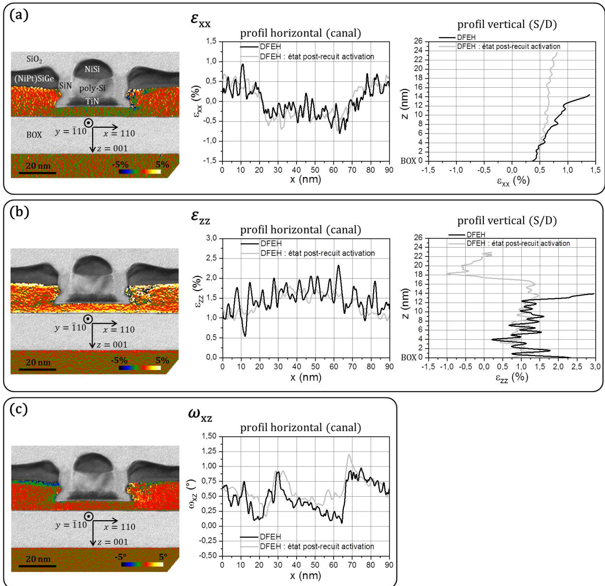
FIGURE 4.14 – Cartographies DFEH de (a) \epsilon_{xx} , (b) \epsilon_{zz} et (c) \omega_{xz} de l'échantillon p-MOS "post-siliciuration", montées avec une image en champ clair pour repérage. Les profils sont extraits dans le canal le long du film mince SiGe et à travers l'épaisseur des S/D SiGe. Les profils de l'échantillon "post-recuit diffusion" sont superposés pour visualiser l'évolution des déformations.
