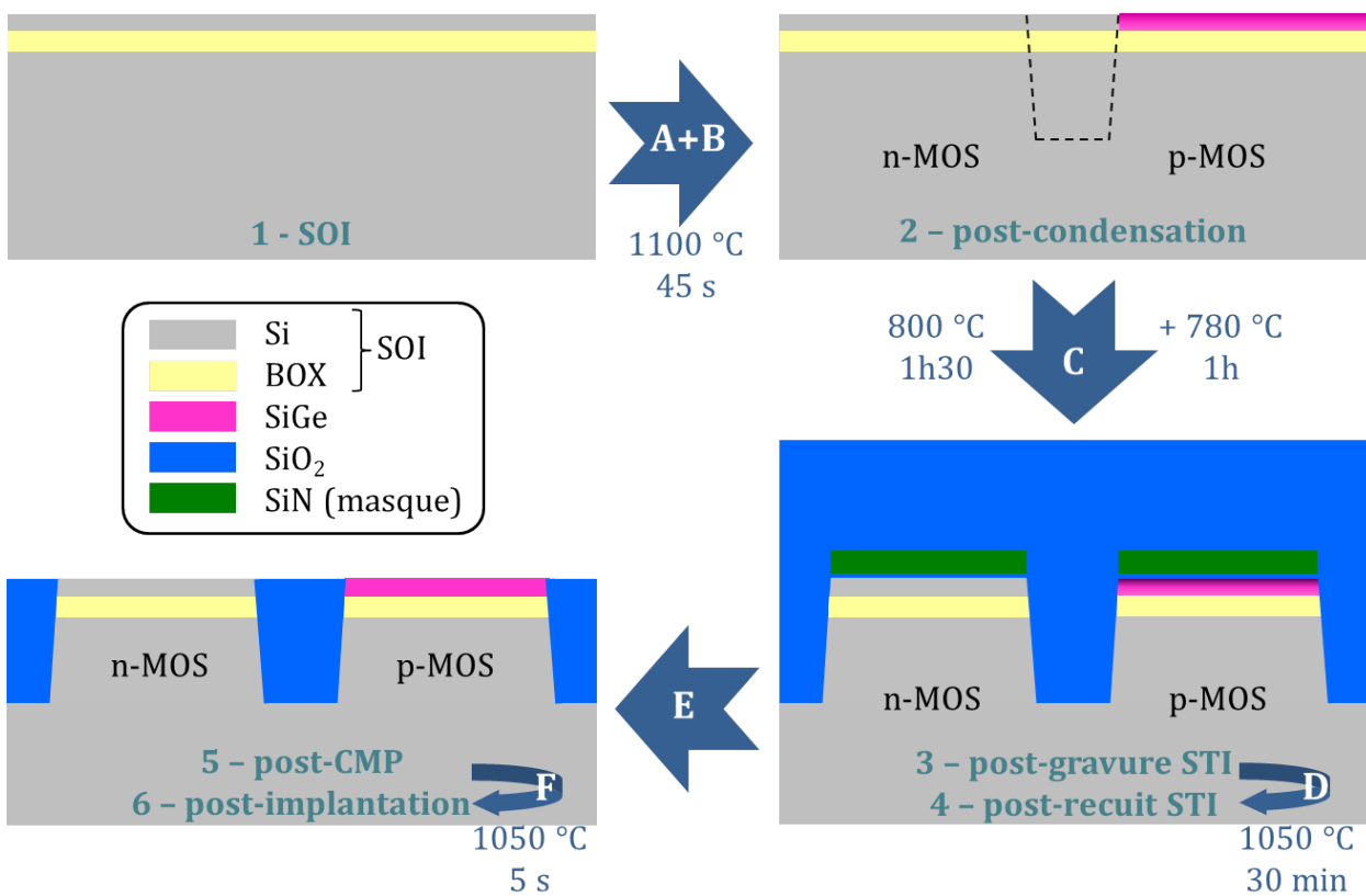
FIGURE 3.1 – Représentation schématique des wafers 1, 2, 3, 4, 5 et 6 prélevés au cours des étapes A, B, C, D, E et F du procédé de fabrication du substrat co-intégré (voir figure 2.3), et description de leur bilan thermique.
