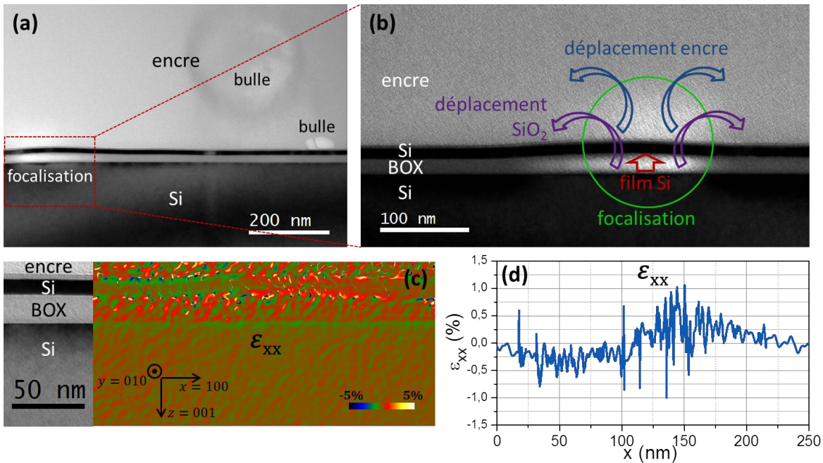
FIGURE 1.35 – Image en champ clair (a) d'un SOI protégé par un dépôt de 3,5 nm de SiO 2 , préparé avec un dépôt d'encre, et (b) montrant l'influence de la focalisation de la sonde électronique lors de son observation. (c) Cartographie des déformations dans le plan \epsilon_{xx} , réalisée au Tecnai, issue de la structure déformée et (d) tracé du profil de déformation extrait le long du film mince Si.
