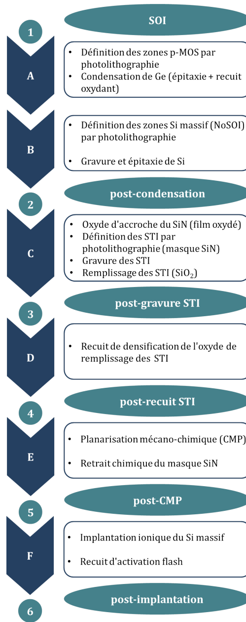
FIGURE 2.3 – Description des étapes (A, B, C, D, E et F) du procédé de fabrication de substrats co-intégrés pour les MOSFETs FDSOI, ainsi que des wafers prélevés (1, 2, 3, 4, 5 et 6) et étudiés dans cette thèse.
