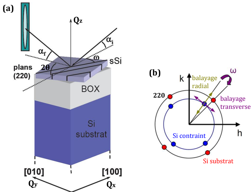
FIGURE 1.12 – (a) Schéma représentant la géométrie d'une mesure GIXRD sur un échantillon sSOI ayant une orientation de surface [001]. (b) Représentation de la mesure sur les plans \{220\} dans l'espace réciproque. Figures adaptées de [Baudo09].
