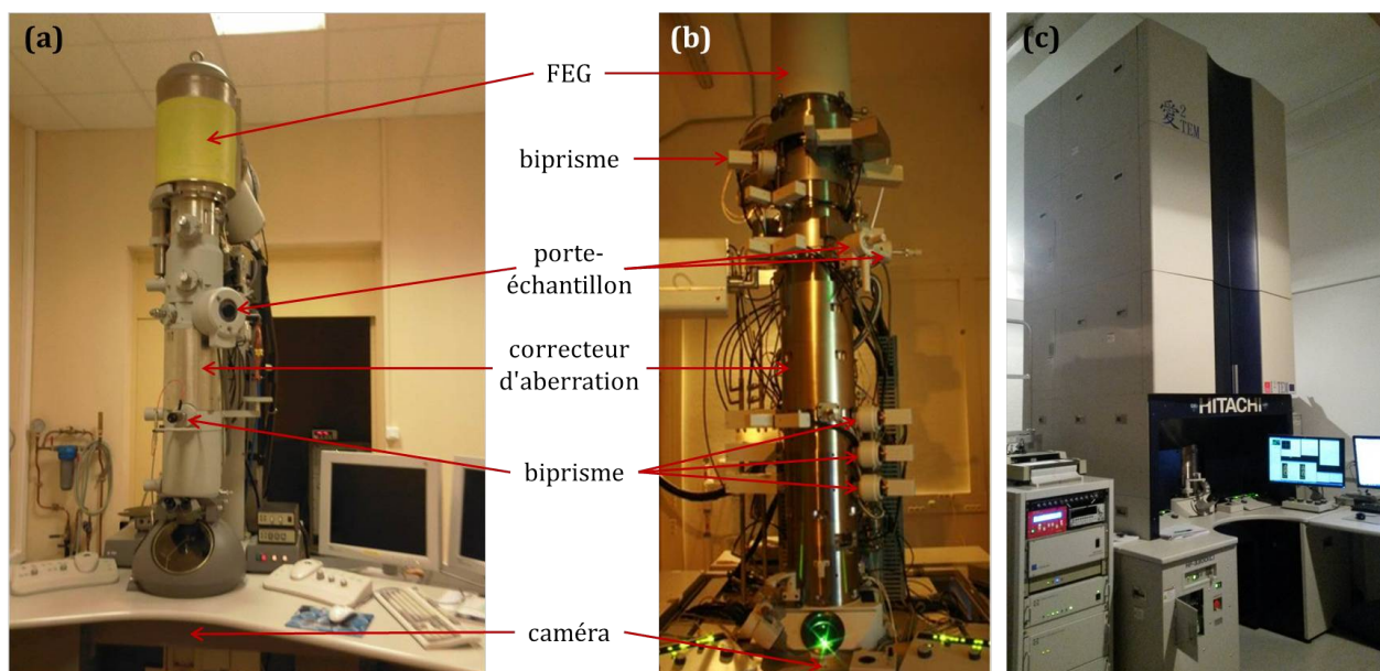
FIGURE 1.22 – (a) Photos du Tecnai, (b) de la colonne de l'I 2 TEM et (c) d'une vue d'ensemble de l'I 2 TEM ; comprenant le repérage des éléments importants pour la DFEH.
