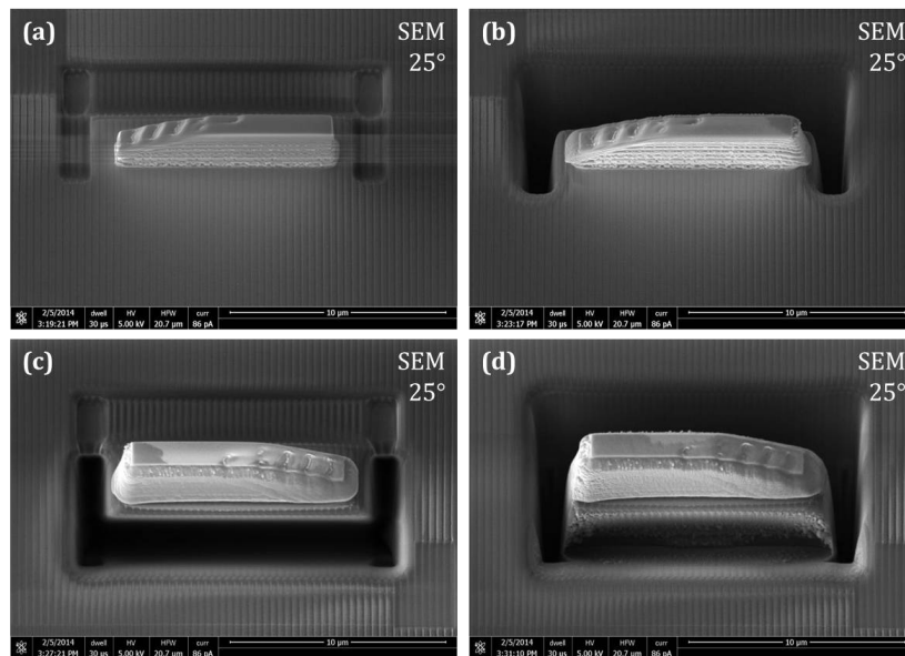
FIGURE 1.29 – Images SEM (angle de 25^\circ entre la normale à la surface et le faisceau imageur) des étapes de découpe de l'échantillon pour la préparation FIB : (a) au cours et (b) après la découpe de la première face puis (c) au cours et (d) après la découpe de la seconde face.
