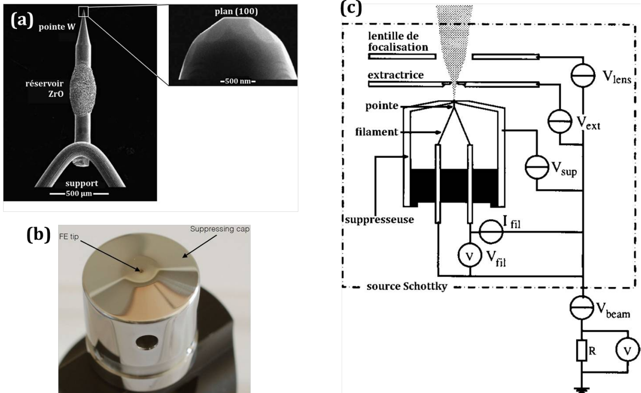
FIGURE B.2 – (a) Image SEM d’une pointe ZrO/W(100) d’une source Schottky, adaptée de [Orlof97]. (b) Photo du bloc contenant la pointe et la supresseuse d’un émetteur York Probe Source (YPS 174) [York15]. (c) Schéma de principe d’une source Schottky, adapté de [Frans98].
