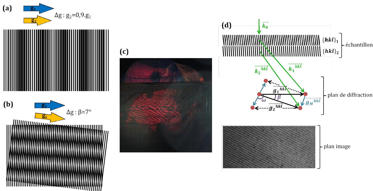
FIGURE 1.14 – Principe de formation des franges de moiré par superposition de deux réseaux sous différentes conditions : (a) dilatation pure de 10 % et (b) rotation pure de 7°. (c) Moirés créés par la superposition de deux toiles en tissus, rétroéclairées par une lumière rouge. (d) Principe de formation de moirés en imagerie TEM, par diffraction multiple, représentant les notations utilisées.
