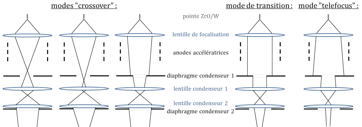
FIGURE B.5 – Schéma de la trajectoire des électrons depuis la source Schottky jusqu'à la seconde lentille condenseur, illustrant les modes de fonctionnement "crossover" et "telescope".
