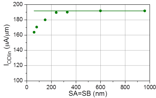
FIGURE 3.17 – Mesure de I_{ODlin} du n-MOSFET en fonction de la distance de la taille de l'active sSOI, tel que SA=SB (la droite représente I_{ODlin} au point de mesure SA=SB=960 nm).
