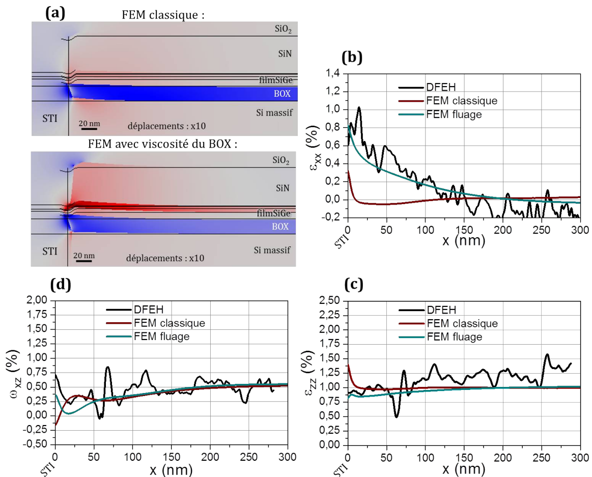
FIGURE 3.9 – (a) Représentation de la structure "post-recuit STI" simulée par éléments finis ; pour une simulation classique et avec un fluage du \text{SiO}_2 . Les déplacements sont amplifiés d'un facteur 10. Tracés des profils (b) \varepsilon_{xx} , (c) \varepsilon_{zz} et (d) \omega_{xz} dans le film SiGe, mesurés par DFEH et simulés par FEM (classiquement et en tenant compte d'un fluage du \text{SiO}_2 ).
