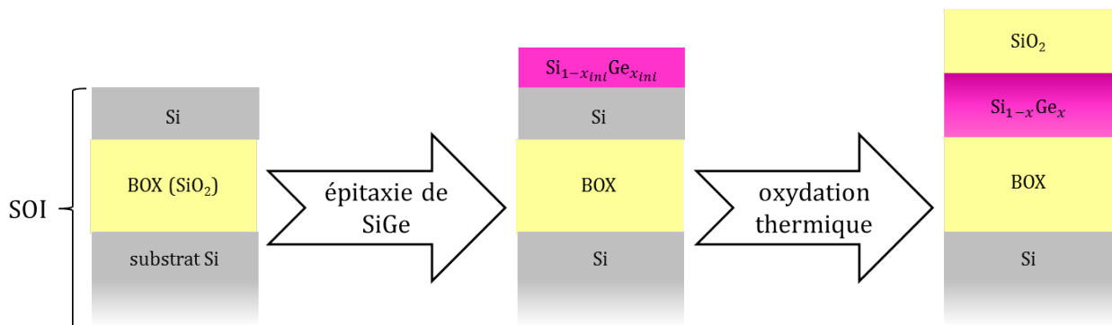
FIGURE 2.2 – Schéma de principe des deux étapes de la condensation de Ge : une épitaxie de \text{Si}_{1-x_{ini}}\text{Ge}_{x_{ini}} sur SOI, suivie d'une oxydation du dessus de la structure.
