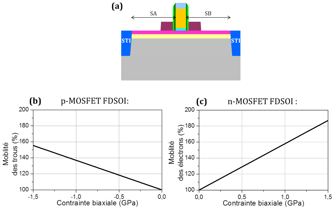
FIGURE 3.15 – (a) Schéma représentant le placement du MOSFET sur l’active en fonction des paramètres géométriques SA et SB. (b) Influence de la compression biaxiale d’un canal FDSOI Si 0,8 Ge 0,2 <110> sur la mobilité des trous, dans l’approximation du modèle piézo-résistif. (c) Influence de la tension biaxiale d’un canal FDSOI Si <110> sur la mobilité des électrons, dans l’approximation du modèle piézo-résistif.
