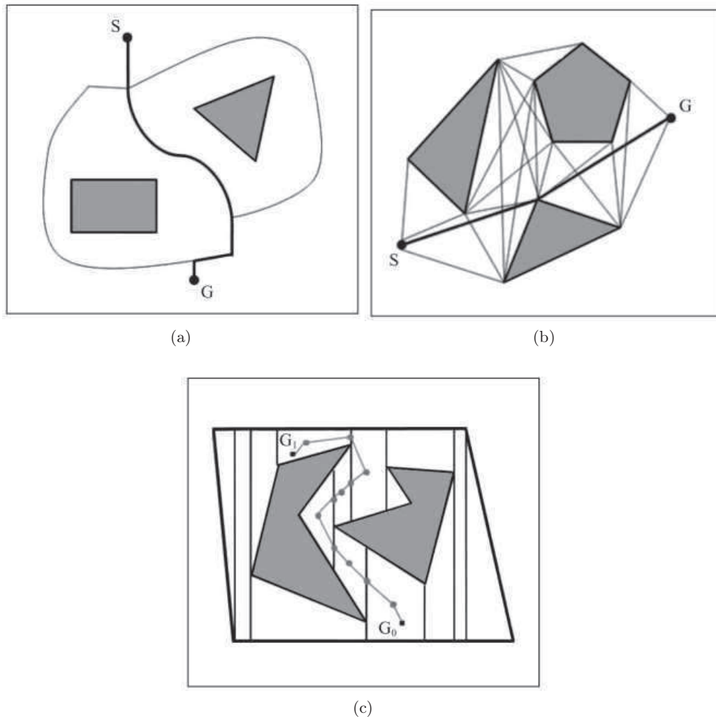
FIGURE 1.5 – Les différents graphes pour la planification de trajectoire extraits de [Tang et al., 2012] (a) Graphe de Vononoï, (b) Graphe de visibilité et (c) Décomposition cellulaire.
