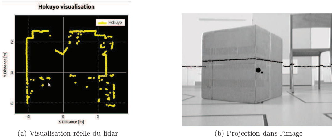
FIGURE 2.8 – La projection des données d'un capteur lidar dans une image perspective.
