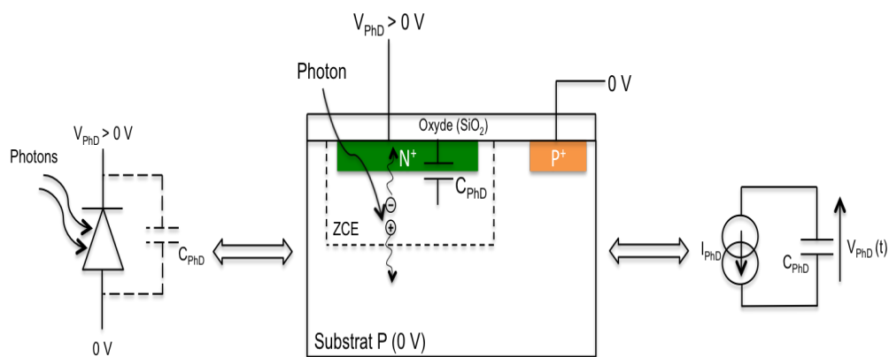
FIGURE 2.13 – Fonctionnement de la photodiode sous éclairage.
