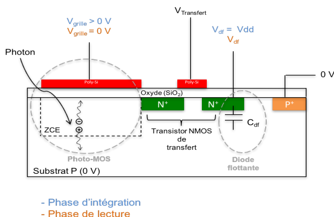
FIGURE 2.14 – Fonctionnement du photo-MOS sous éclaircissement.
