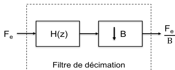
FIGURE 3.7 – Vue conceptuelle d'un filtre de décimation.
