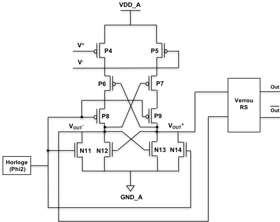
FIGURE 3.25 – Comparateur utilisé.
