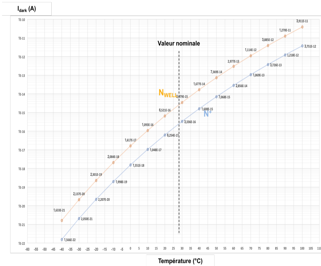
FIGURE 3.14 – Variation du courant d'obscurité en fonction de la température pour les deux architectures de diode et pour une taille de diode de 28,5 \text{ } \mu\text{m} \times 28,5 \text{ } \mu\text{m} .
