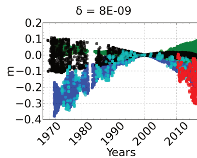
C_{3,0}, Moon
