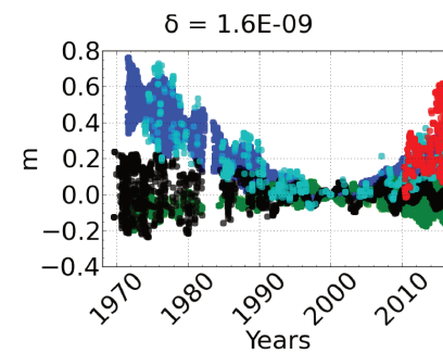
C_{3,2}, Moon
