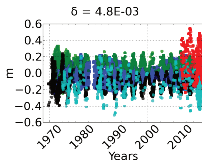
\tau_{Moon}
