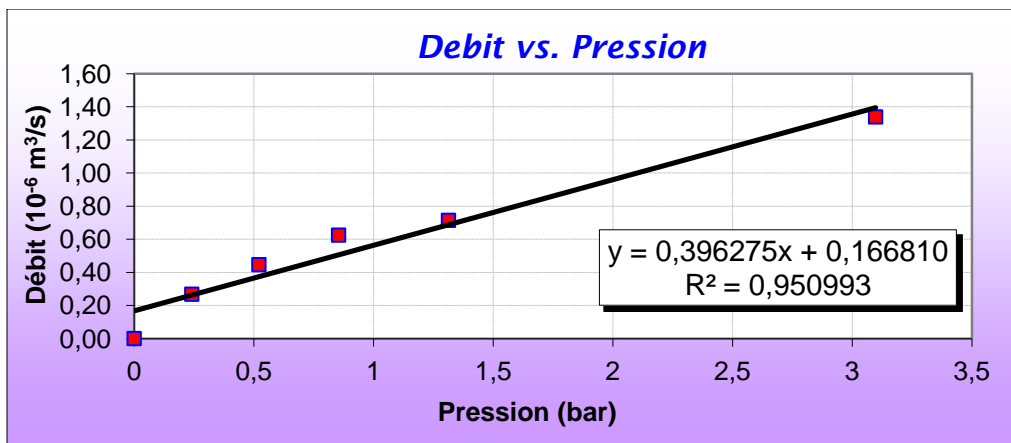
Illustration 11 Mesure de K_z pour tissu H
