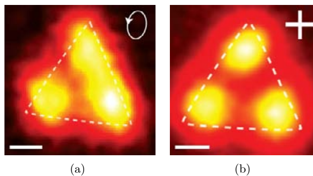
FIGURE IV.3 – (a) Image TPL expérimentale d'un prisme isolé balayé avec un faisceau polarisé de façon quasi-circulaire. (b) Carte TPL d'un autre prisme obtenue en sommant les signaux calculés pour deux polarisations linéaires perpendiculaires matérialisées par la croix blanche. Barres d'échelle 200 nm. Figure adaptée de la référence [170].
