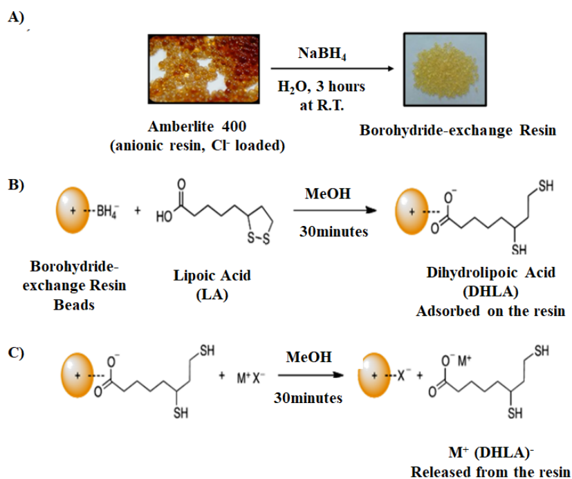
Figure 2 Préparation de la résine (a). Réduction de l'acide lipoïque avec une résine modifiée au borohydrure (b) et extraction de l'acide dihydrolipoïque à partir des billes de résine avec un sel MX (c).
