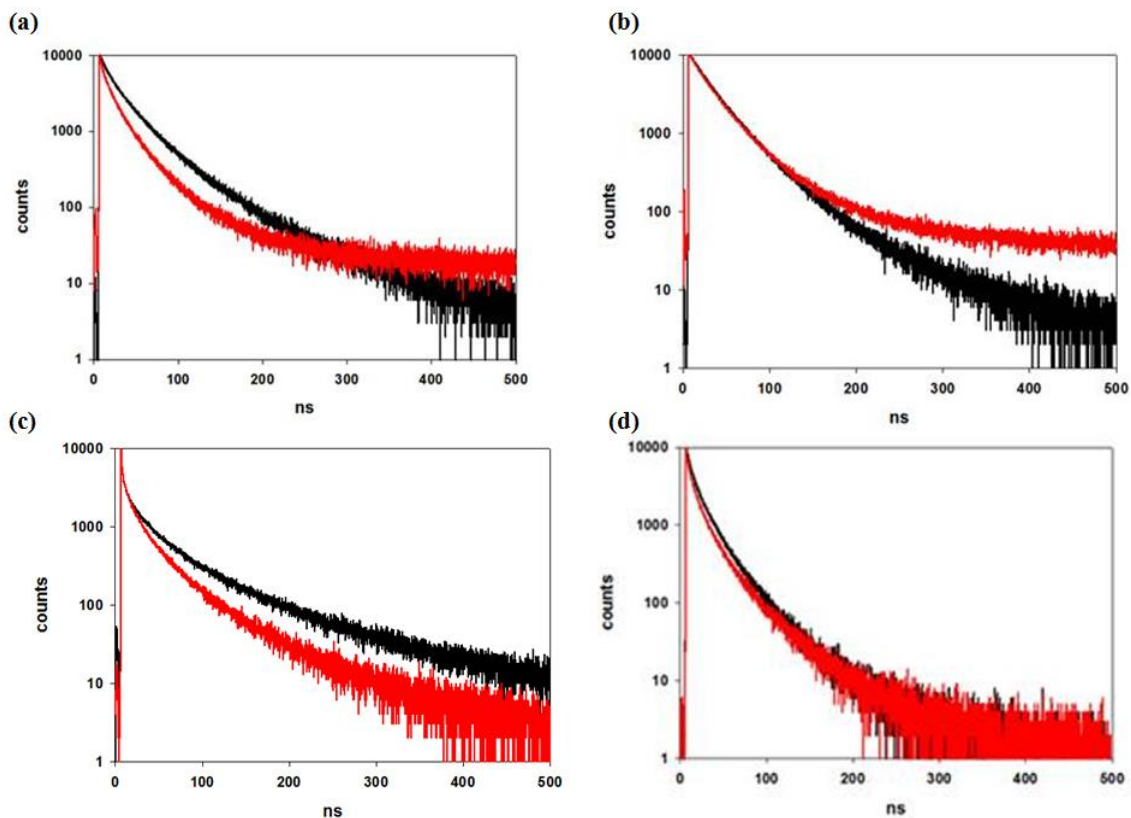
Figure 9 Durée de vie de la luminescence des CdSe QDs 2 (a), 3 (b), 1 (c) 4 (d) fonctionnalisées avec des échantillons 1-PCA (lignes rouges) et non fonctionnalisés (lignes noires) enregistrés dans l'heptane dégazé en excitant sélectivement les QDs à 405 nm et en regardant leurs émissions. L'échelle de temps est de 500 ns tandis que les 10000 comptes détectés sont rapportés en échelle logarithmique.
