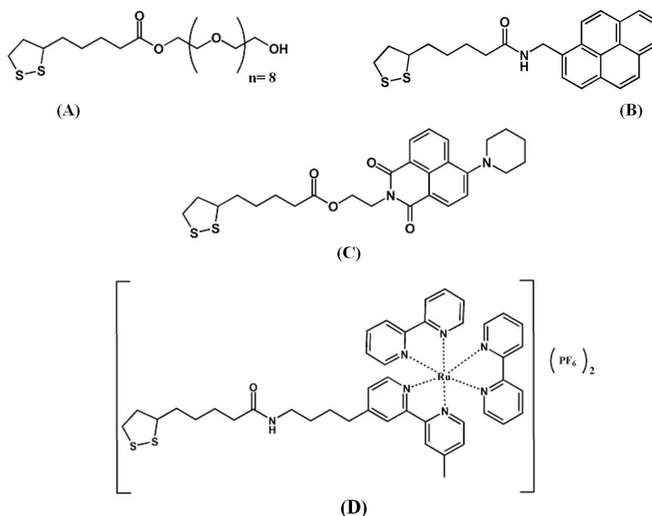
Figure 5.10 Molecular structure of (A) LA-PEG 400 ; (B) LA-PYR; (C) LA-NAP; (D) LA-Ru.
