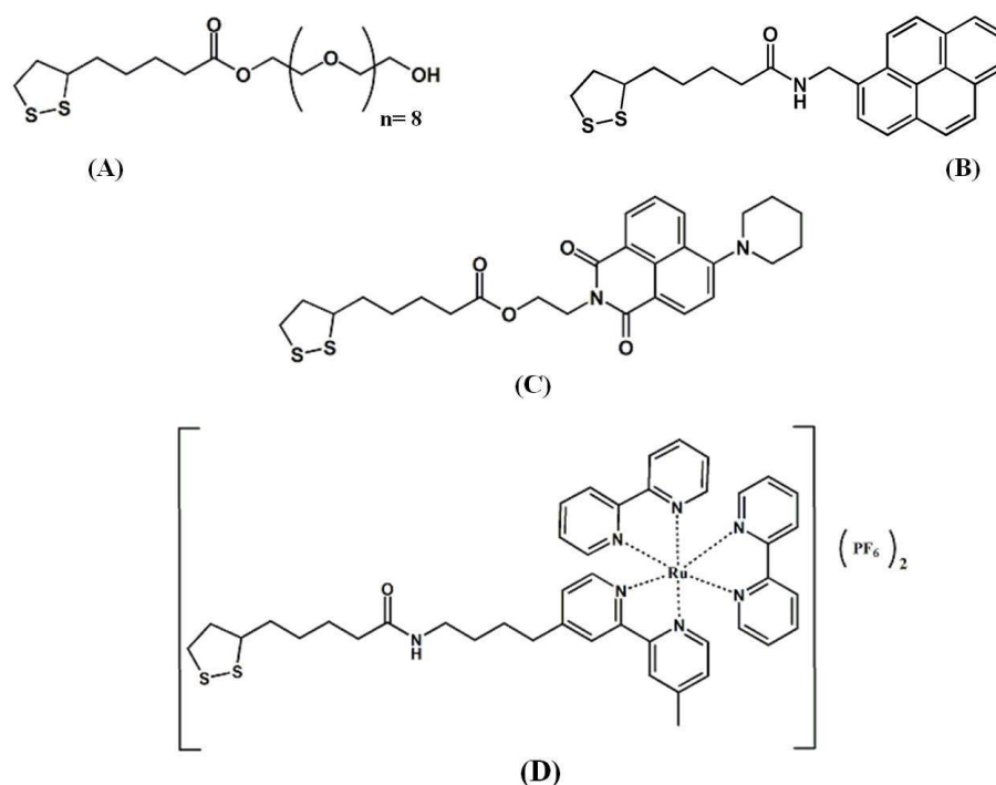
Figure 6 Structure moléculaire de (A) LA-PEG 400 ; (B) LA-PYR; (C) LA-NAP et (D) LA-Ru.
