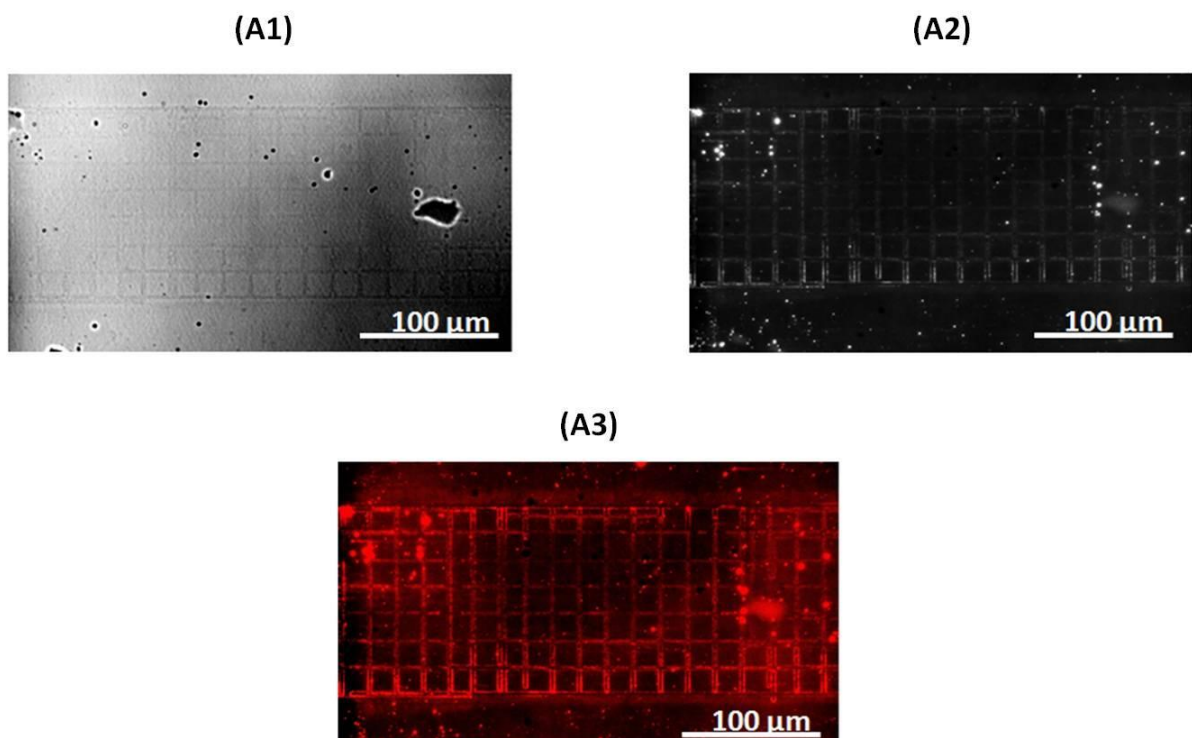
Figure 11 Les images de transmission (A1) et de fluorescence (A2) du modèle A. (A3) est le recouvrement entre (A1) et (A2).
