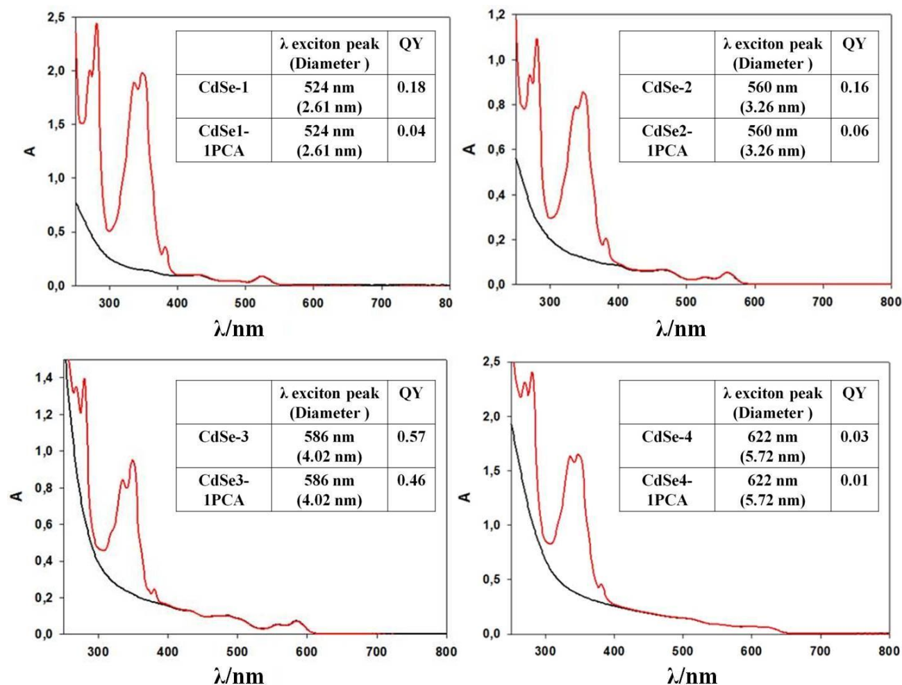
Figure 8 Spectre d'absorption de CdSe QDs avant (lignes noires) et après (lignes rouges) fonctionnalisation avec 1-PCA, enregistré avec la même valeur d'absorbance au pic d'exciton. Dans les inserts, les propriétés photophysiques et dimensionnelles de chaque échantillon, avec et sans 1-PCA, sont rapportées.
