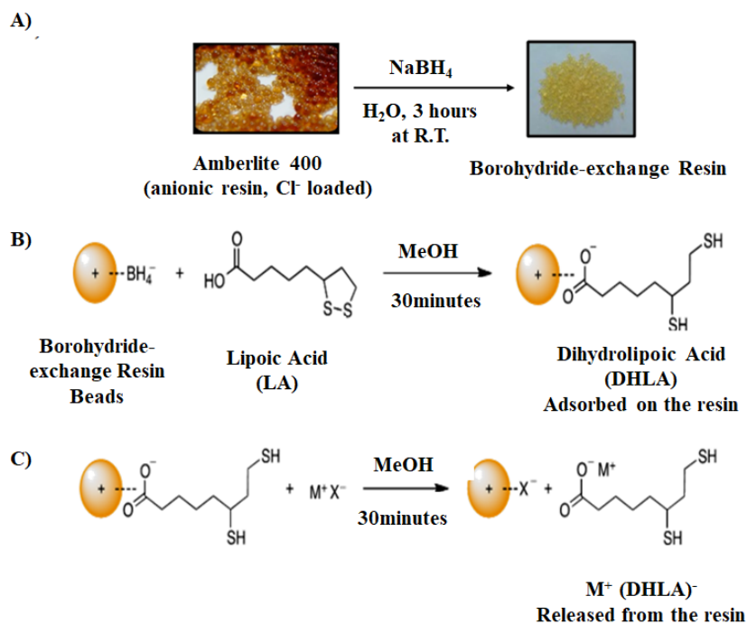
Figure 2 Préparation de la résine (a). Réduction de l'acide lipoiq̃ue avec une résine modifi e au borohydrure (b) et extraction de l'acide dihydrolipo ique   partir des billes de r sine avec un sel MX (c).
