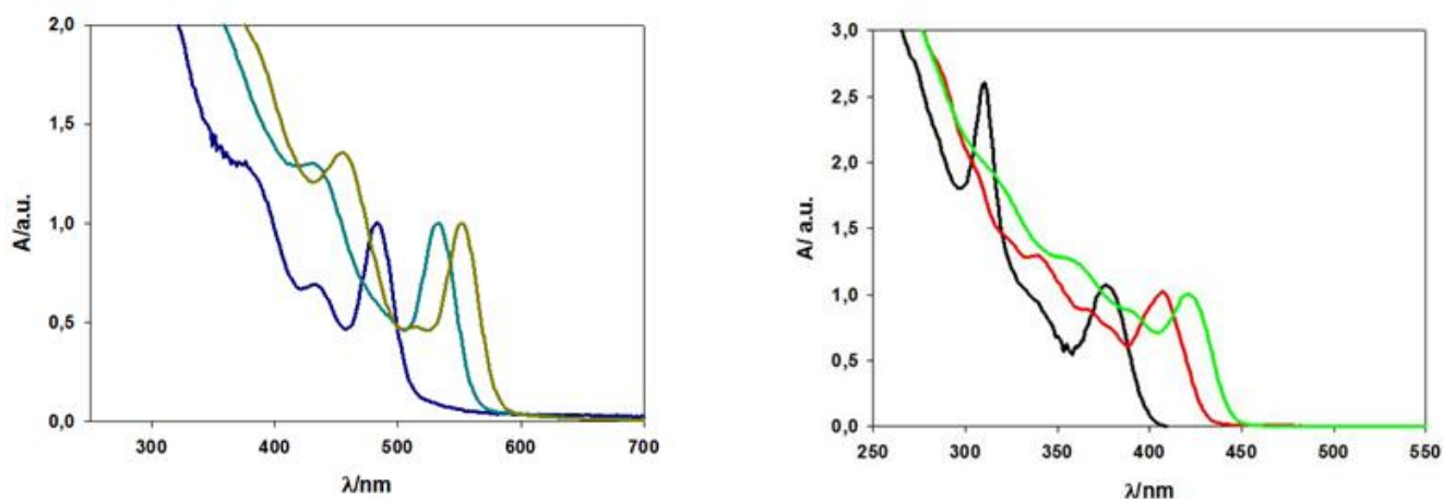
Figure 4 Spectres d'absorption normalisés des échantillons CdSe-1 (ligne bleu foncé), CdSe-2 (ligne cyan foncé) et CdSe-3 (ligne jaune foncé) à gauche et des échantillons CdS-1 (ligne noire), CdS-2 (ligne rouge), CdS-3 (ligne verte) sur la droite. Tous les spectres sont enregistrés dans \text{CHCl}_3 .
