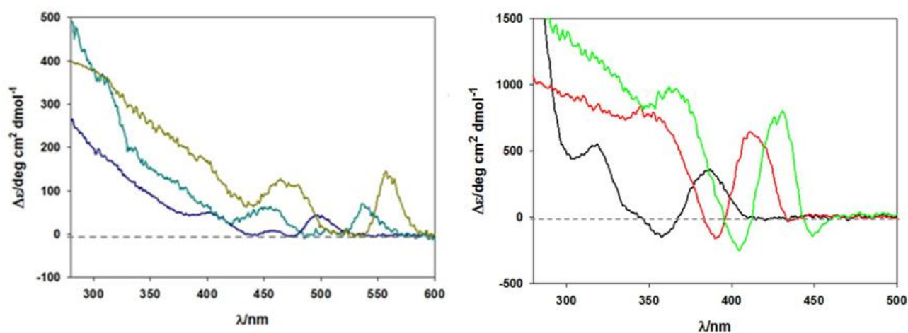
Figure 5 Coefficient d'absorption différentielle. Spectres des échantillons CdSe-1 (ligne bleu foncé), CdSe-2 (ligne cyan foncé) et CdSe-3 (ligne jaune foncé) à gauche et des échantillons CdS-1 (ligne noire), CdS-2 (ligne rouge) et CdS-3 (ligne verte) sur la droite.
