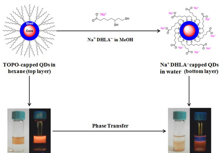
Figure 3 Transfert de phase des QDs hydrophobes dans un solvant polaire par échange de ligands.
