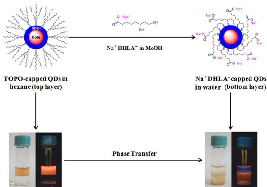
Figure 3 Transfert de phase des QDs hydrophobes dans un solvant polaire par  change de ligands.
