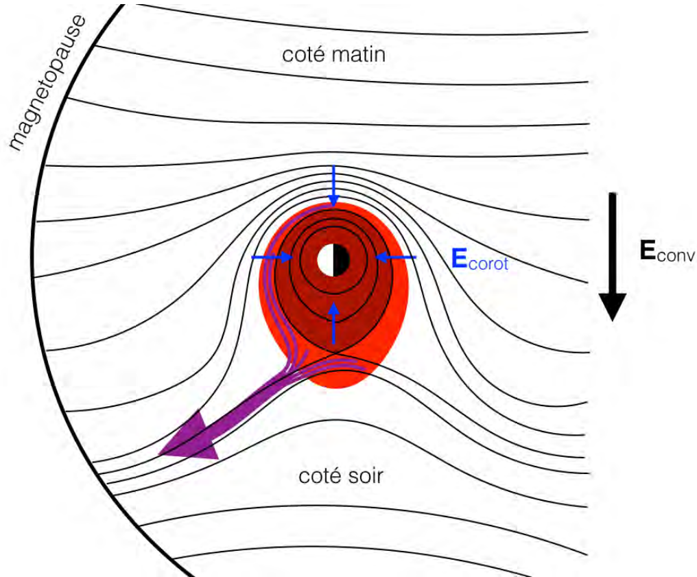
FIGURE 1.20 – Coupe équatoriale de la magnétosphère. Les lignes noires représentent les équipotentielles du champ électrique. La flèche noire (resp. les flèches bleues) représente la direction du champ électrique de convection (resp. de corotation). La zone rouge est la plasmasphère avant perturbation du champ électrique. La zone rouge foncée est la plasmasphère après perturbation. L'augmentation du champ de convection modifie les équipotentielles du champ électrique de telle sorte que certaines populations auparavant piégées dans des équipotentielles fermées se retrouvent sur des équipotentielles ouvertes. Elles vont alors pouvoir dériver vers la magnetopause suivant les nouvelles lignes équipotentielles (flèche violette), créant ainsi une plume plasmasphérique.
