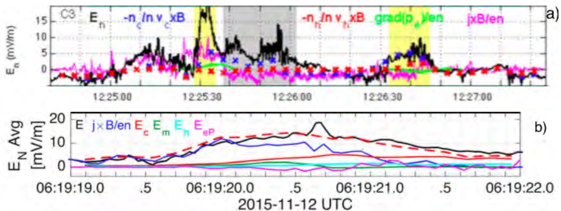
FIGURE 6.5 – Estimations des termes de la loi d'Ohm lors d'une traversée du champ de Hall par Toledo-Redondo et al. (2015) (graphe a) et André et al. (2016) (graphe b). (a) - Données du 8 Avril 2008 par Cluster II (satellites C3 et C4). Les zones de champ de Hall sont indiquées en jaune. La légende associant chaque courbe de couleur à un terme de la loi d'Ohm est donnée dans le graphe. Les données de champ électriques sont estimées comme peu fiables dans la région marquée en gris. (b) - Données du 11 Décembre 2015 par MMS (moyenne sur les quatre satellites). La légende associant chaque courbe de couleur à un terme de la loi d'Ohm est donnée dans le graphe. E_c , E_m et E_h sont les termes -n_s/n \mathbf{v}_s \times \mathbf{B} associés respectivement aux ions froids ( \sim 50 eV dans ce cas), aux ions tièdes (de la magnétogaine, \sim 0,8 - 1 keV) et aux ions chauds ( 7 - 25 keV). E_{eP} représente le terme de divergence de la pression dans la loi d'Ohm. La courbe pointillée rouge montre la somme de ces différents termes.
