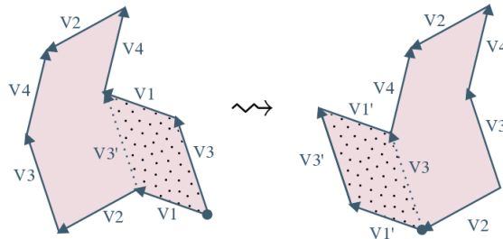
FIGURE 3. Deux surfaces de translation équivalentes.
