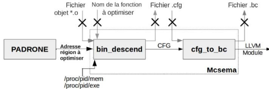
Figure 4: L'intégration de McSema dans Padrone
