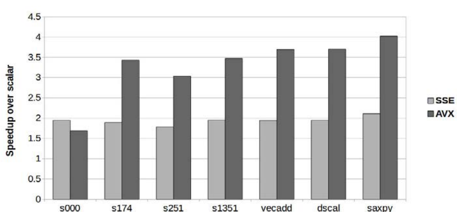
Figure 6: Les résultats de la vectorisation automatique
