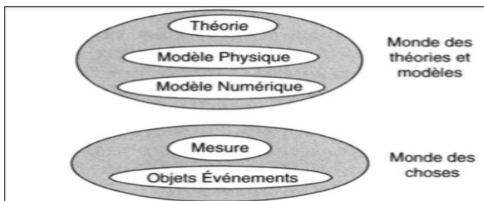
Figure 2. Place des aspects quantitatifs dans la description des deux mondes en relation.
