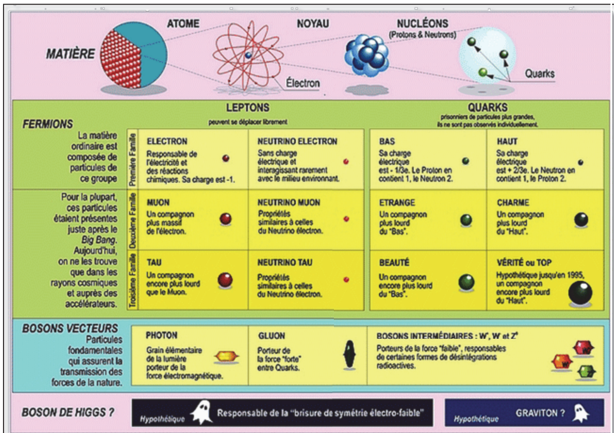
Figure 11. Modèle des particules élémentaires dans le cadre du modèle standard de la physique 81 .
