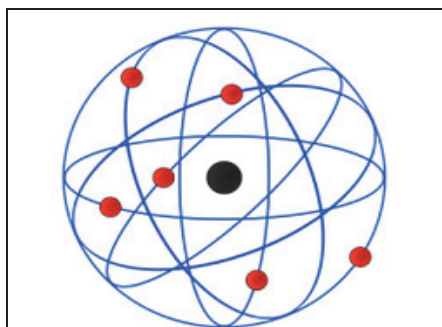
.Figure 7. Représentation lacunaire de la matière modèle planétaire de Rutherford.
