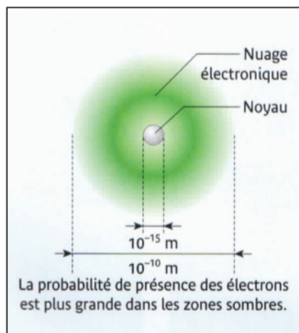
Figure 9. Le modèle quantique de l'atome.
