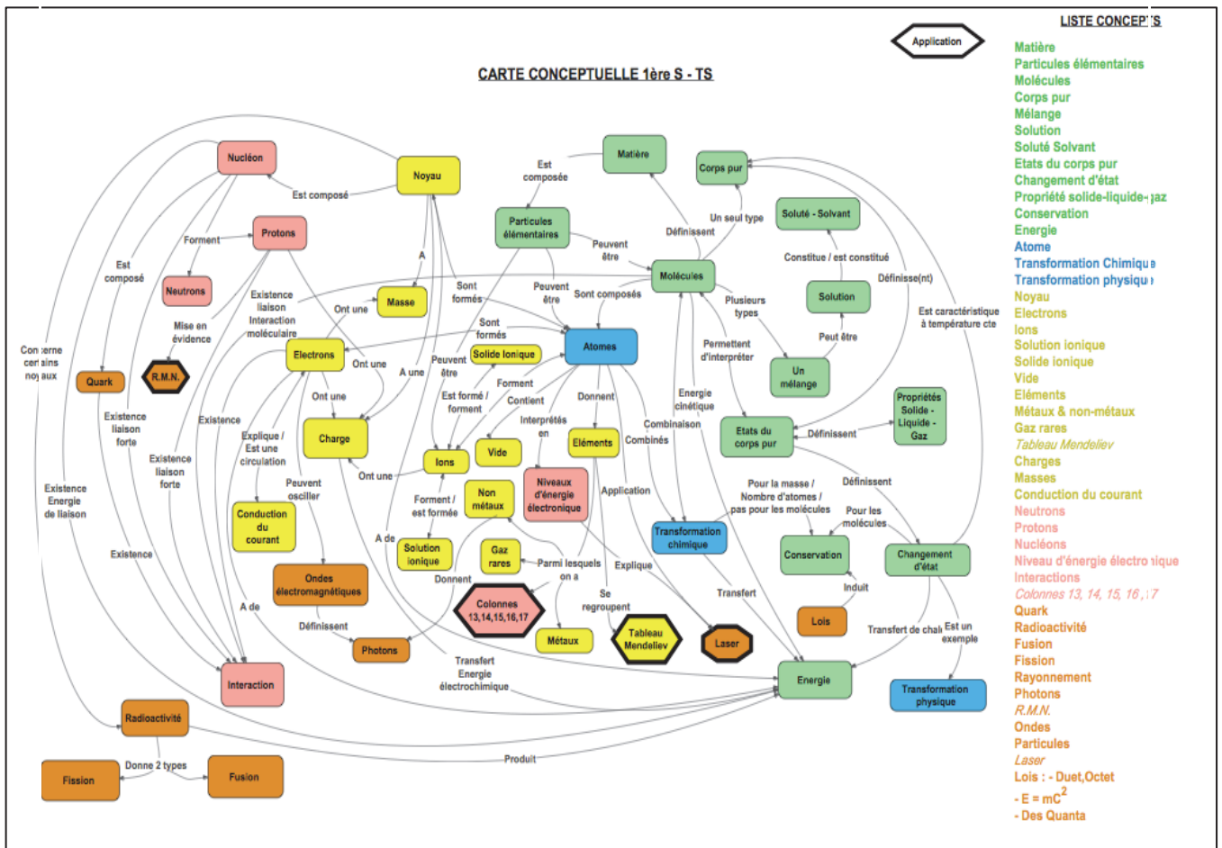
Figure 27. Carte conceptuelle de l'atome pour le lycée en terminale S (Dubosq 2015)
