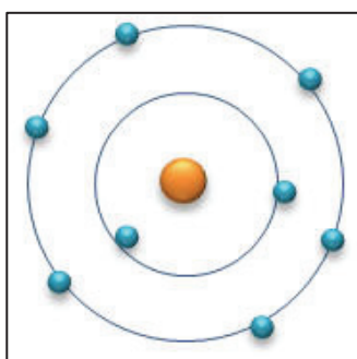
.Figure 8. Représentation du modèle de Bohr pour l'atome d'oxygène.
