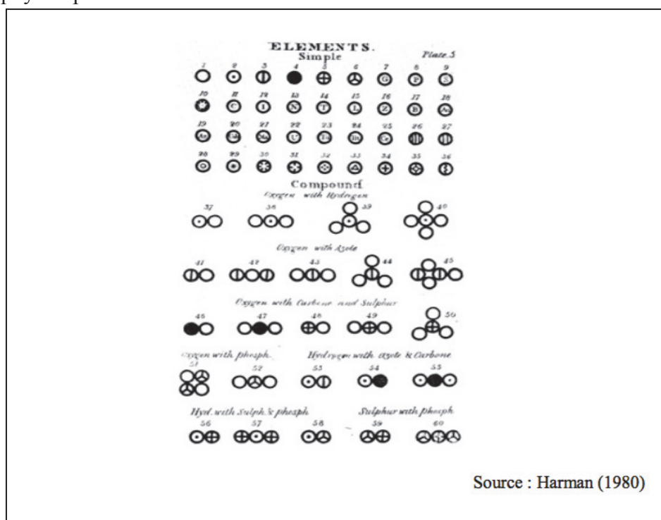
Figure 4. Représentation daltonienne des atomes et des molécules.
