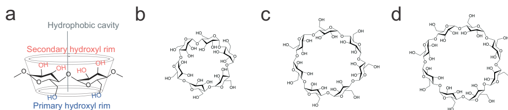
Figure 8.1: Structure chimique des cyclodextrines natives a) Structure 2D de la cyclodextrine montrant l'arrangement des monomères de glucose b) \alpha CD c) \beta CD d) \gamma CD.
